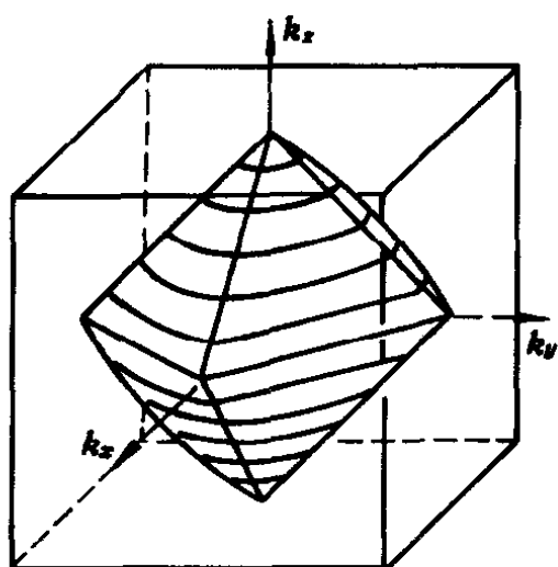
图 4-42 E = E_0 - 2J_1 等能面
