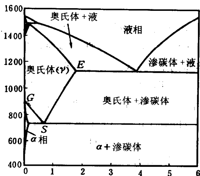
图 13-6 Fe-C 相图
