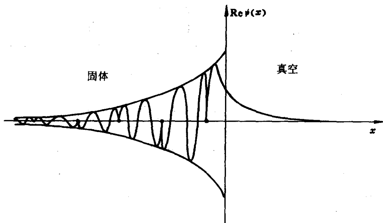
图 4-48 表面态波函数
