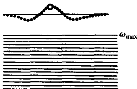
图 3-17 晶格振动的局域模
