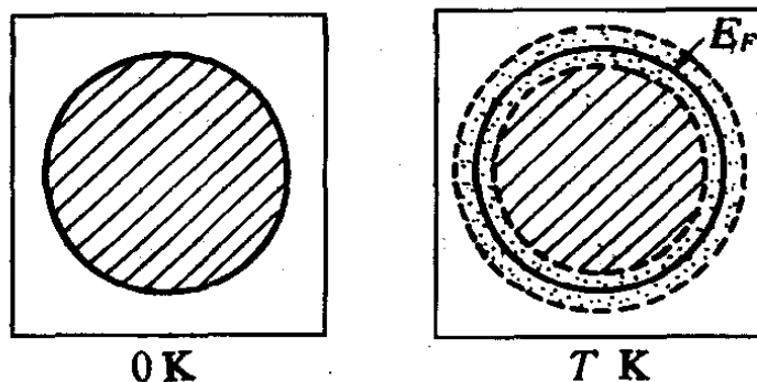
图 6-2 费米面和热激发
