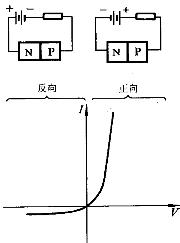
图 7-12 PN 结的单向导电性
