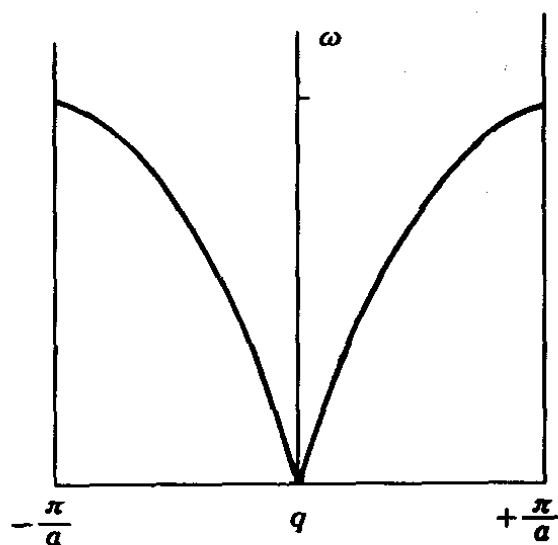
图3-4 一维单原子链的 \omega - q 函数关系
