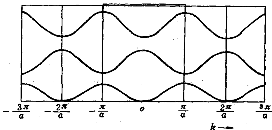
图 4-32 周期布里渊图象
