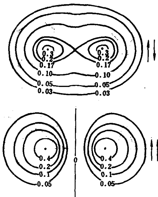
图 2-2 H_2 分子中电子云的等密度线图
