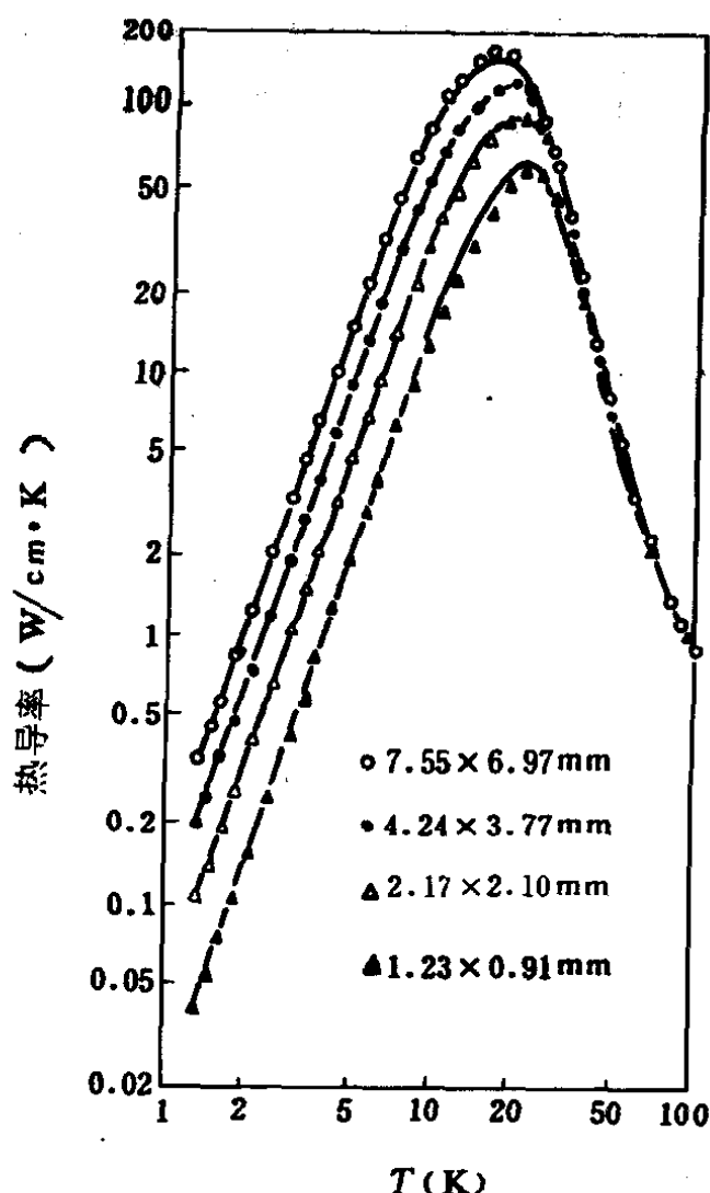
图 3-31 热导与样品尺寸之间的关系
