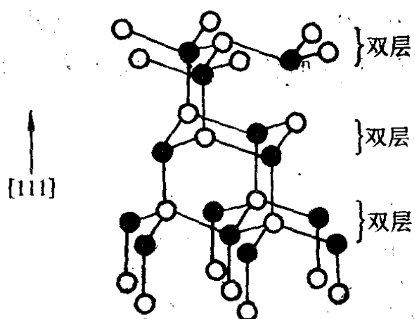
图 1-23 金刚石晶格中的双层密排面
