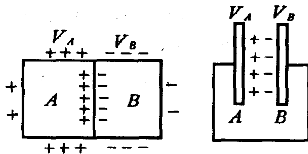
图 6-10 接触电势
