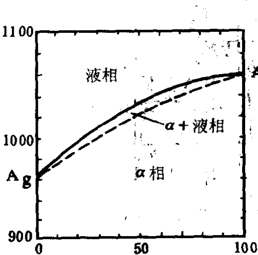
图 13-1 Ag-Au 相图
