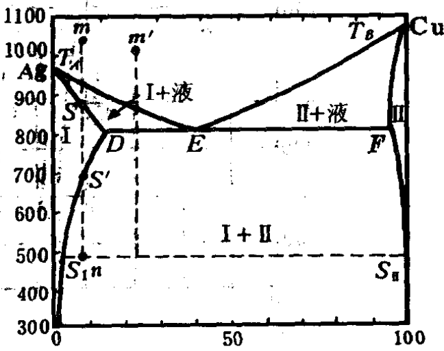
图 13-2 Ag-Cu 相图
