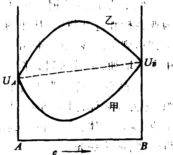
图 13-14 能量函数的两种情况
