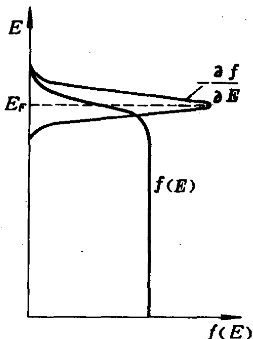
图 6-4 \left(-\frac{\partial f}{\partial E}\right) 的特点
