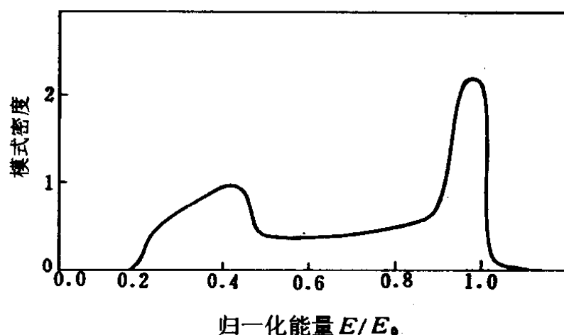
图 3-35 非晶硅的模式密度
