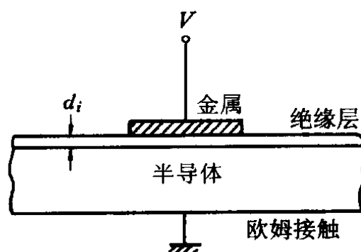
图 7-15 MIS 结构
