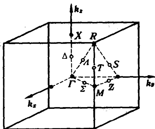
图 4-24 简单立方布里渊区
