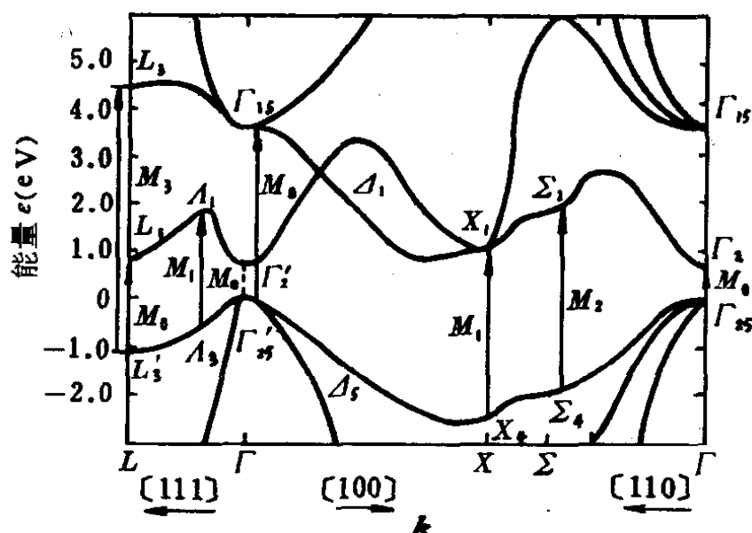
图 9-4 镉的能带结构,图中标出了联合态密度的奇点位置及它们与图 9-3 之间的对应关系
