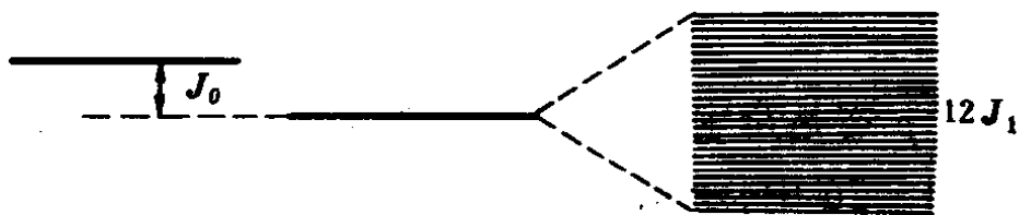
图 4-25 原子能级分裂成能带
