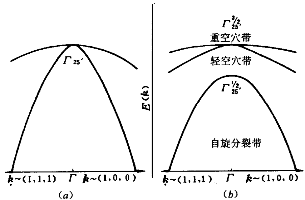
图 7-2 锗、硅价带结构示意图
