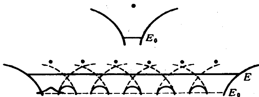
图 4-1 一维周期场
