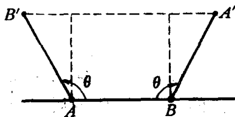
图 1-31 转动变换的示意图
