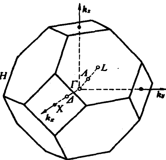
图 4-13 面心立方晶格的简约布里渊区
