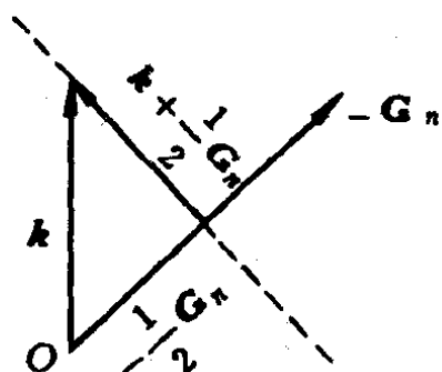
图 4-8 发散条件
