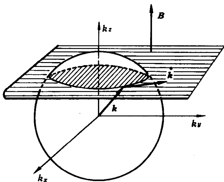
图 5-13 在磁场作用下自由电子在 \mathbf{k} 空间运动的轨迹
