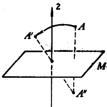
图 1-29 镜面
