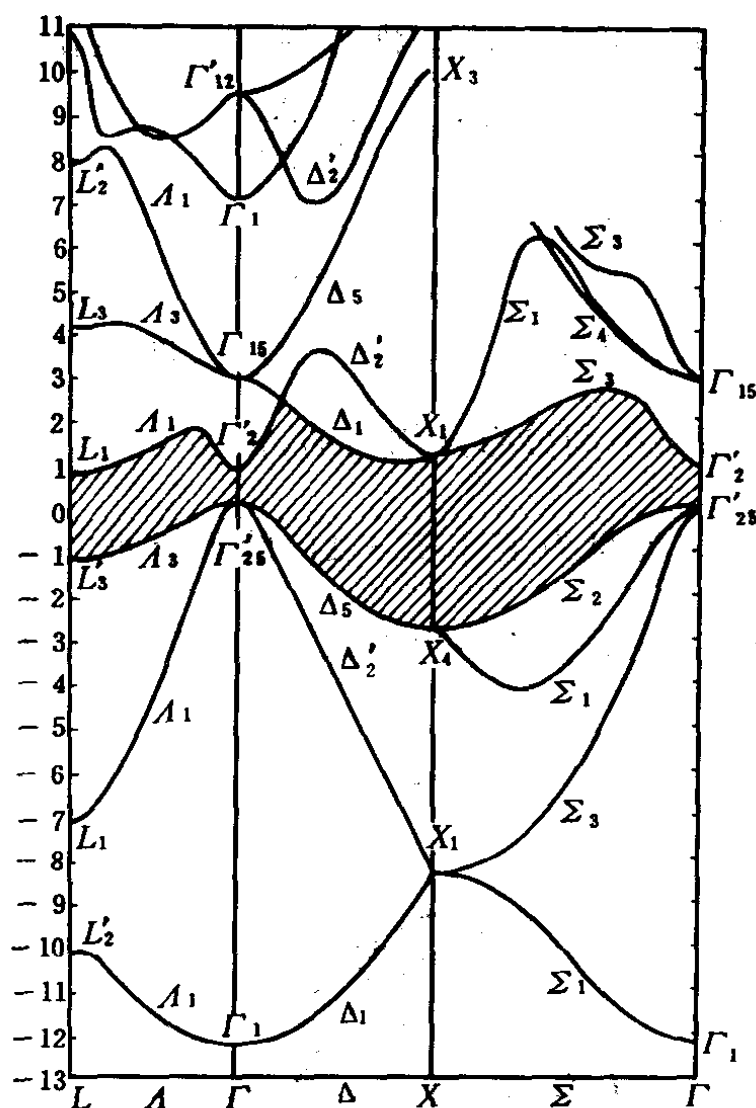
图 4-35 Ge 的能带
