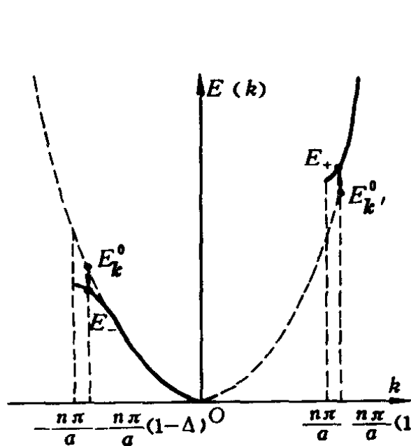
图 4-3 能量的微扰
