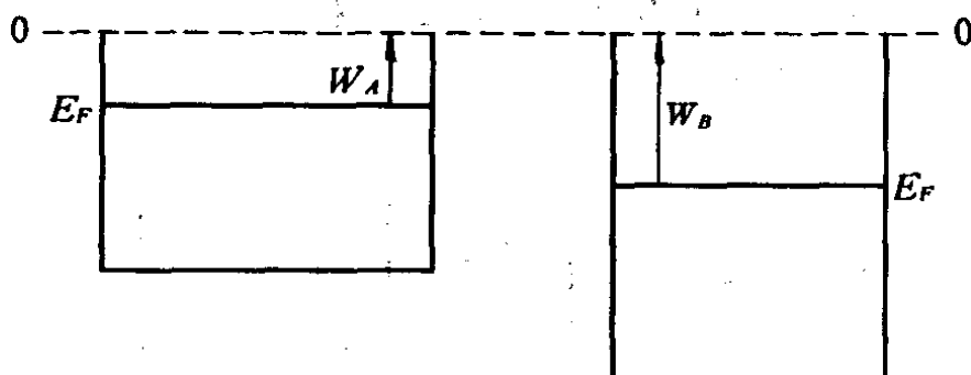
图 6-11 金属的能级图和功函数
