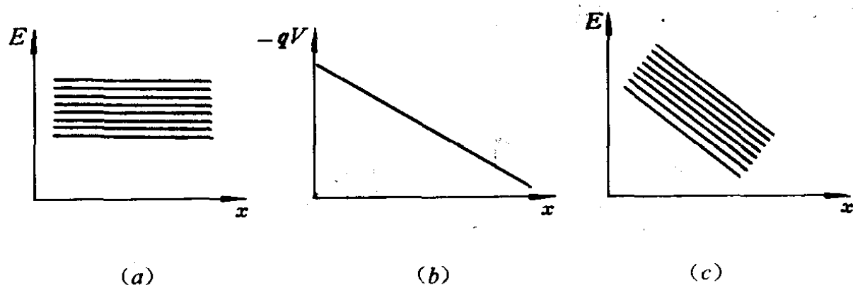
图 5-5 能带的倾斜
