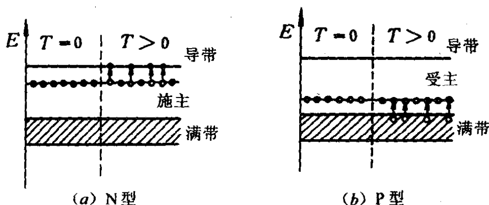
图 7-3 施主和受主
