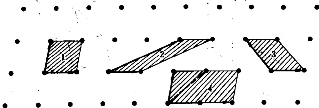
图 1-11 原胞示意图
