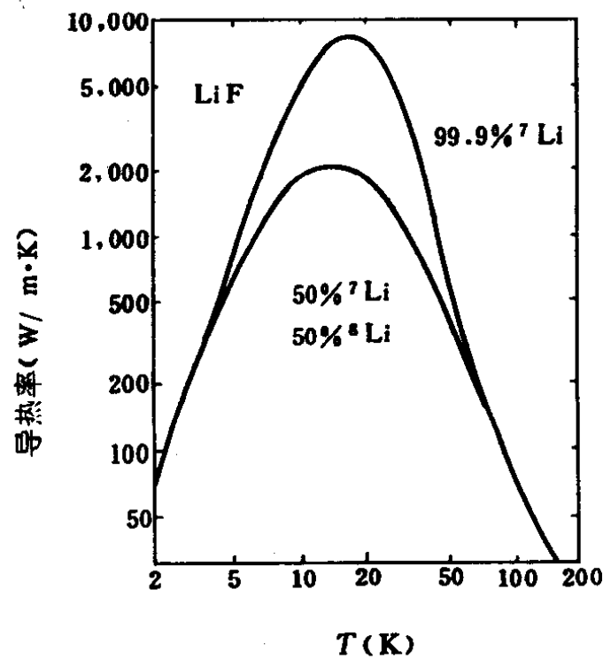
图 3-32 热导与杂质
