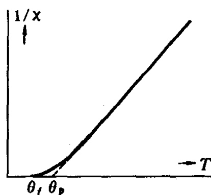
图 8-9 高温顺磁性
