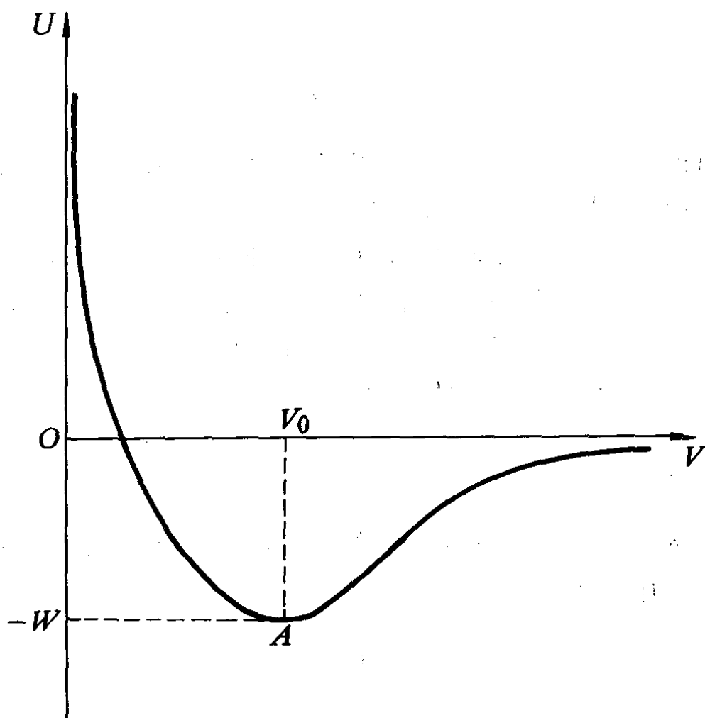
图 2-1 内能函数
