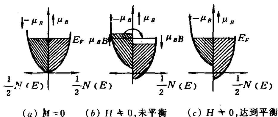
图 8-4 电子自旋顺磁性的分析
