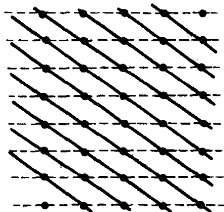
图 1-16 晶列
