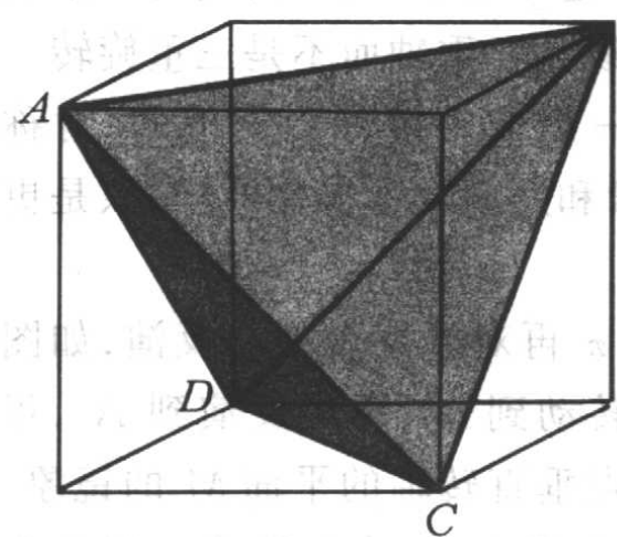
图 1-27 共四面体
