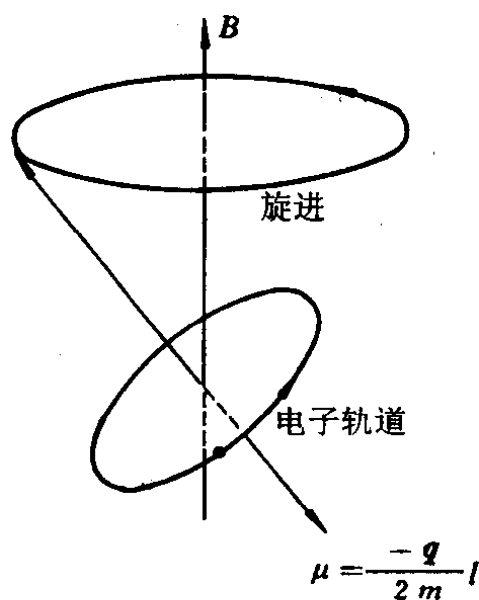
图 8-3 拉摩旋进
