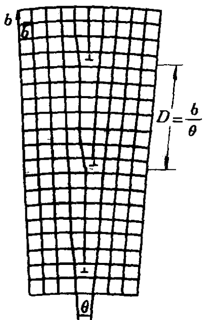
图 12-10 小角晶界
