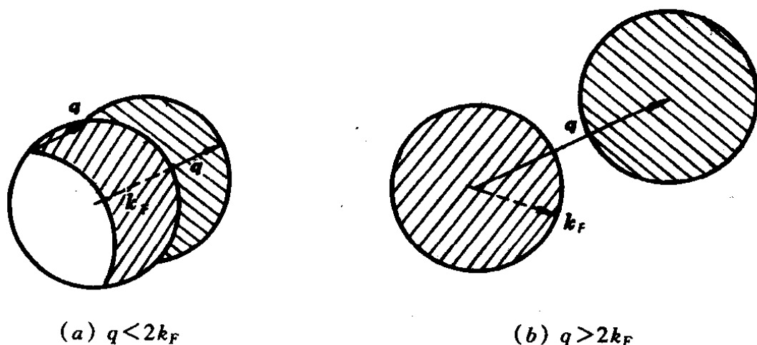
图 11-1 单电子激发
