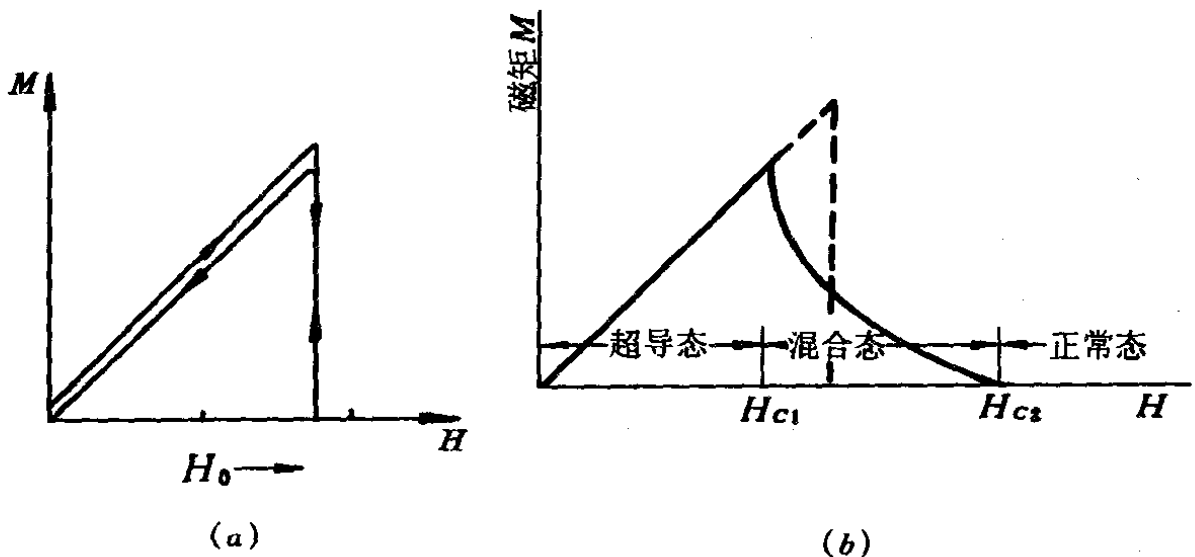
图 10-15 磁化曲线
