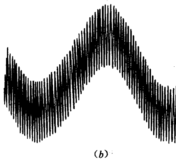
图 5-19 德·哈斯-范·阿芬效应
