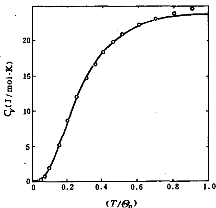
图 3-23 德拜理论与实验比较(实验点是铋的测量值)
