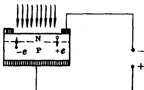
图 7-24 PN 结光生伏特效应
