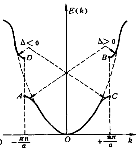
图 4-4 k = \pm \frac{n\pi}{a} 处的微扰
