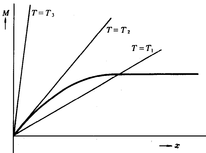
图 8-7 自发磁化图解
