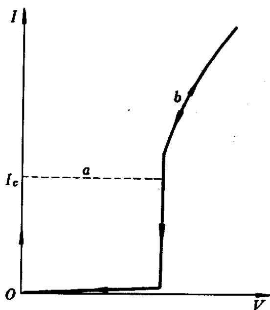
图 10-25 直流约瑟夫森效应的 电流 - 电压关系
