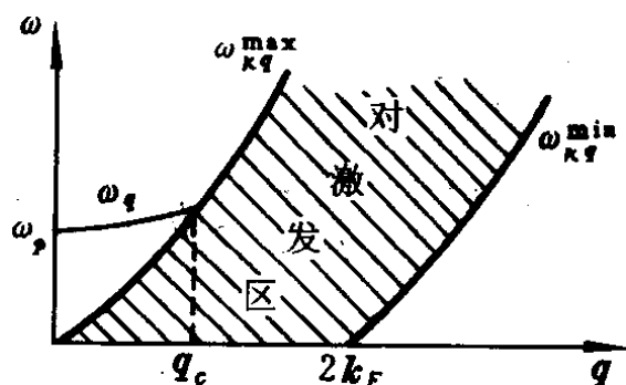
图 11-2 对激发区和等离子集体振荡的色散关系
