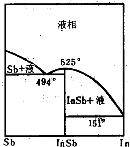
图 13-4 Sb-In 相图
