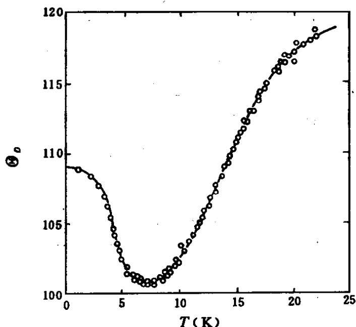
图 3-24 金属钢的德拜温度 \Theta_D 随温度的变化
