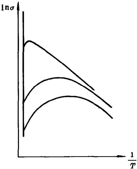
图 7-7 锗的电导率和温度关系
