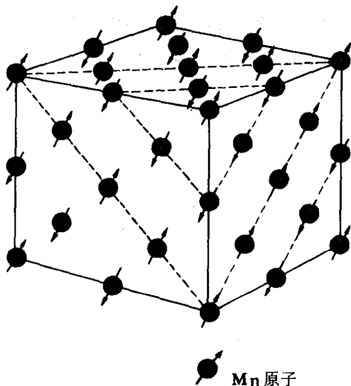
图 8-26 MnO 晶体反铁磁排列
