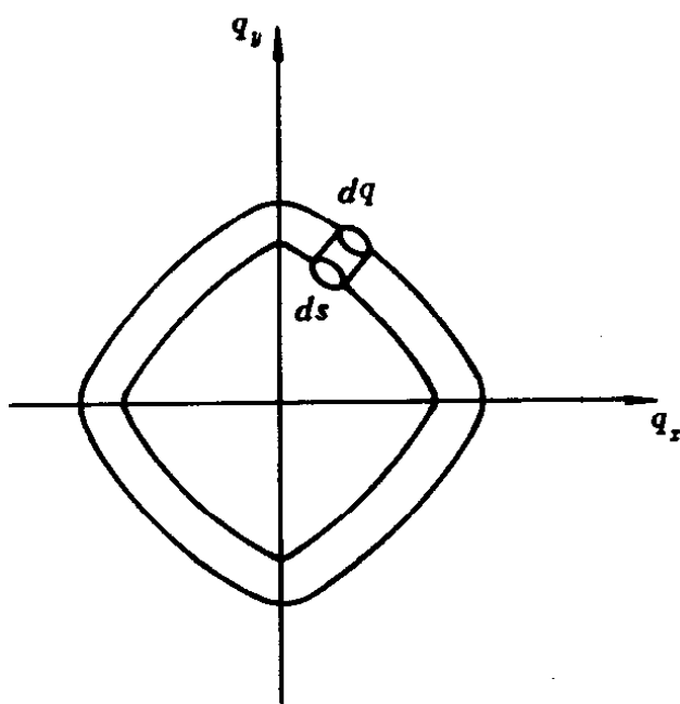
图 3-26 等频面示意图
