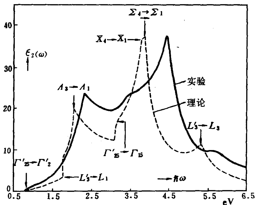
图 9-3 锗的介电常数的虚部; 实线: 实验结果; 虚线: 理论计算结果
