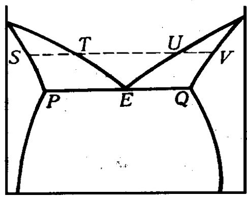
图 13-20 与 13-19 图相对应的相图
