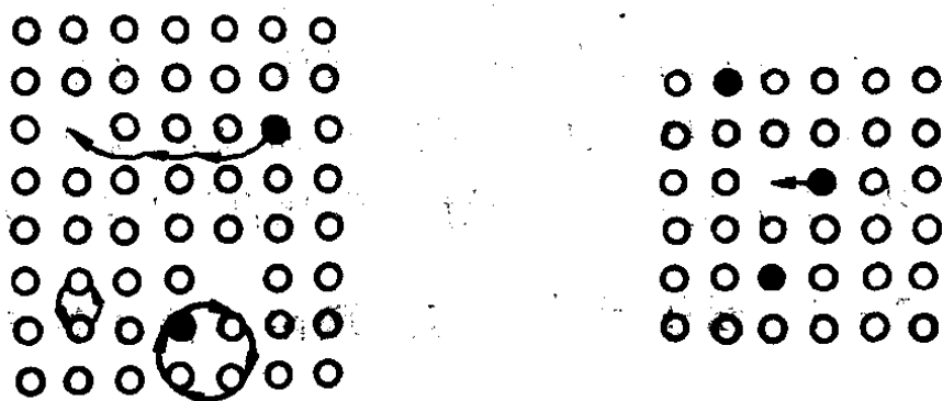
图 12-20 空位式扩散
