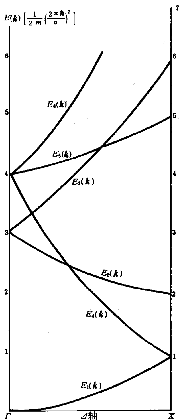
图 4-14 沿 \Delta 轴的自由电子的 E(k) 函数
