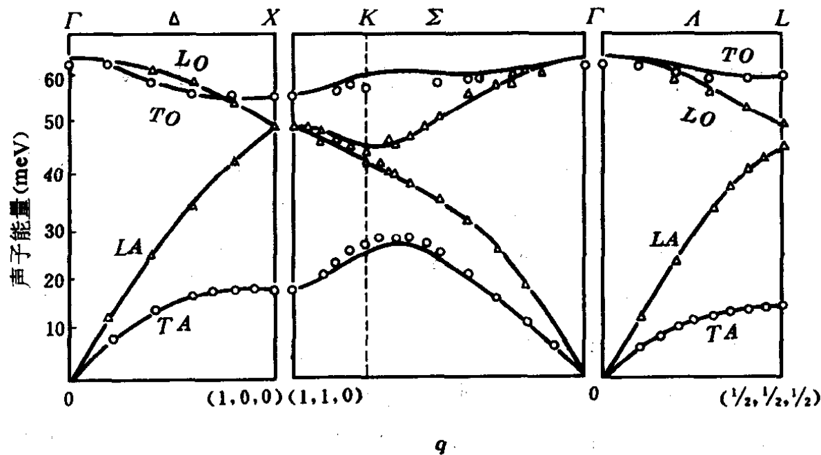
图3-10 硅的格波谱
