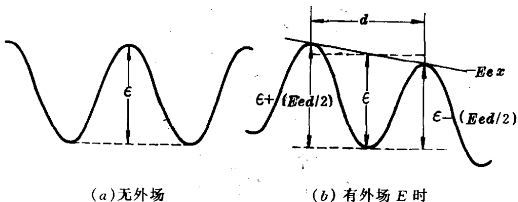
图 12-22 离子势能
