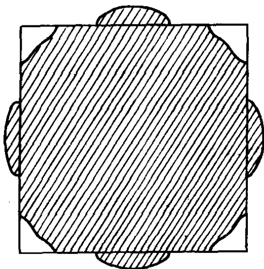
图 4-45 二价金属的费米面
