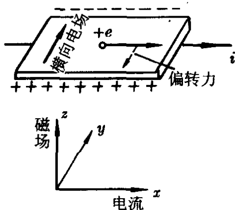
图 7-8 霍耳效应
