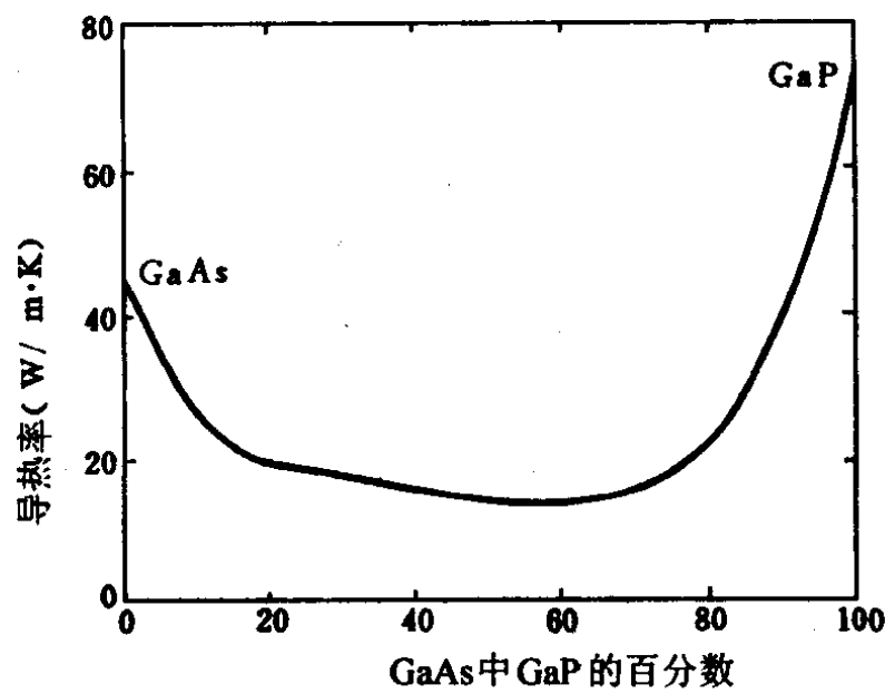
图 3-33 合金的热导
