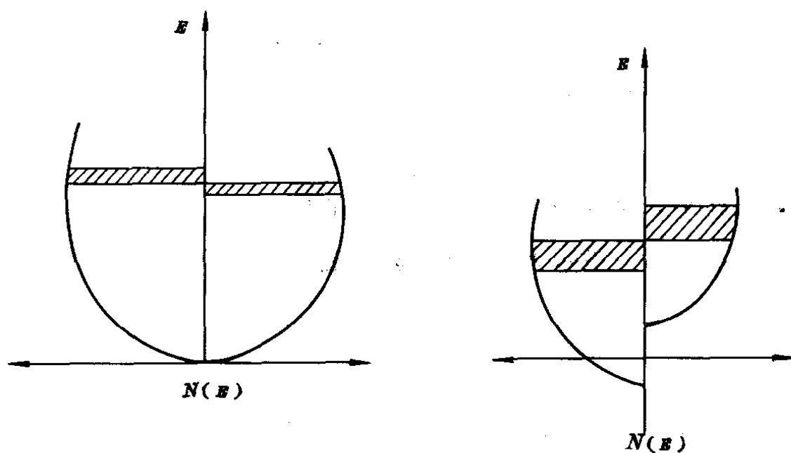
图 8-15 斯托纳模型
