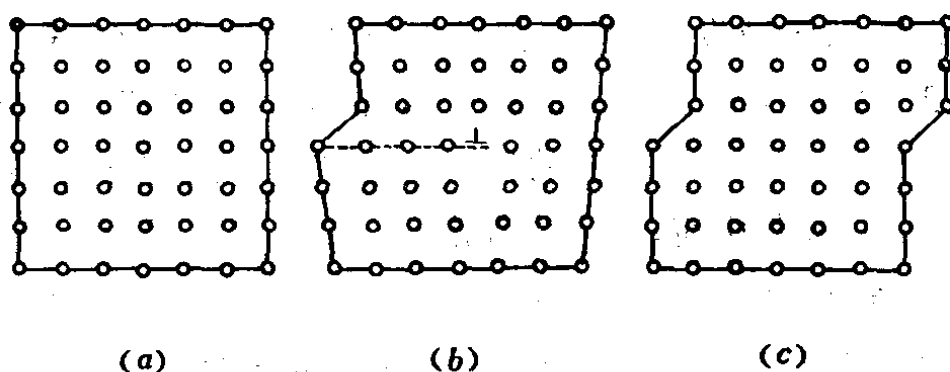
图 12-5 滑移过程图
