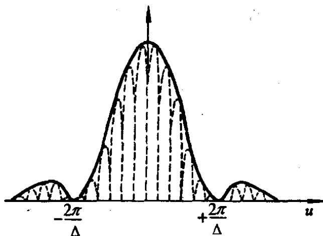
图 5-1 波包
