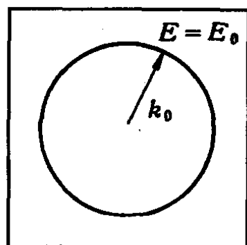
图 4-44 费米球
