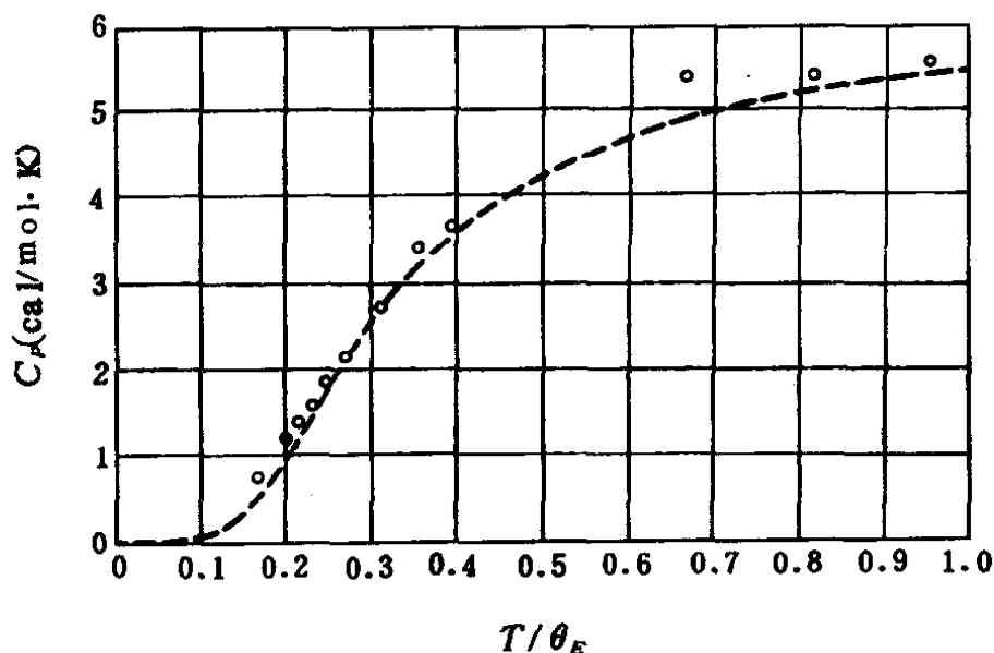
图 3-21 爱因斯坦理论与实验比较(圆点为金刚石实验值,温度以 \theta_E = \hbar\omega_0/k_B 为单位)
