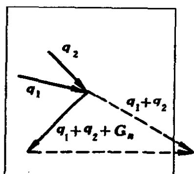
图 3-30 翻转过程
