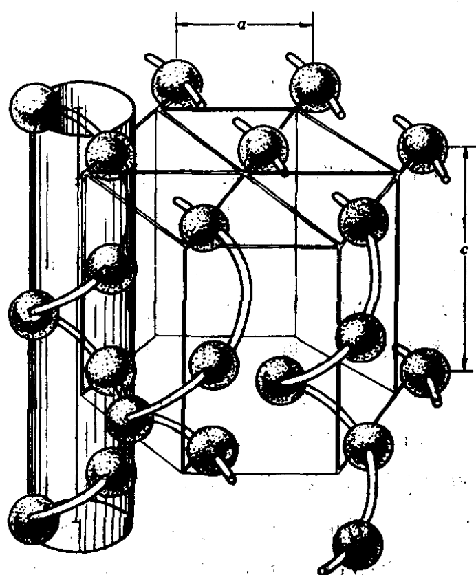
图 2-9 硒、碲的结构
