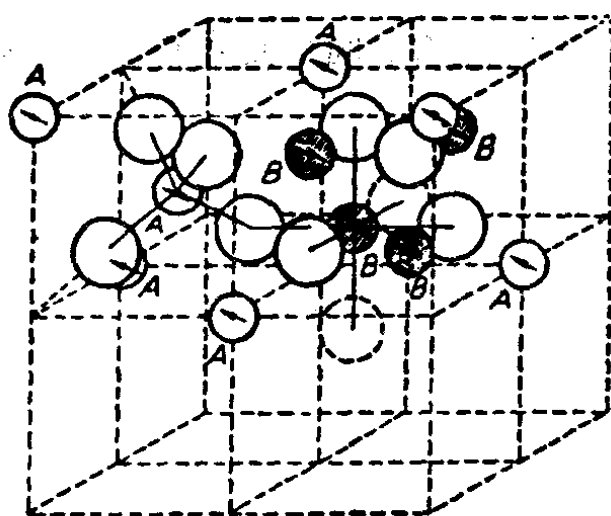
图 8-27 尖晶石结构
