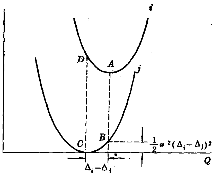
图 9-10 位形坐标图
