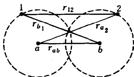
图 8-10 氢分子
