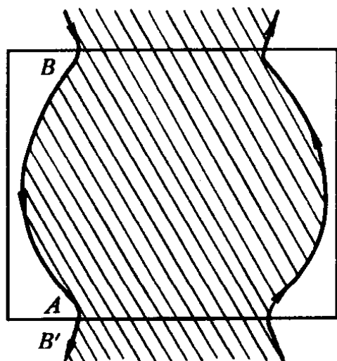
图 5-28 开轨道
