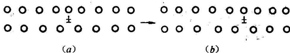
图 12-6 位错运动
