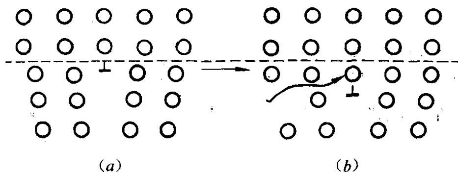
图 12-14 攀移
