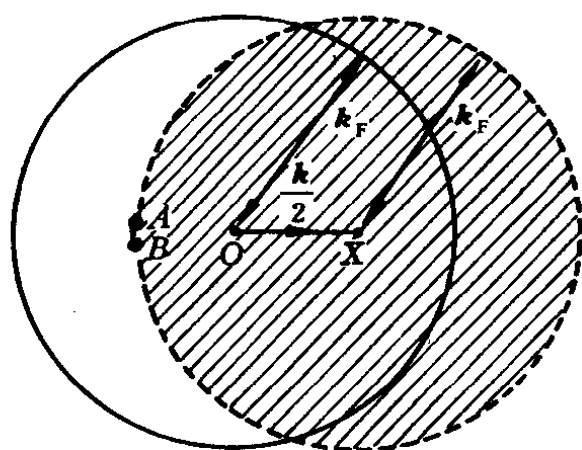
图 10-14 载流超导体的动量分布
