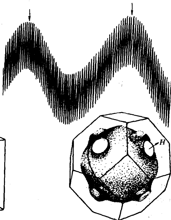
图 5-26 磁场沿 \langle 111 \rangle 方向时银的德哈·斯-范·阿尔芬效应
