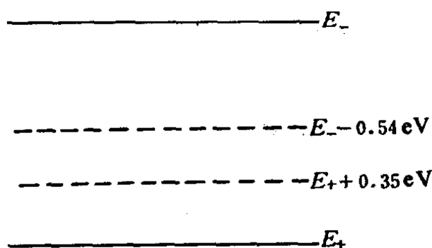
图 7-5 硅中金能级
