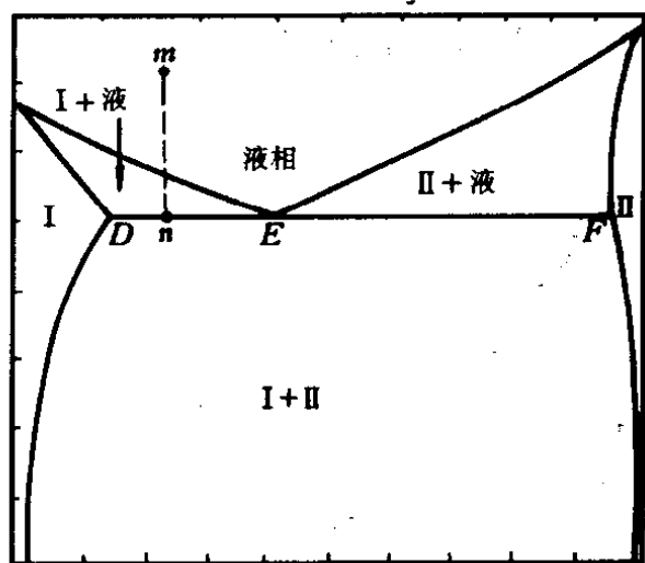
图 13-11 共晶转变
