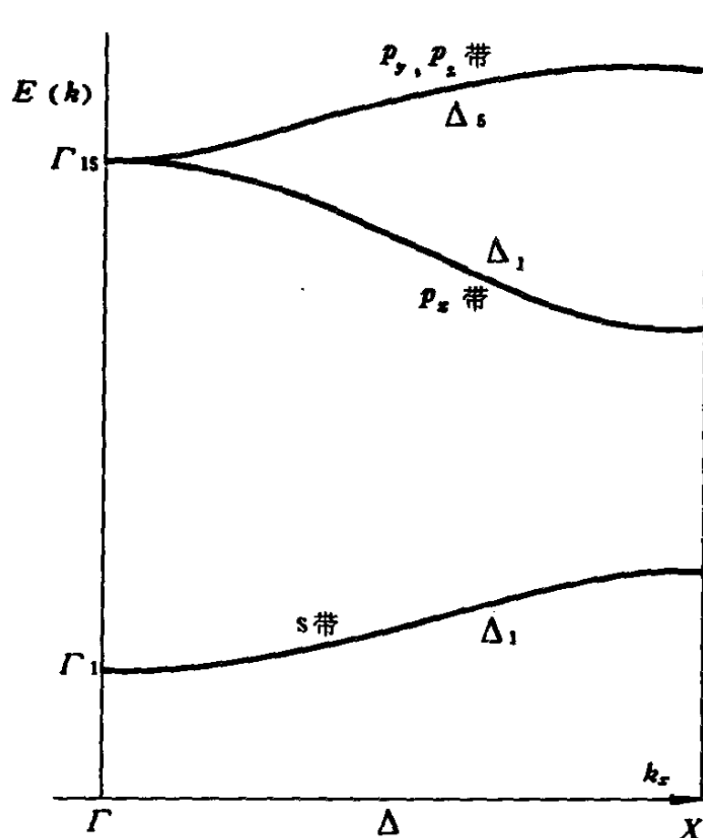
图 4-34 简单立方晶格 s 带和 p 带的对称性
