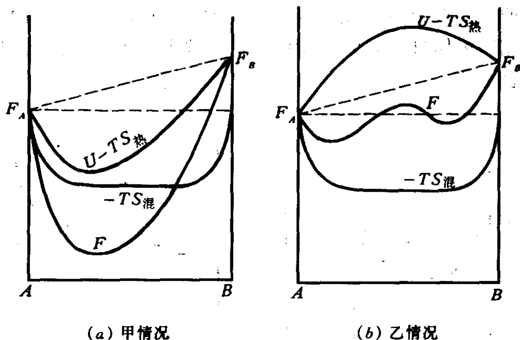
图 13-15 自由能曲线
