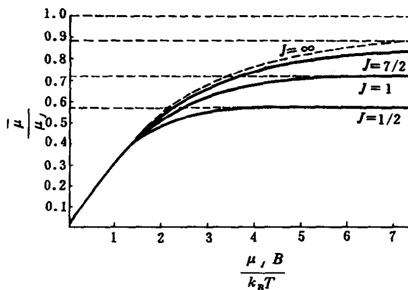
图 8-5 (\bar{\mu}/\mu_J) 随 (\frac{\mu_J B}{k_B T}) 的变化
