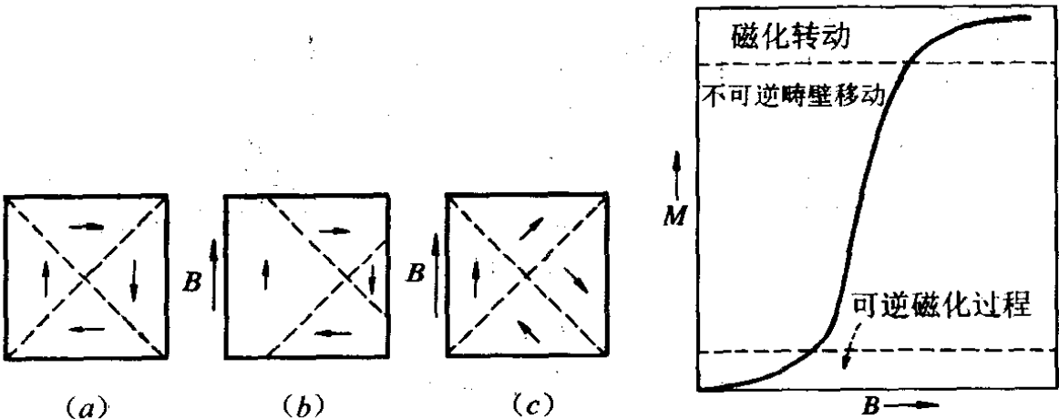
图 8-21 磁化过程的分析
