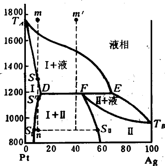
图 13-3 Pt-Ag 相图
