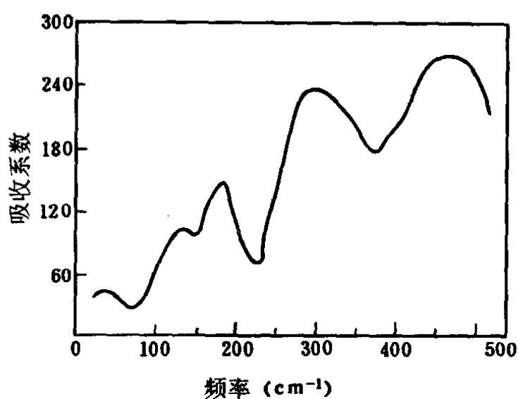
图 3-37 非晶硅的红外吸收光谱
