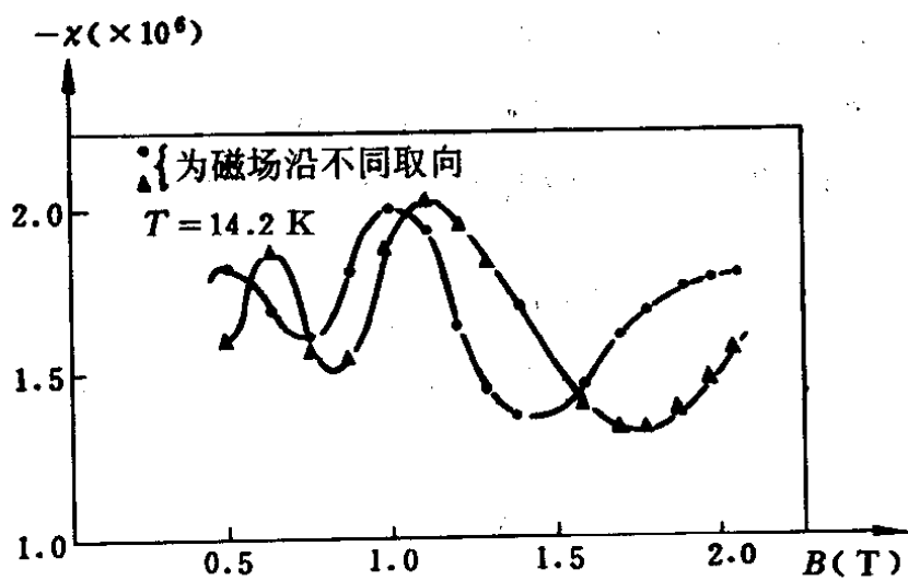
图 5-18 14.2K 铈单晶磁化率随磁场的变化
