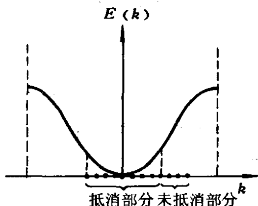
图 5-10 外场改变对称分布
