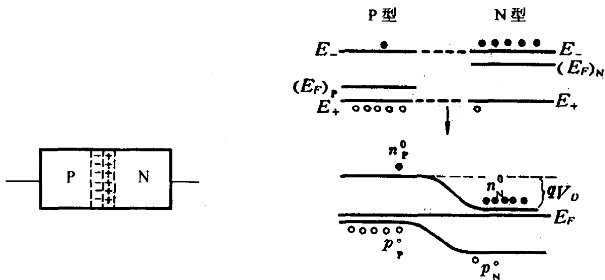
图 7-13 PN 结势垒
