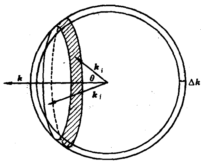
图 10-12 形成总的波矢量为 k 的电子对的示意图
