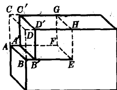
图 12-4 局部的滑移
