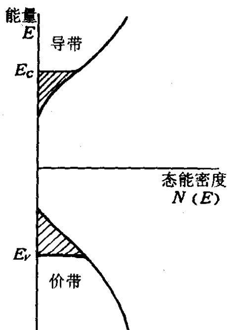
图 7-26 非晶态半导体的态能密度
