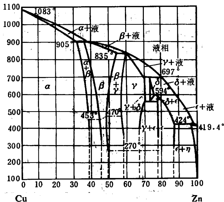
图 13-5 Cu-Zn 相图
