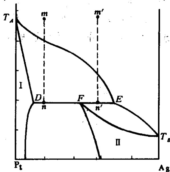
图 13-12 包晶转变
