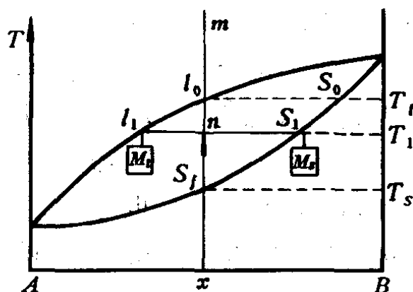
图 13-9 连续固溶体相图及其相变过程
