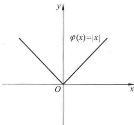
Fig.2-6-3 Absolute-value function \varphi(x) = |x|
