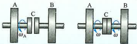
图 3-20 两飞轮的摩擦啮合
