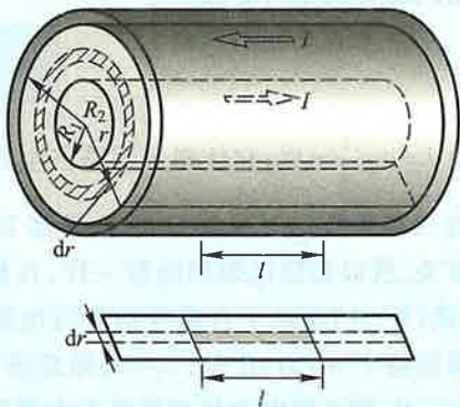
图 9-24 电缆的自感
