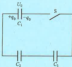
图 7-53 电容器的连接
