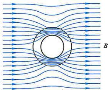
图 8-60 磁屏蔽
