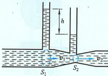
图 3-27 文丘里流量计
