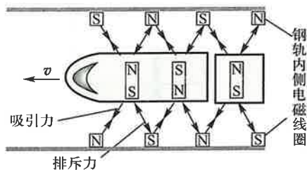
(b) 电磁驱动原理图
