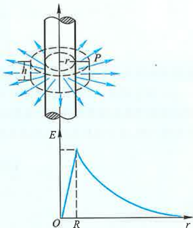
图 7-24 “无限长”均匀带电圆柱体的电场
