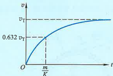
图 1-30 沉降速度增长曲线
