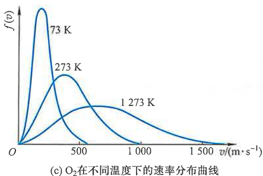
图 5-5 麦克斯韦速率分布曲线
