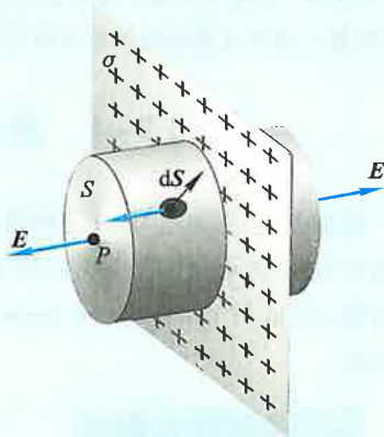
图 7-25 “无限大”均匀带电平面的电场
