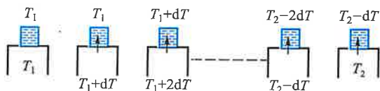
图 6-1 一系列有微小温度差的恒温热源
