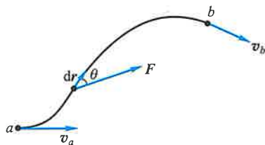
图 2-21 动能定理
