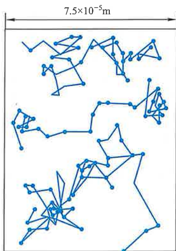
图 5-2 布朗运动
