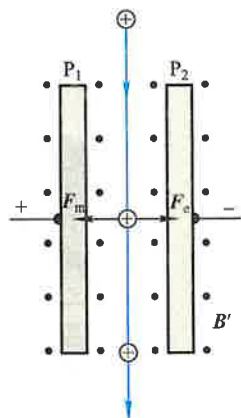
图 8-37 速度选择器
