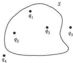
图 7-22 闭合曲面 内外均有电荷
