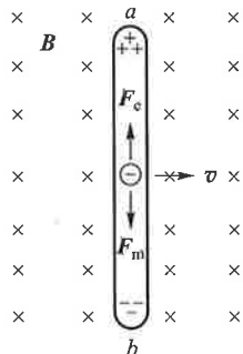
图 9-9 动生电动势的电子理论解释
