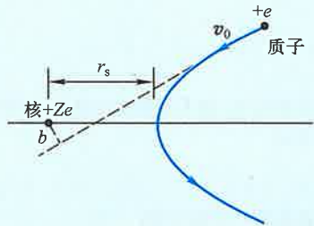
(1) 图 2-38 质子通过原子核时的轨迹
