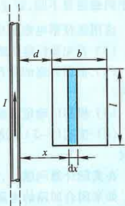
图 9-7 电磁感应举例
