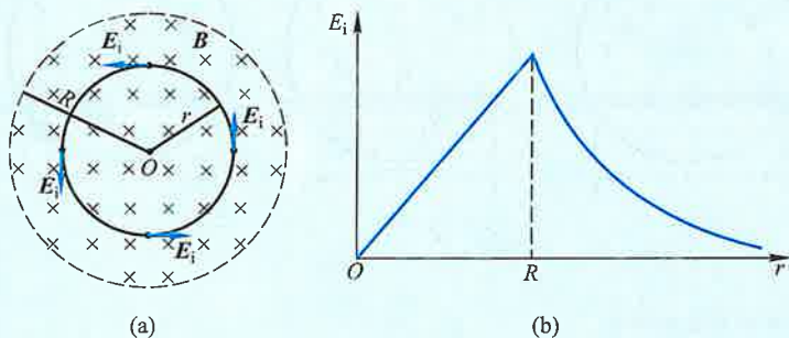
图 9-16 螺线管内外的感生电场
