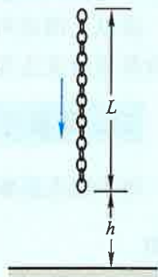
图 2-8 链条下落
