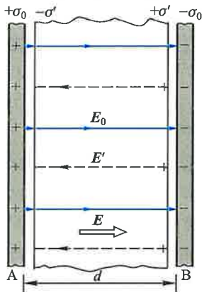
图 7-63 电介质中的电场强度
