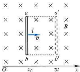
图 9-8 动生电动势
