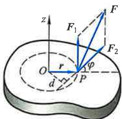
图 3-3 力矩
