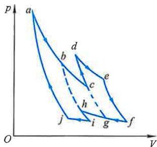
图 6-21 一个可逆循环,
