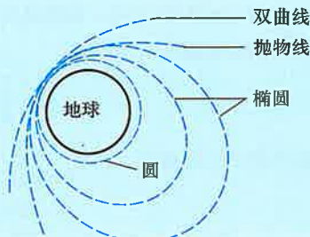
图 2-37 宇宙速度
