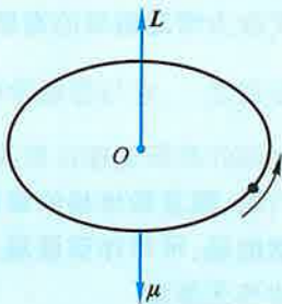
角动量方向的关系
