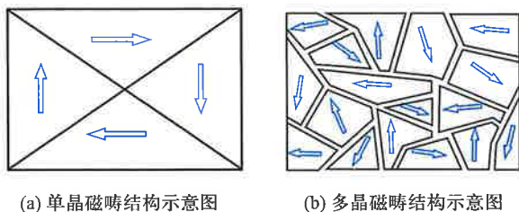
图 8-55 磁畴
