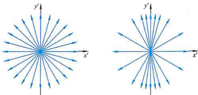
(a) 点电荷在静止或作低速运动时的电场线分布
