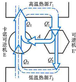
图 6-20 卡诺定理的证明
