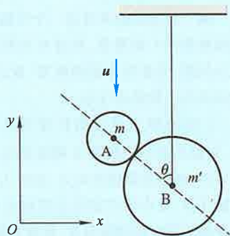
图 2-42 两球的斜碰
