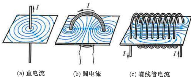
图 8-9 几种不同形状电流磁场的磁感应线
