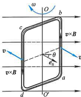
图 9-13 磁场中转动线圈的感应现象
