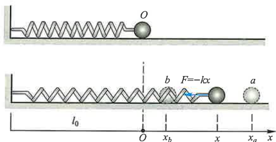
图 2-25 弹性力的功
