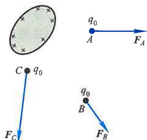
图 7-5 检验电荷 q_0 在电场中受力的情况
