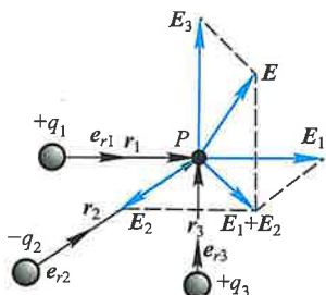
图 7-7 点电荷系的电场强度
