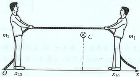
图 2-11 两人在冰面上对拉
