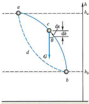
图 2-24 重力的功
