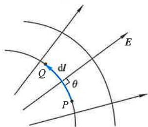
图 7-32 等势面与电场线正交的证明
