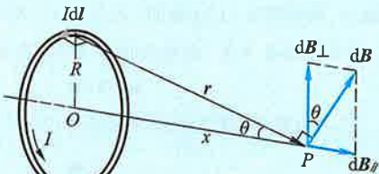
图 8-14 圆电流轴线上磁场的计算
