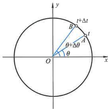
图 1-15 角位移
