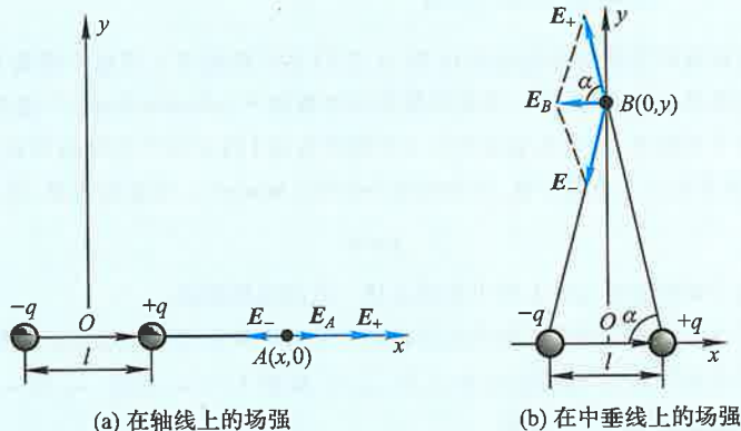
图 7-8 电偶极子
