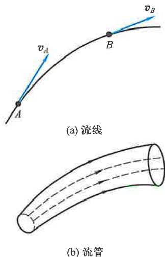
图 3-24 流线和流管
