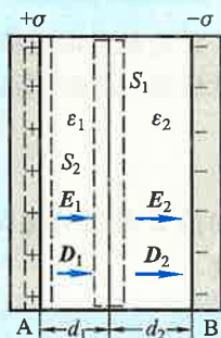
图 7-68 两平行板间 充满两种电介质
