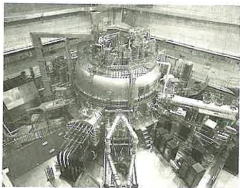
图 8-34 托卡马克
