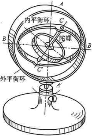
(a) 现代回转仪中的万向支架
