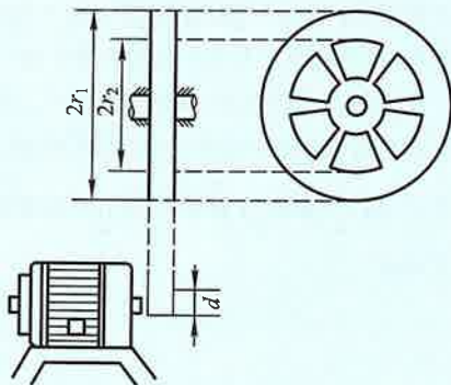
图 3-12 冲床上的转动飞轮
