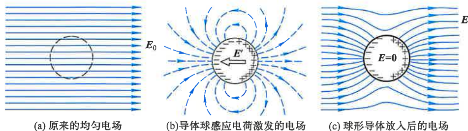
图 7-36 电场中的球形导体
