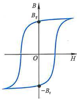
图 8-59 硬磁材料磁滞回线
