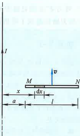
图 9-12 在长直导线产生的磁场中运动的金属棒
