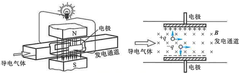
图 8-39 磁流体发电机原理示意图
