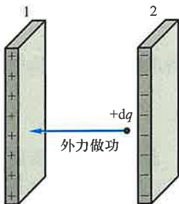
图 7-69 电容器的充电过程
