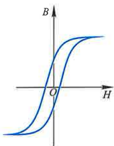
图 8-58 软磁材料磁滞回线
