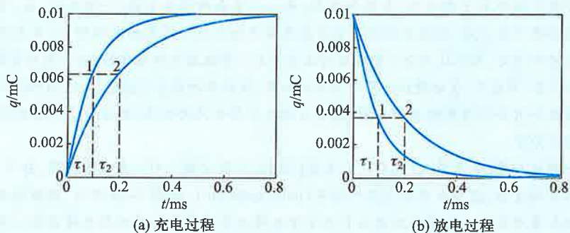
图 7-55 电容器在充放电过程中 q 随 t 变化的曲线 ( \tau_2 > \tau_1 )
