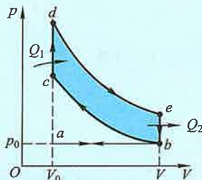
图 6-14 奥托循环
