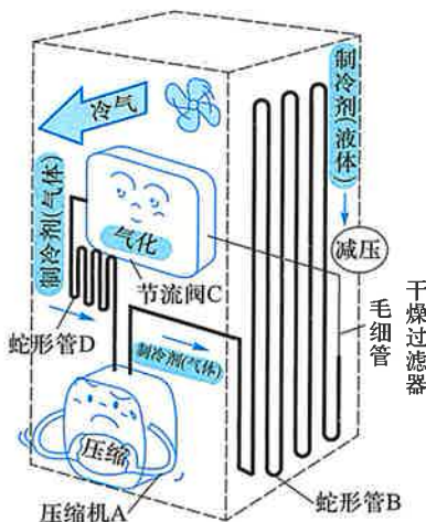
图 6-13 压缩型制冷机
