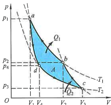
图 6-16 卡诺逆循环(制冷机)的 p - V 图
