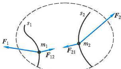
图 2-31 系统的外力和内力的功
