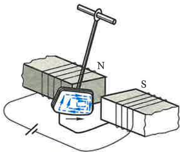
图 9-21 阻尼摆
