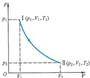
图 5-1 平衡态和准静态过程的示意图
