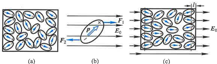
图 7-60 极性分子的极化示意图
