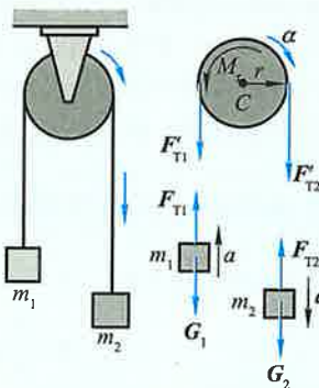
图 3-9 阿特伍德机
