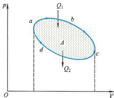
图 6-9 正循环过程
