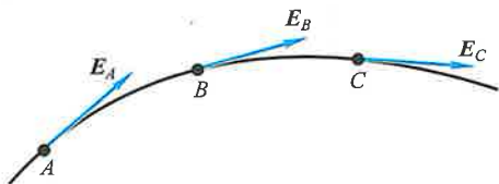
图 7-15 电场线
