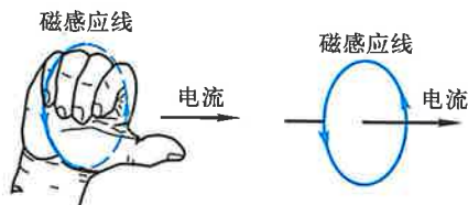
图 8-10 磁感应线环行方向与电流方向的关系
