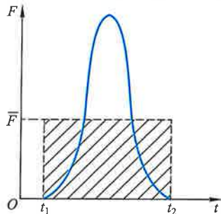
图 2-5 冲击力示意图
