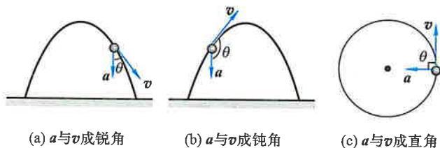
图 1-6 曲线运动中的加速度与速度的方向
