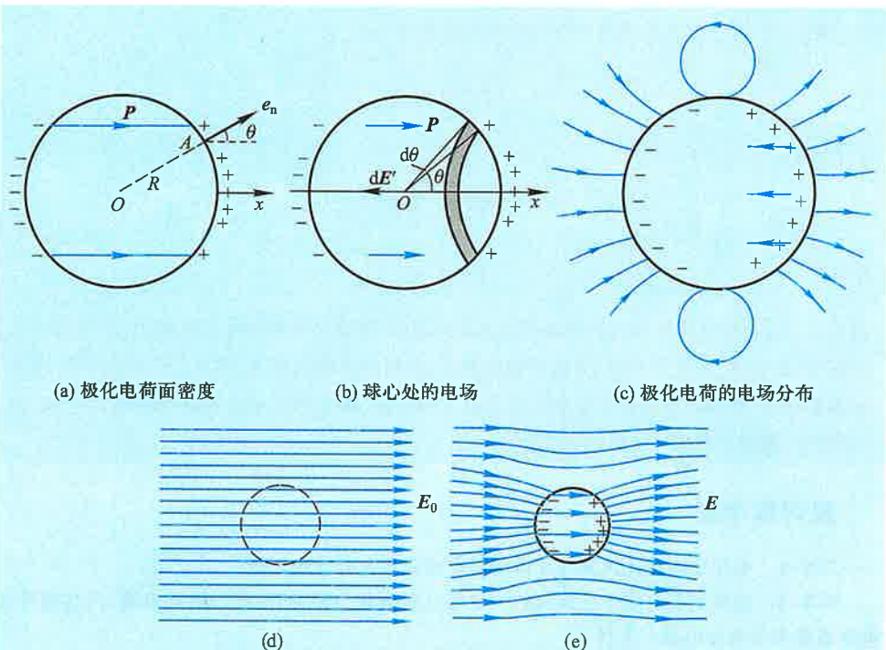
图 7-64 电介质球
