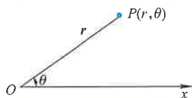
图 1-14 平面极坐标系
