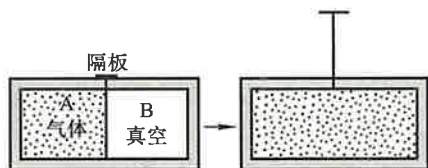
图 6-19 气体的自由膨胀
