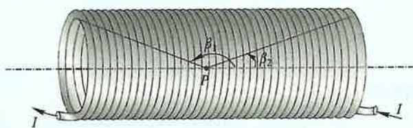
(a) 载流直螺线管
