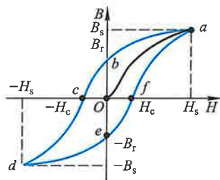
图 8-54 磁滞回线
