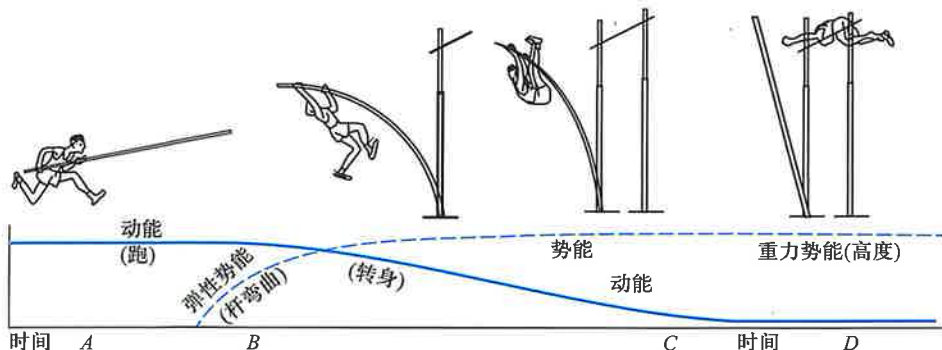
图 2-32 撑竿跳高中的能量转化
