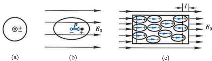
图 7-59 无极分子极化示意图
