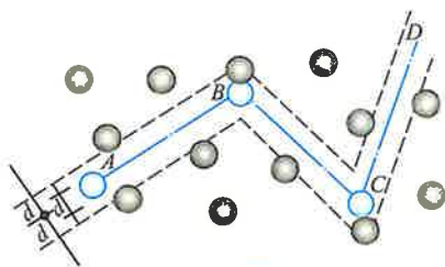
图 5-9 \bar{\lambda} 及 \bar{Z} 的计算
