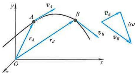
图 1-4 速度的增量
