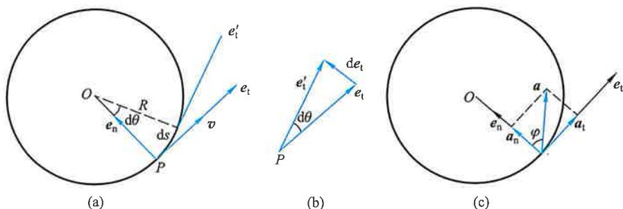
图 1-13 自然坐标系
