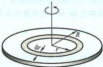
图 3-8 圆盘转动惯量的计算
