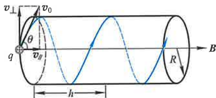
图 8-29 带电粒子在匀强磁场中的运动(初速 v_0 与 B 斜交)
