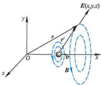
图 9-35 电荷在 K 系内的场强
