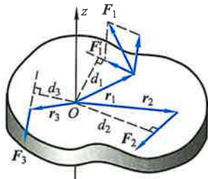
图 3-4 几个力的总力矩
