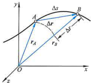
图 1-2 曲线运动中的位移
