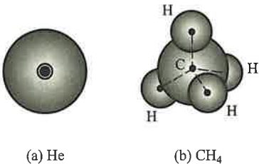
图 7-58 无极分子
