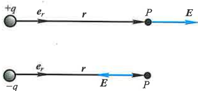
图 7-6 点电荷的电场强度
