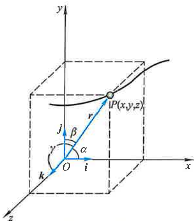
图 1-1 位矢
