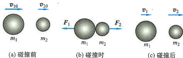
图 2-40 两球的对心碰撞
