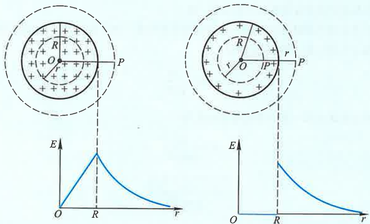
(a) 均匀带电球体的电场强度曲线
