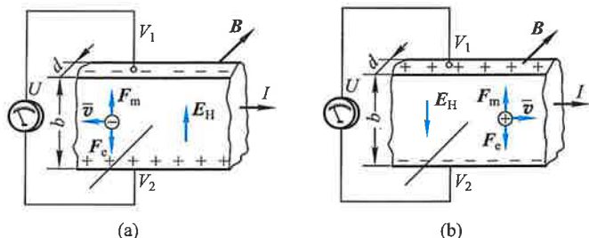
图 8-38 霍尔效应
