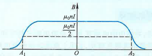
图8-17 螺线管轴线上的磁场分布
