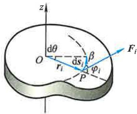
图 3-11 力矩的功
