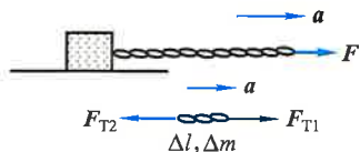
图 1-24 绳中的张力
