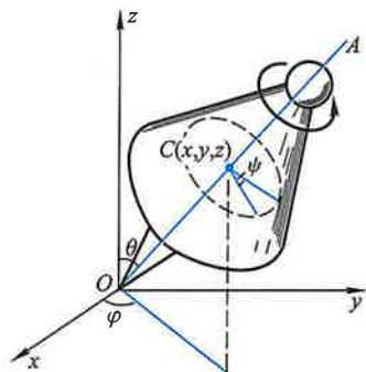
图 3-2 刚体的自由度
