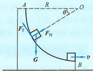
图 2-34 物体沿圆轨道下滑
