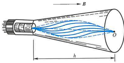
图 8-30 磁聚焦
