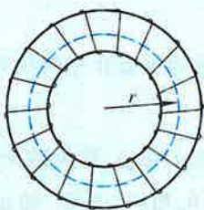
图 8-51 螺绕环内的磁场
