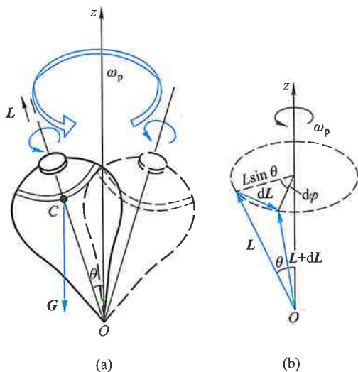
图 3-22 陀螺的进动
