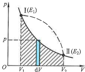
图 6-3 气体膨胀做功的图示
