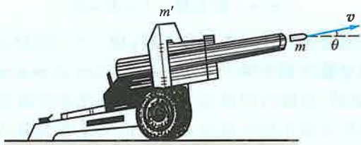
图 2-9 炮车的反冲
