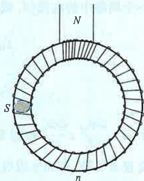
图 9-27 螺绕环与小线圈间的互感
