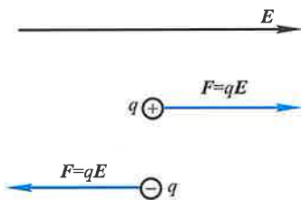
图 7-12 电场对正、负电荷作用力的方向
