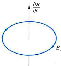
图 9-15 \mathbf{E}_i 和 \frac{\partial \mathbf{B}}{\partial t} 成左手螺旋关系
