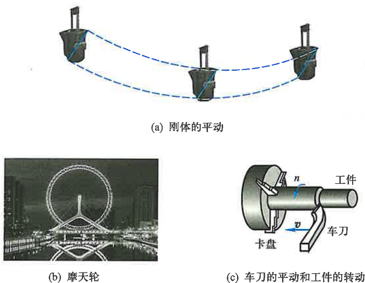
图 3-1 平动和转动
