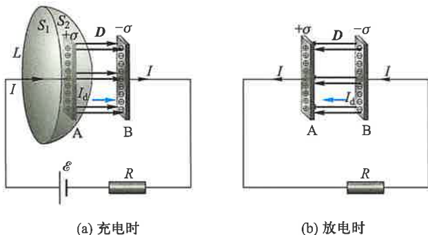
图 9-31 位移电流
