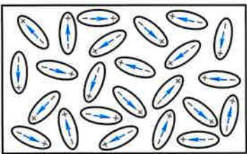
图 7-57 由极性分子组成的电介质, 总的电偶极矩的矢量和等于零
