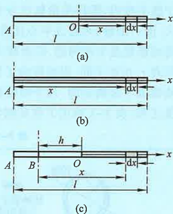
图 3-7 细棒的转动惯量计算
