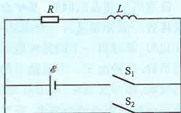
图 9-25 RL 电路
