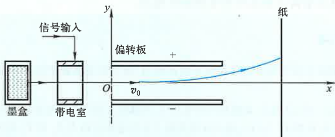
图 7-14 静电喷墨打印机机构示意图
