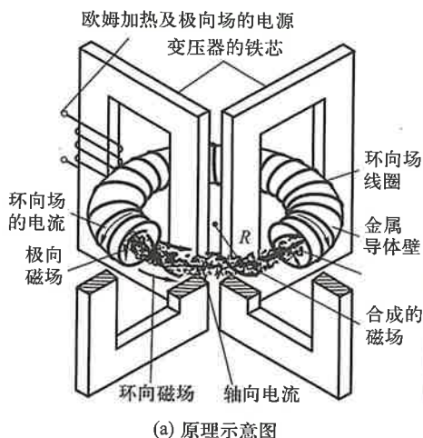
图 8-34 托卡马克
