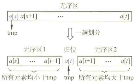
图 3.2 快速排序的一趟排序过程
