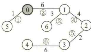
图 9.2 G 的一棵最小生成树
