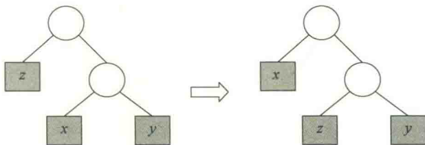
图 7.10 交换 x, z 结点
