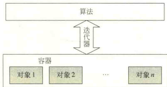
图 1.10 容器、算法和迭代器之间的关系
