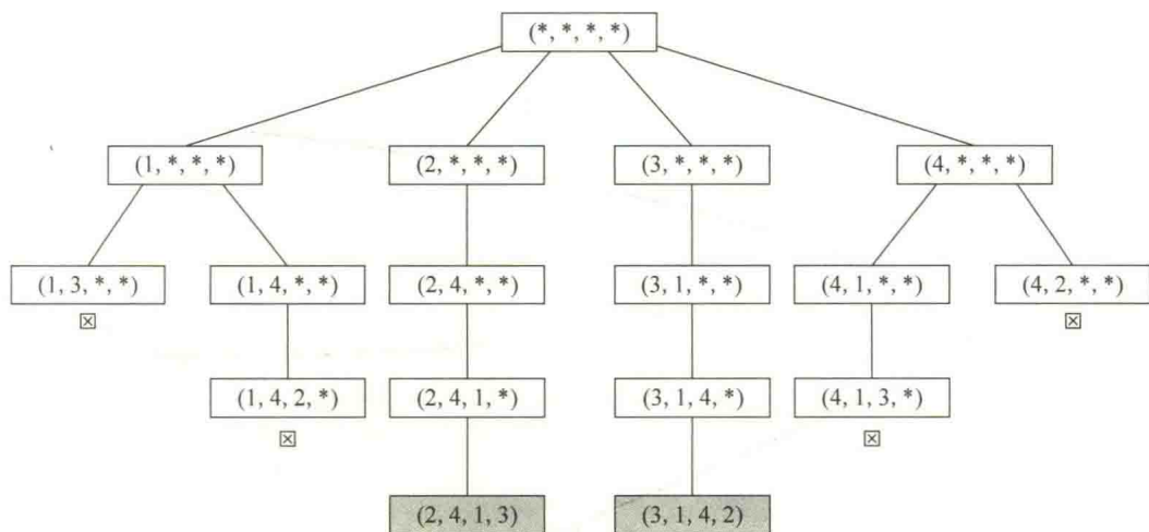
图 5.4 4 皇后问题的解空间树
