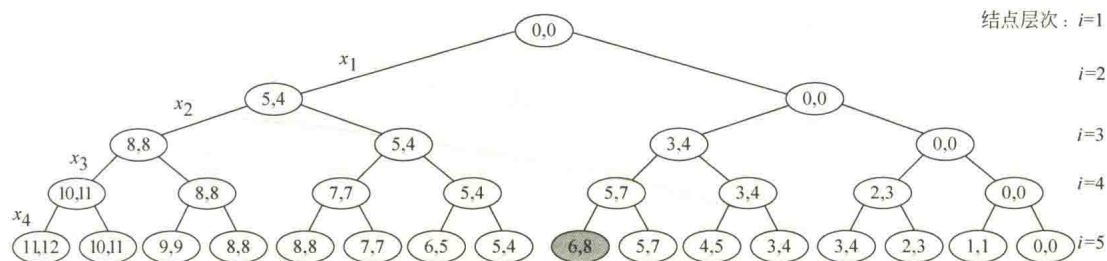
图 5.10 描述背包问题求解过程的解空间树
