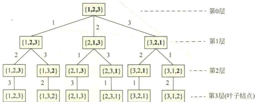
图 5.9 求全排列的解空间树
