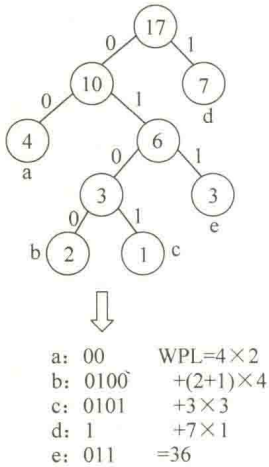
图 7.9 产生哈夫曼编码
