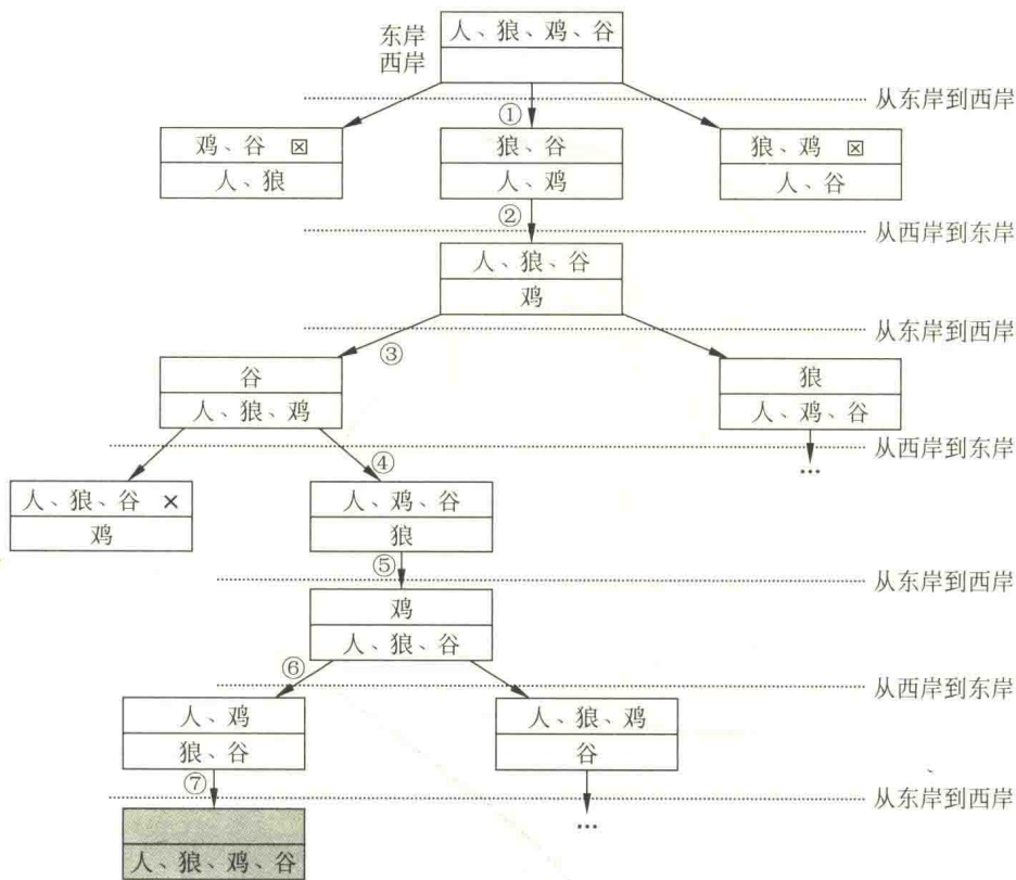
图 5.3 农夫过河的部分搜索空间
