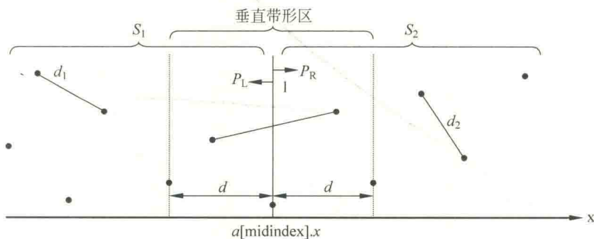
图 10.19 采用分治法求最近点对
