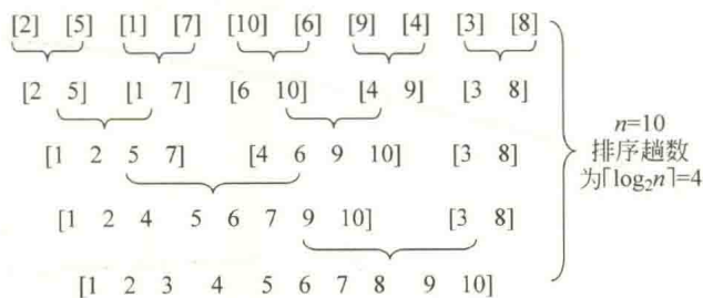
图 3.4 自底向上的二路归并排序过程
