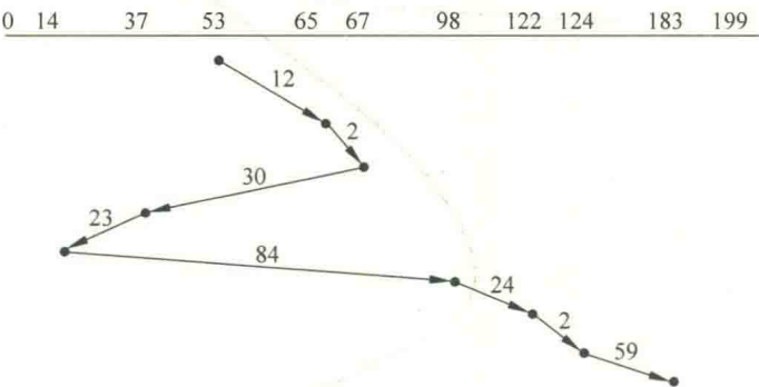
图 7.2 最短寻道时间优先算法的磁盘调度过程
