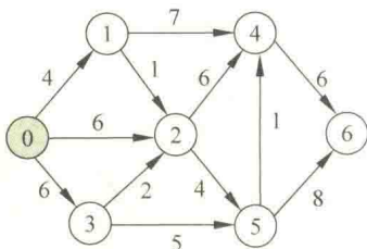
图 9.10 一个带权有向图
