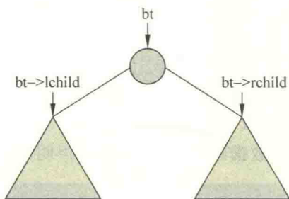
图 2.2 二叉树 bt 的一般结构
