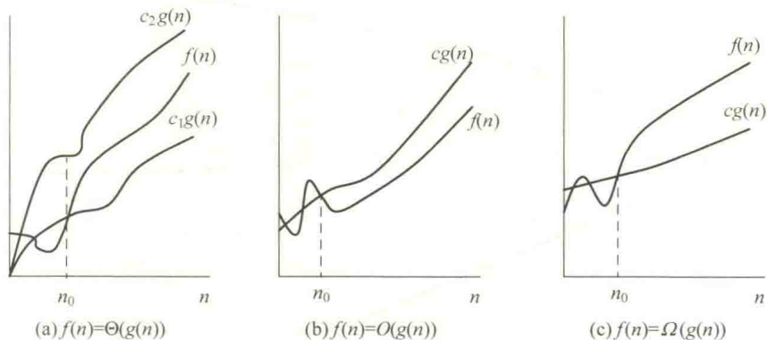
图 1.8 3 种符号的图例
