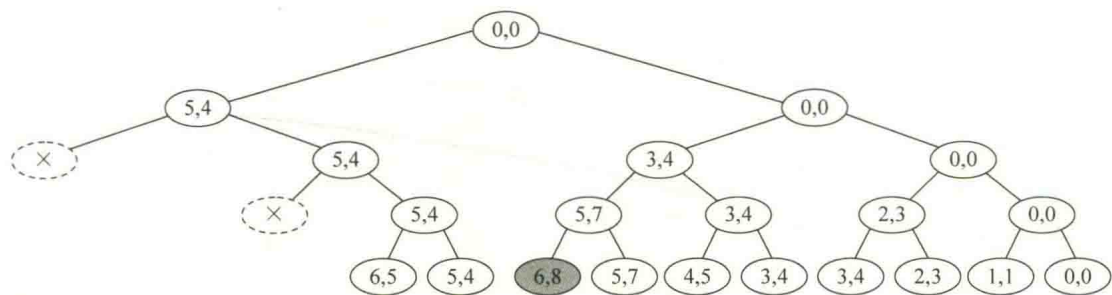
图 5.11 剪枝后的解空间树
