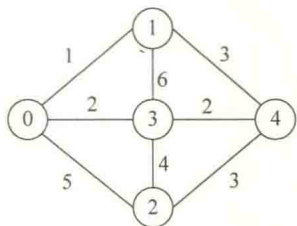
图 12.2 一个带权无向连通图
