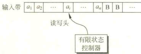
图 11.1 图灵机的基本结构
