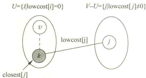
图 9.3 顶点集合 U 和 V-U
