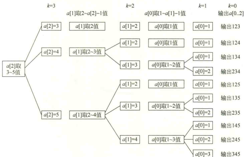
图 4.9 求从 1~5 中取 3 个整数的组合的过程
