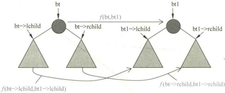
图 2.12 二叉树的复制
