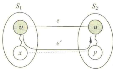
图 9.7 证明克鲁斯卡尔算法的正确性
