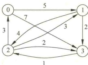
图 9.15 一个带权有向图
