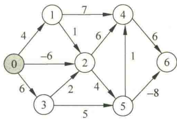
图 9.12 一个带负权的有向图
