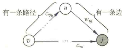
图 9.8 从顶点 v 到顶点 j 的路径比较
