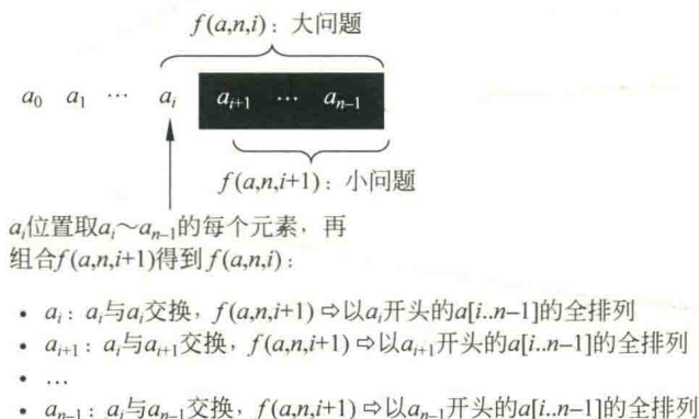
图 5.7 求 f(a, n, i) 的过程
