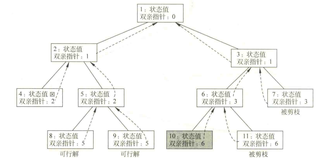
图 6.4 每个结点保存指向双亲的指针
