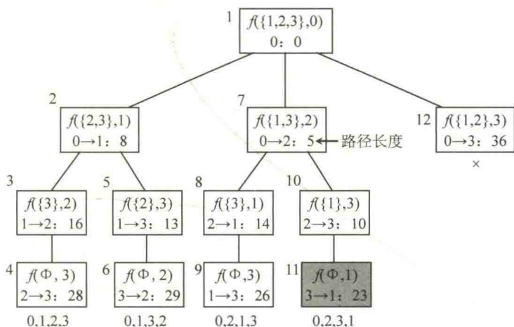
图 9.19 用回溯法求解 TSP 问题的搜索空间
