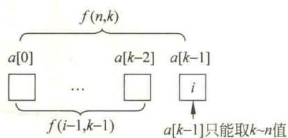
图 4.8 求 f(n, k) 的过程
