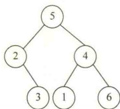
图 2.20 一棵二叉树
