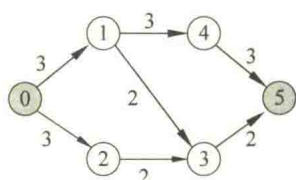
图 9.25 一个网络流
