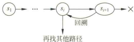
图 5.5 回溯过程
