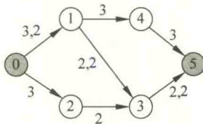
图 9.26 一个网络流
