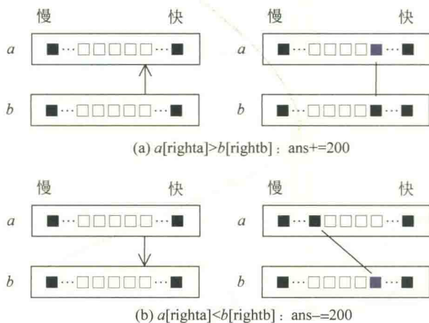
图 7.6 两者最快的马的速度不相同
