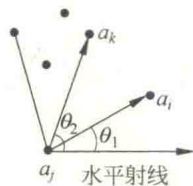
图 10.14 求点 a_i , 使得 a_j a_i 与以 a_j 为起点的水平方向射线的角度最小
