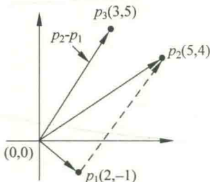
图 10.2 向量的减法
