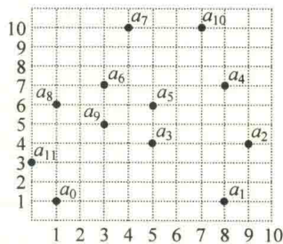
图 10.23 一个点集 A
