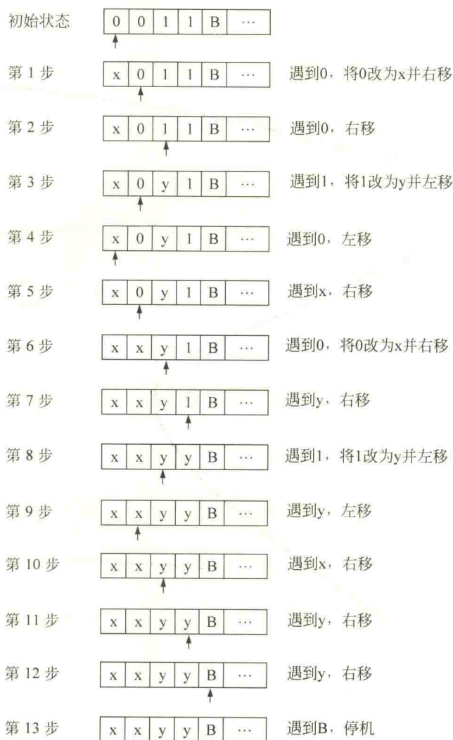
图 11.2 识别 0011 的过程
