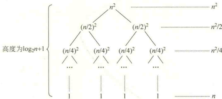
图 2.18 一棵递归树
