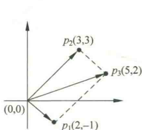
图 10.1 向量的加法
