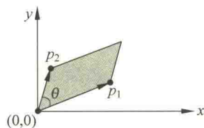
图 10.4 两个向量的叉积
