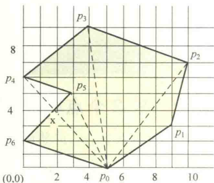
图 10.11 一个多边形
