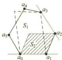
图 10.22 找粗边的过程
