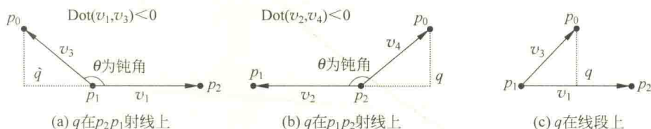
图 10.6 投影点 q 的 3 种情况
