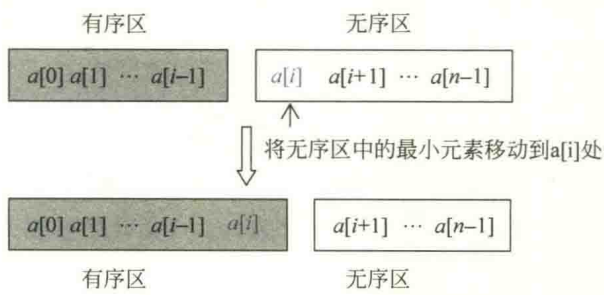
图 2.13 一趟排序
