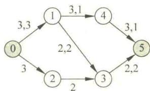
图 9.28 一个网络流
