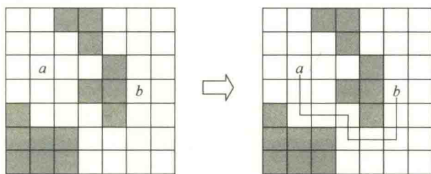
图 6.15 一个布线的例子
