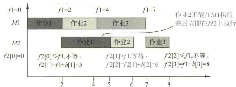
图 5.19 另一种调度方案的总时间计算
