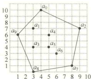
图 10.13 一个点集的凸包
