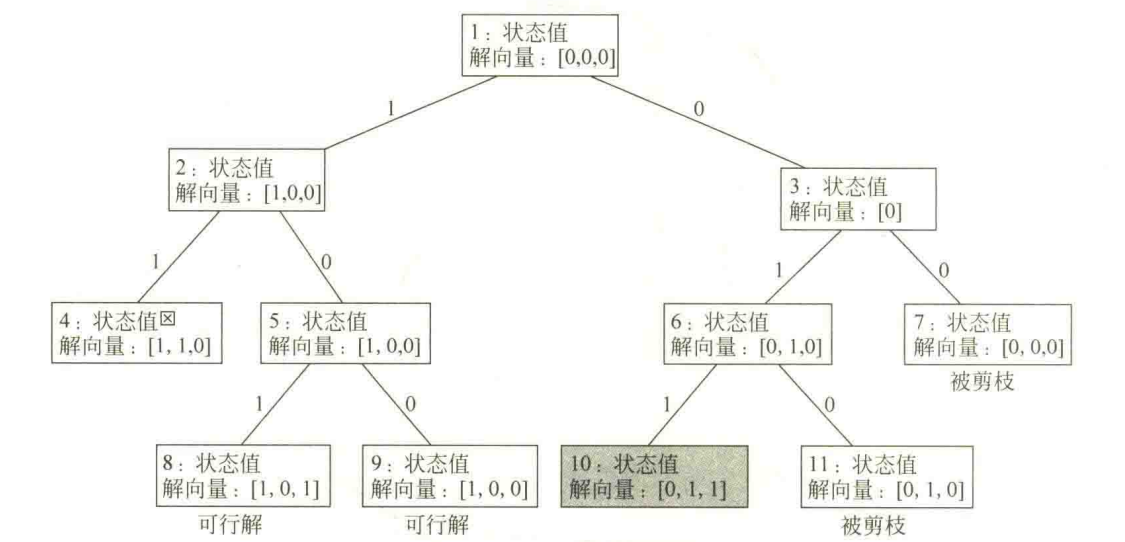
图 6.3 每个结点保存可能的解向量
