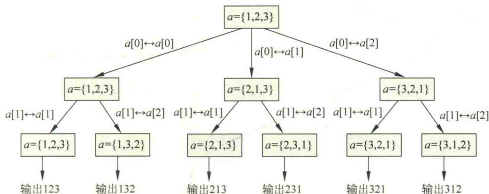
图 5.8 求 a[] = \{1, 2, 3\} 的全排列的过程
