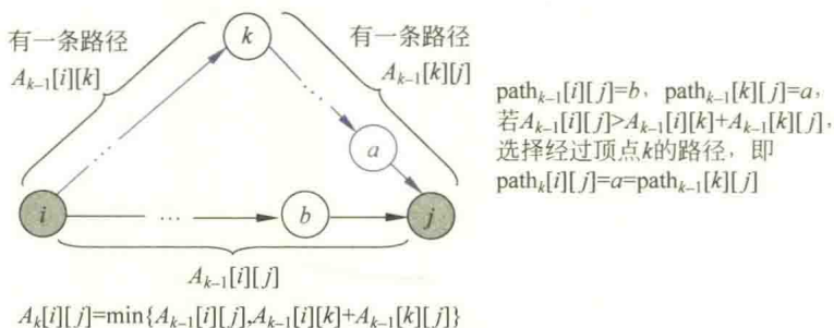
图 9.14 考虑顶点 k 时路径的调整
