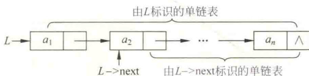
图 2.1 不带头结点的单链表 L 的一般结构
