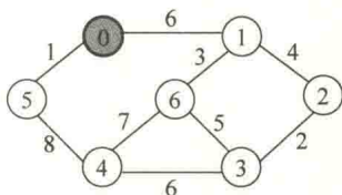
图 9.1 一个带权连通图 G
