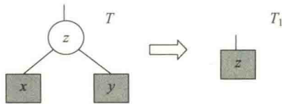
图 7.11 由 T 删除 x, y 结点得到 T_1
