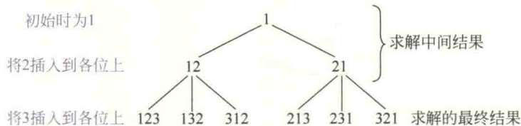
图 4.7 产生 1 \sim 3 全排列的过程
