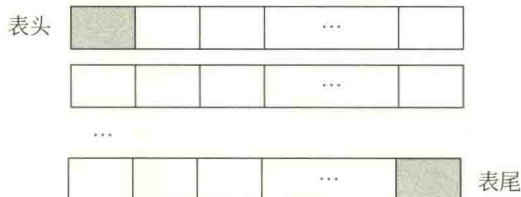
图 1.13 deque 容器的存储方式
