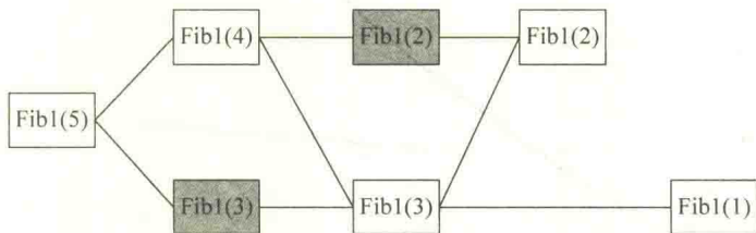
图 8.2 求 Fib1(5)的过程
