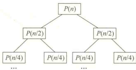
图 3.1 二分法的基本策略
