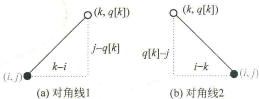
图 2.15 两个皇后构成对角线的情况
