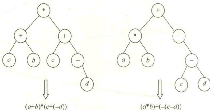
图 2.21 两棵表达式树对应等价的中缀表达式
