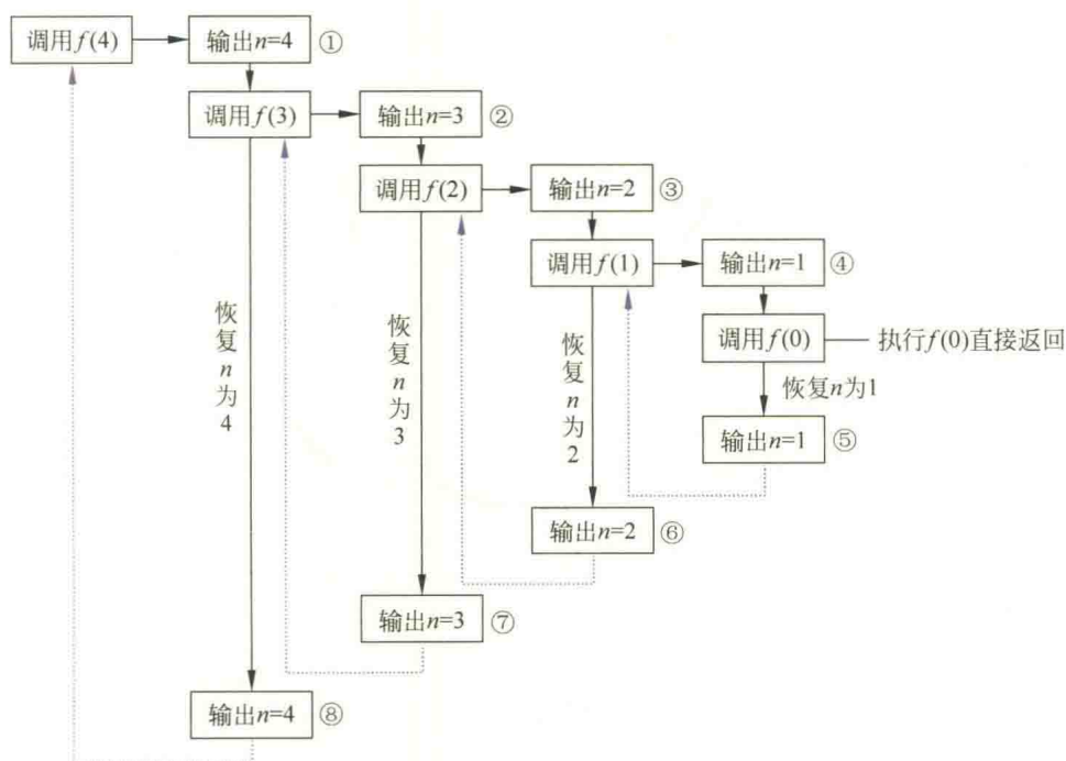
图 2.8 f(4) 的执行过程
