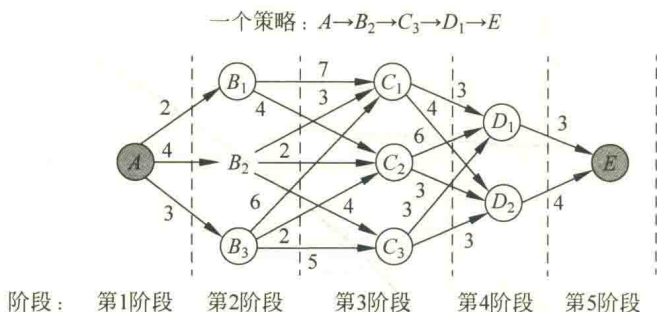
图 8.4 一个多阶段图或多段图
