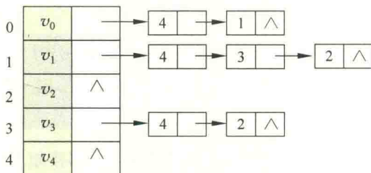
(b) 图的邻接表
