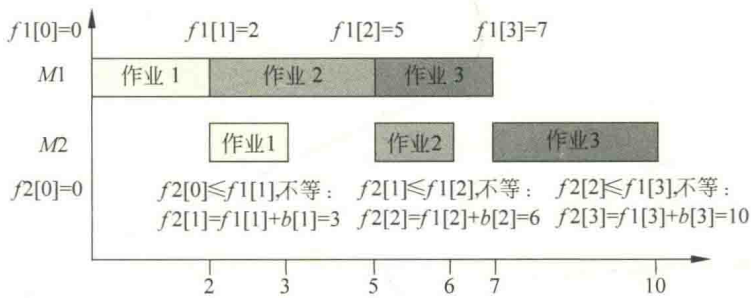
图 5.18 一种调度方案的总时间计算
