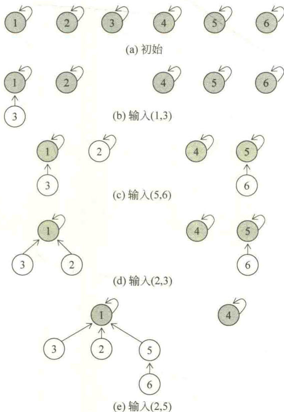
图 9.6 构造并查集的过程
