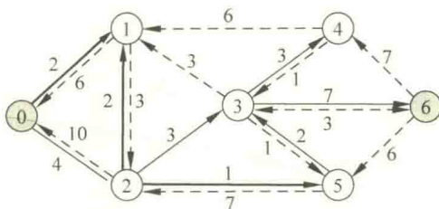
图 9.23 图 9.22 对应的残留网络
