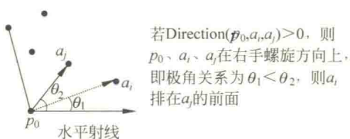
图 10.15 相对于点 p_0 , 点 a_i 排在点 a_j 之前
