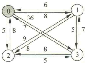
图 9.16 一个 4 城市的图
