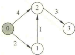
图 9.13 一个带权的有向图
