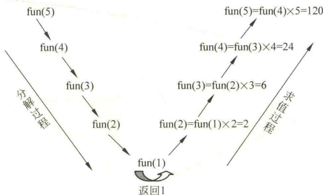
图 2.5 \text{fun}(5) 的求解过程
