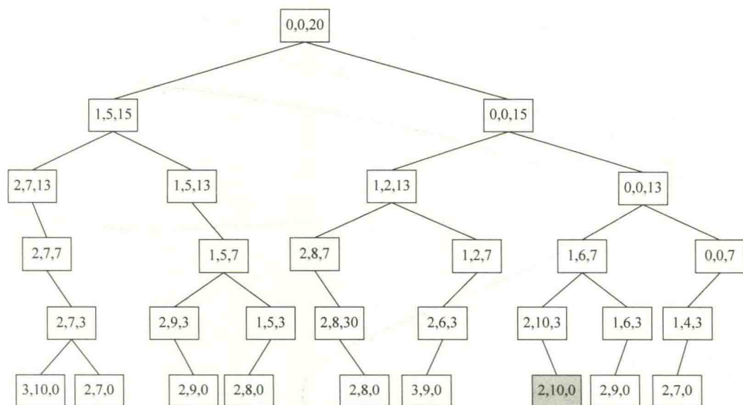
图 5.14 装载问题的解空间树
