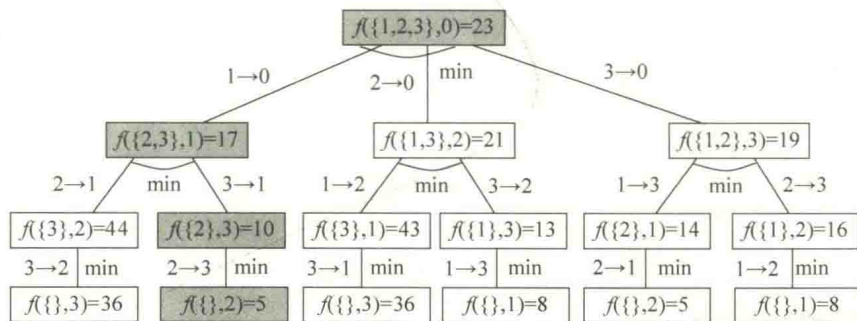
图 9.18 用动态规划法求解 TSP 问题的过程
