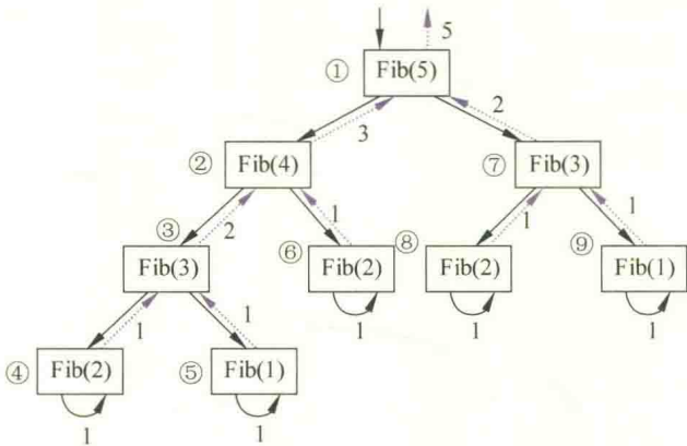
图 2.6 求 Fib(5)的递归树
