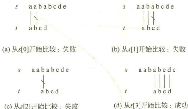
图 4.4 两个字符串的匹配过程
