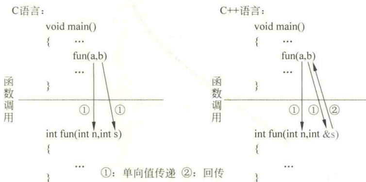
图 1.4 算法中引用型参数的作用
