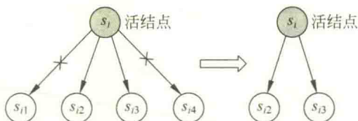
图 6.2 通过限界函数删除一些不必要的子结点
