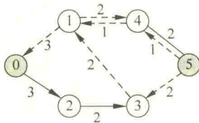
图 9.29 一个残留网络
