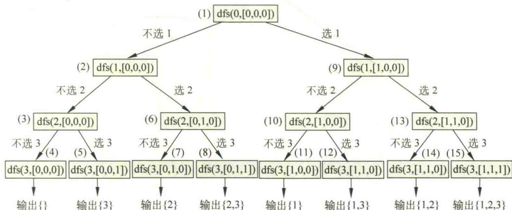
图 5.6 \text{dfs}(0, [0, 0, 0]) 的求解过程
