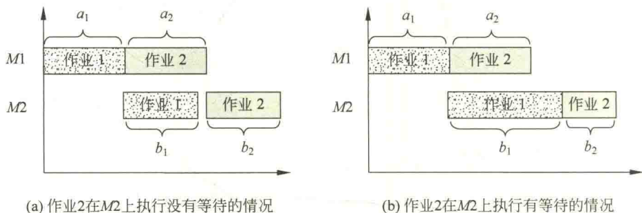
图 7.13 两个作业执行的两种情况
