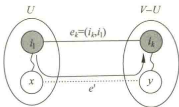
图 9.4 证明普里姆算法的正确性
