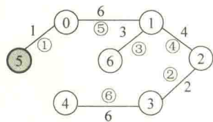
图 9.5 G 的一棵最小生成树
