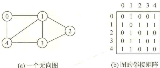
图 4.10 一个无向图及其邻接矩阵表示
