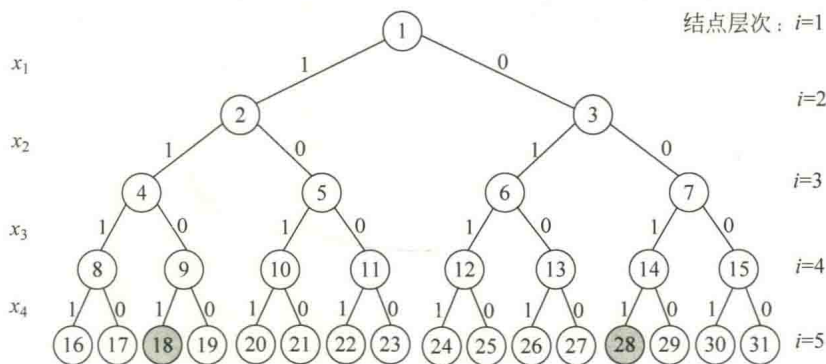
图 5.15 子集和问题的解空间树
