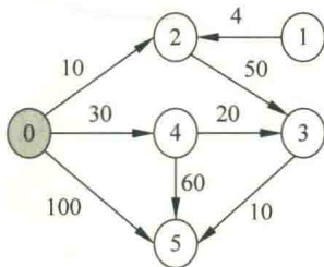
图 6.9 一个带权有向图
