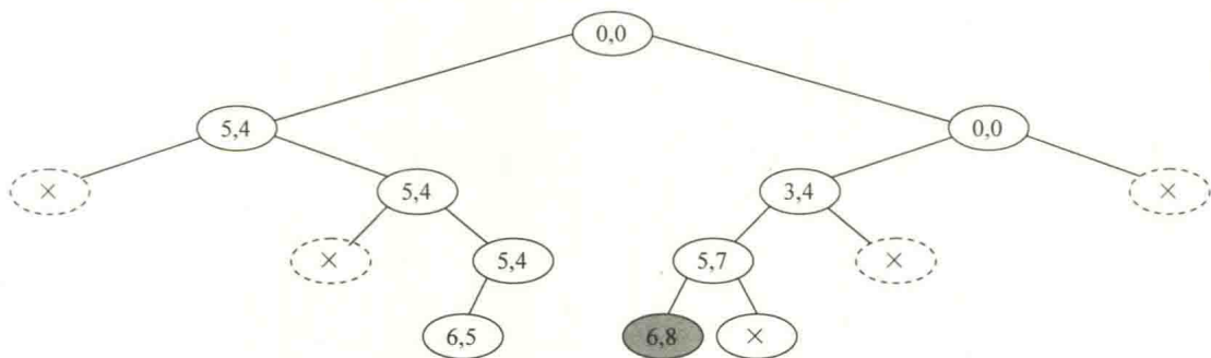
图 5.12 进一步剪枝的解空间树
