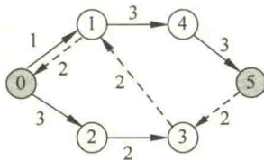
图 9.27 一个残留网络
