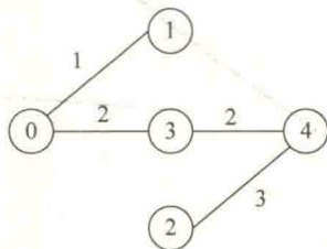
图 12.3 最小生成树 tree
