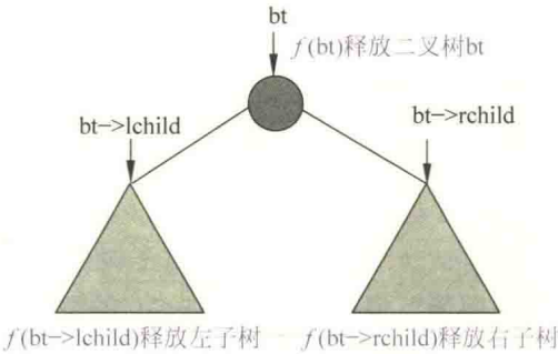
图 2.11 二叉树的释放
