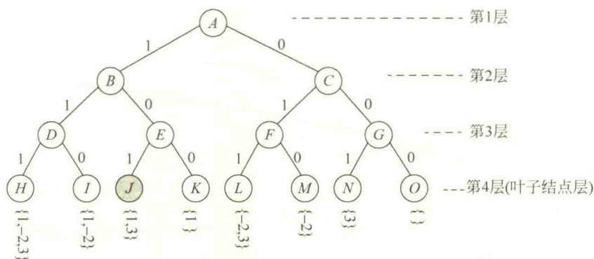
图 5.2 求集合 \{1, -2, 3\} 的幂集的解空间树
