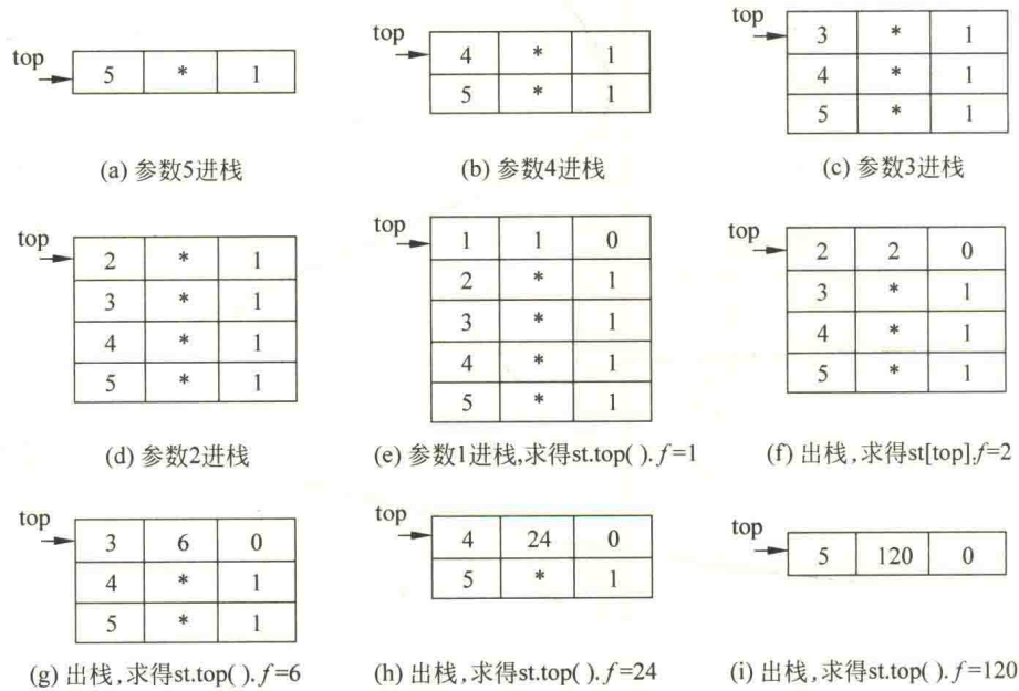
图 2.17 求 fun2(5) 时栈 st 中元素的变化
