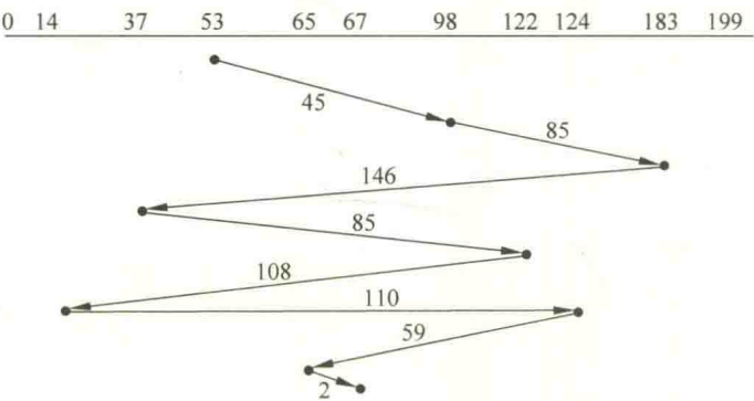
图 7.1 先来先服务算法的磁盘调度过程
