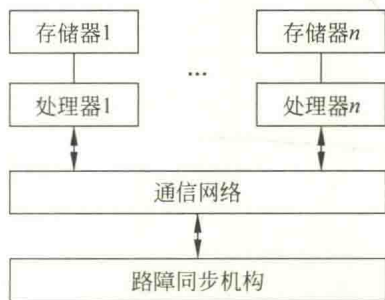
图 3.15 BSP 模型
