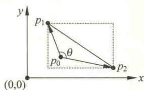
图 10.7 判断点 p 是否在矩形内
