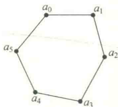
图 10.12 一个凸多边形
