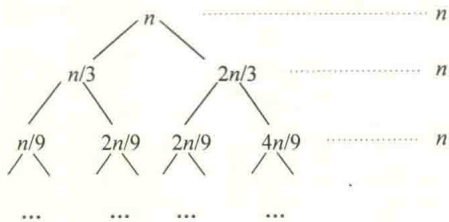
图 2.19 一棵递归树
