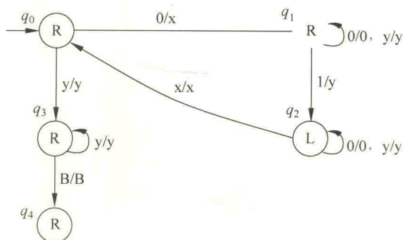
图 11.3 状态转换图
