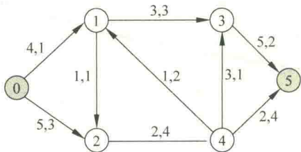
图 9.30 一个网络
