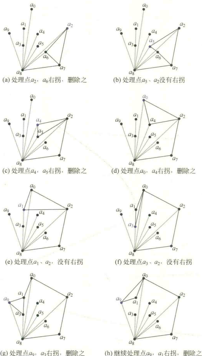
图 10.18 求凸包的过程
