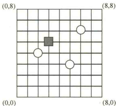
图 7.16 一个街道图
