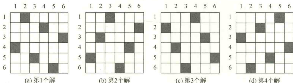
图 2.16 6 皇后解描述
