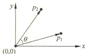
图 10.3 两个向量的点积
