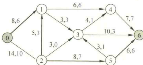
图 9.22 一个网络流
