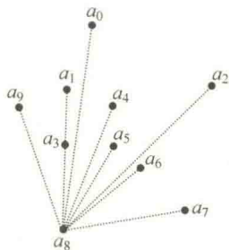
图 10.17 以 a_8 为源点, 按极角从小到大排列
