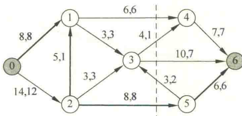
图 9.24 最大网络流
