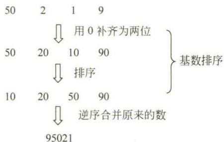
图 7.4 \{50, 2, 1, 9\} 的求解过程
