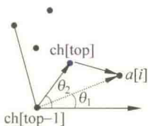
图 10.16 扫描遇到右拐的情况
