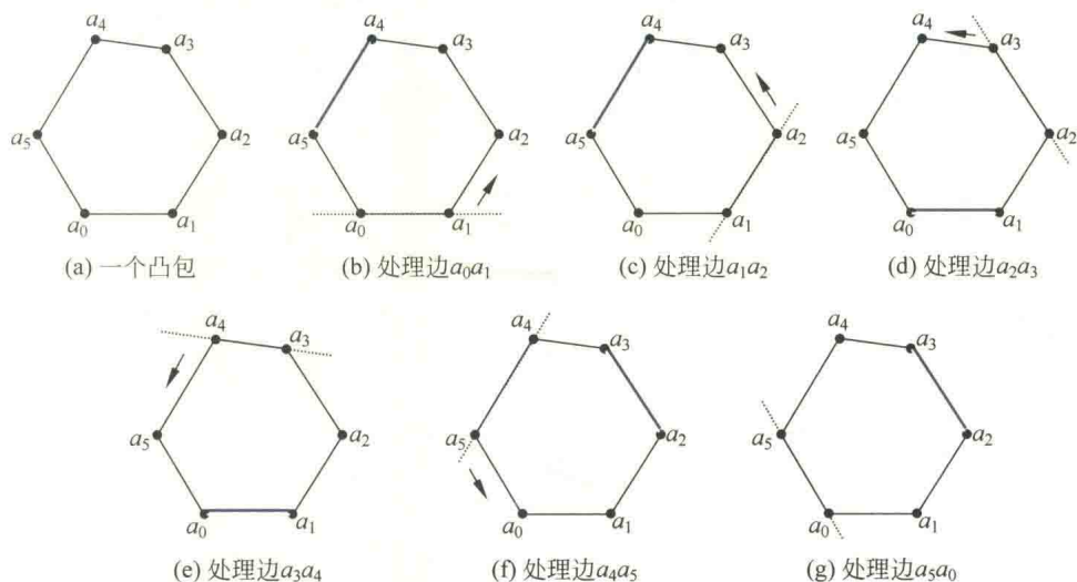
图 10.21 用旋转卡壳算法求最远点对的过程
