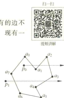
图 10.9 判断点 p 是否在一个多边形内
