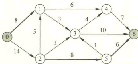
图 9.21 一个网络
