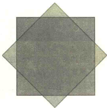
图 10.24 用糍糊涂抹两张剪纸的共同区域
