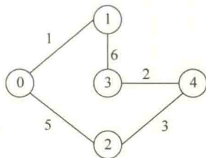
图 12.4 哈密顿回路
