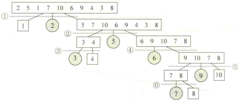
图 3.3 (2,5,1,7,10,6,9,4,3,8)序列的快速排序过程
