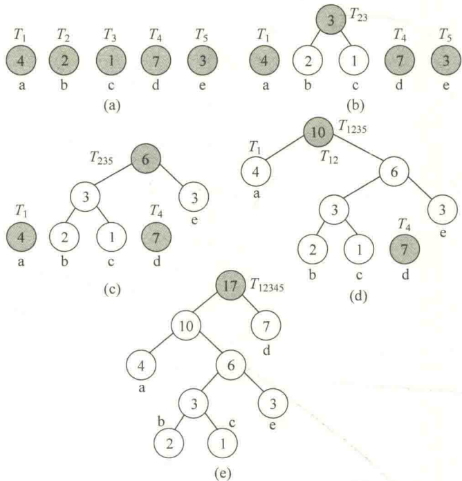
图 7.8 哈夫曼树的构造过程
