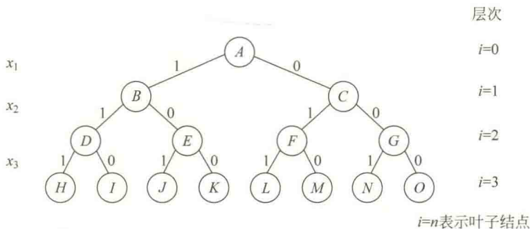
图 6.5 求 0/1 背包问题的解空间树
