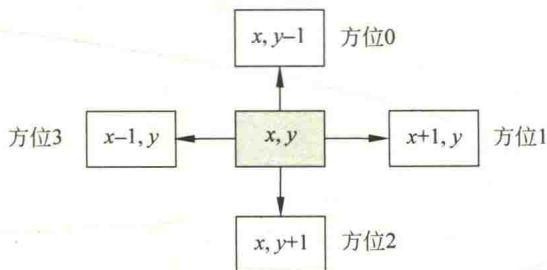
图 4.14 从 (x, y) 方块可以试探的 4 个方位
