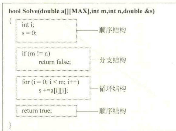
图 1.6 一个算法的组成
