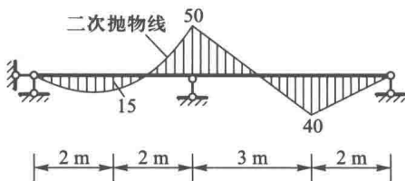
M图(单位 kN·m)
