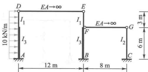
题 7-14 I_1 : I_2 : I_3 = 1 : 2 : 5
