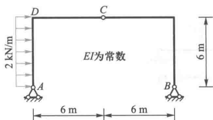
题 6-11 求 \Delta_{Cx} , \Delta_{Cy} , \varphi_D , * 并勾绘变形曲线
