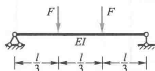
题 6-6 求最大挠度
