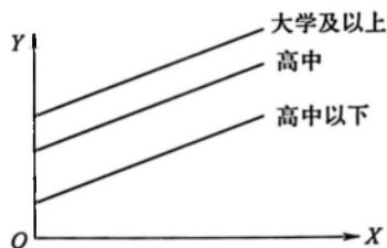
图 3.6.2 不同教育程度人员保健支出示意图
