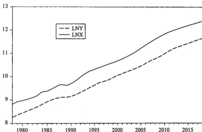
图 5.3.1 \ln Y 与 \ln X 的时间序列
