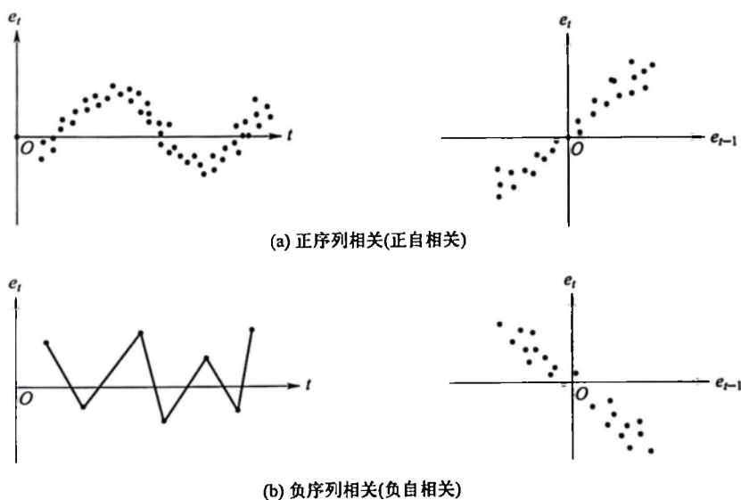
图 5.1.1 残差项序列相关图
