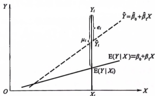
图 2.1.3 总体回归线与样本回归线的基本关系
