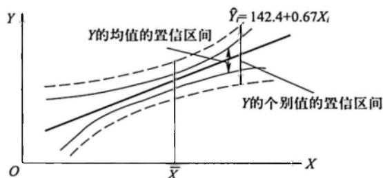
图 2.5.1 Y 的均值与个别值的置信区间
