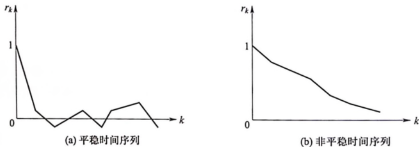
图 5.2.2 平稳时间序列与非平稳时间序列样本相关图
