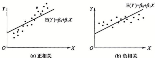
图 4.3.1 随机解释变量与随机干扰项相关图
