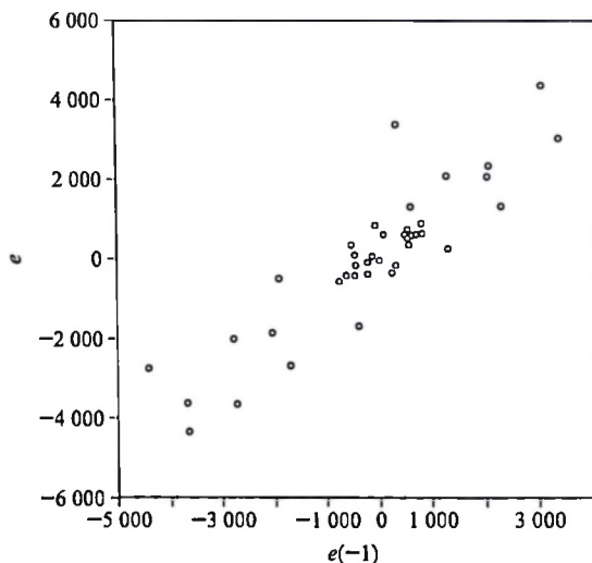
图 5.1.3 残差相关图
