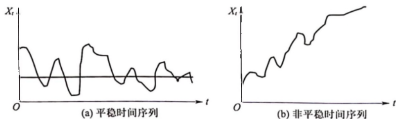
图 5.2.1 平稳时间序列与非平稳时间序列图
