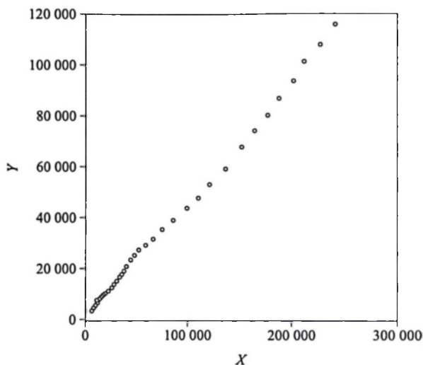
图 5.1.2 X 和 Y 关系图
