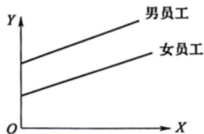
图 3.6.1 男员工平均薪金示意图
