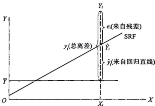
图 2.2.1 离差分解示意图
