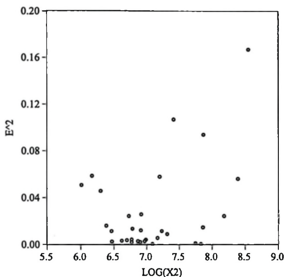
图 4.2.3 异方差性检验图
