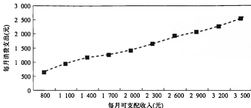
图 2.1.2 家庭可支配收入与消费支出的样本散点图
