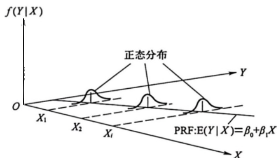
图 2.3.2 总体回归函数与 Y 的条件分布图
