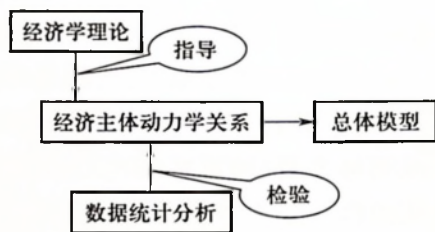
图 7.2.1 理论、数据、动力学关系与总体模型
