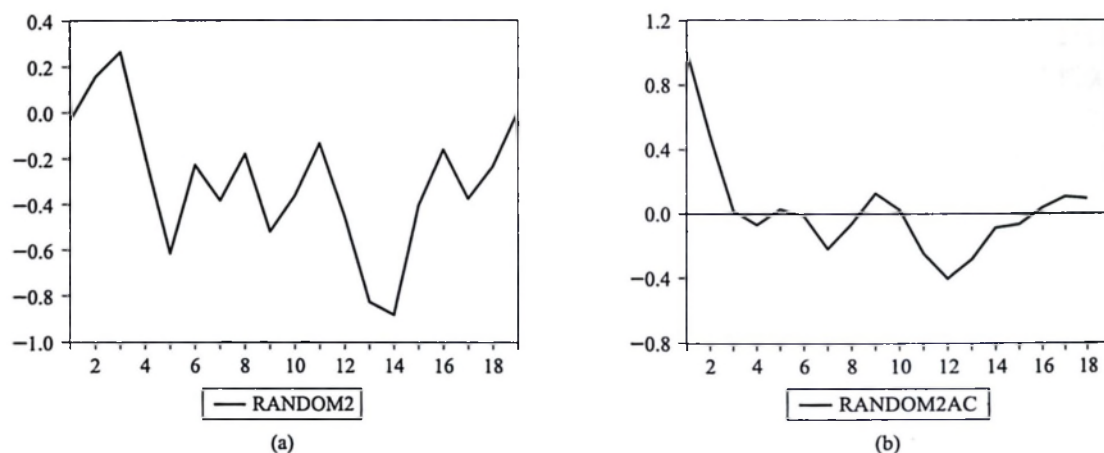
图 5.2.4 随机游走序列 Random2 样本图及其样本自相关系数图
