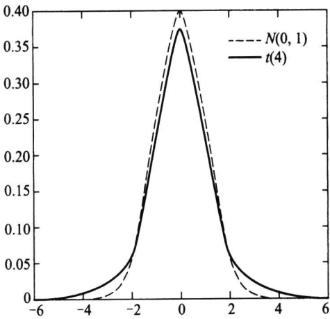
图 5.4.3 t 分布与 N(0, 1) 的密度函数
