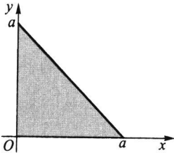
图 1.2.7 线段分成三段 的样本空间 \Omega
