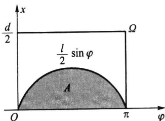
图 1.2.5 比丰投针问题中的 \Omega 和 A
