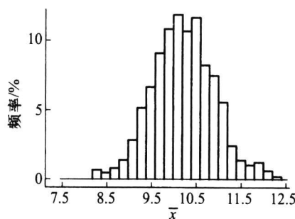
图 5.3.2 500 个样本均值形成的直方图
