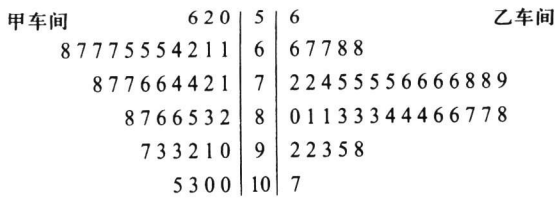
图 5.2.4 两车间产量的背靠背茎叶图
