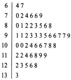
图 5.2.3 测试成绩的茎叶图
