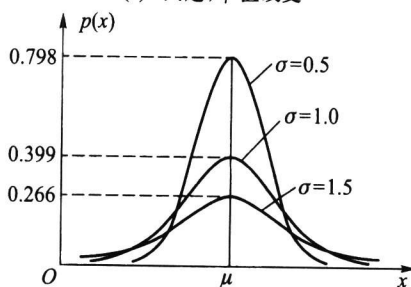
(b) \mu 固定, \sigma 值改变
