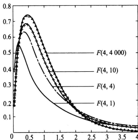
图 5.4.2 F 分布的密度函数
