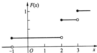
图 2.1.3 离散随机变量的分布函数
