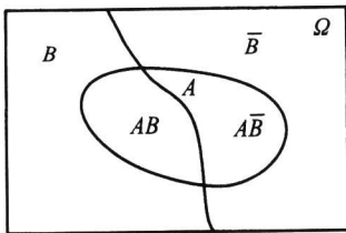
图 1.4.3 用 B 和 \bar{B} 来分割样本空间
