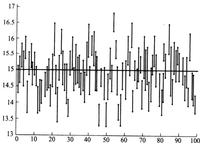
图 6.6.2 \mu 的置信水平为 0.50 的置信区间
