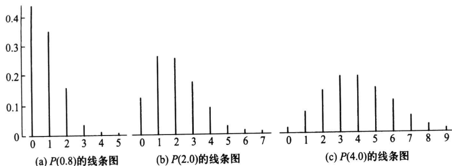
图 2.4.2 泊松分布 P(\lambda) 的线条图
