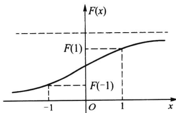
图 2.1.1 柯西分布函数
