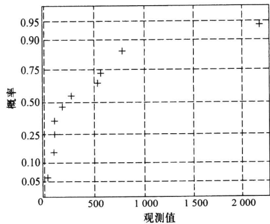
图 7.5.3 例 7.5.2 的正态概率纸
