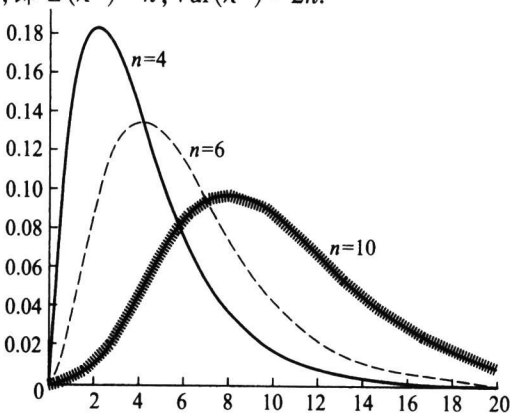
图 5.4.1 \chi^2(n) 分布的密度函数
