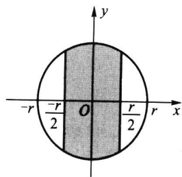
图 3.1.4 p(x, y) 的非零区域
