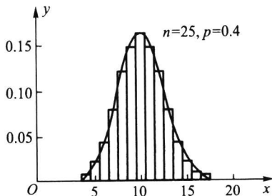
图 4.4.2 二项分布正态近似时的修正
