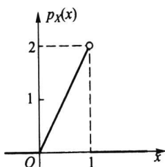
图 3.2.2 X 的边际密度函数 ( Be(2, 1) )
