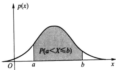
图 2.1.7 连续随机变量场合的概率
