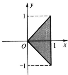
图 3.2.1 p(x, y) 的非零区域
