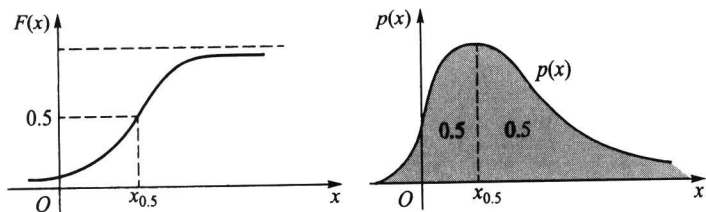
图 2.7.2 连续随机变量的中位数
