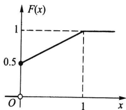
图 2.1.8 既非离散又非连续的分布函数示例
