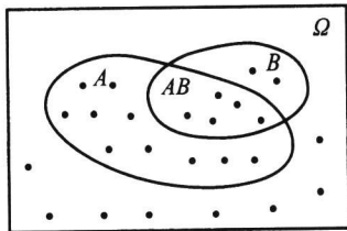
图 1.4.1 例 1.4.2 的维恩图
