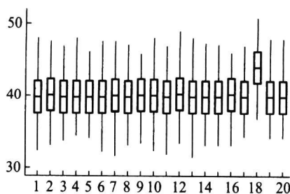
图 5.3.9 20 天生产的某产品的直径的箱线图
