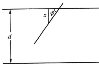
图 1.2.4 比丰投针问题
