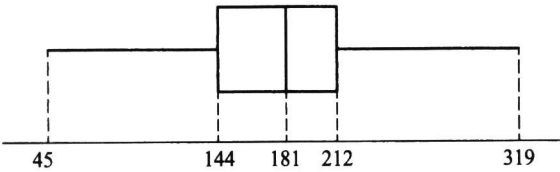
图 5.3.7 月销售量数据的箱线图
