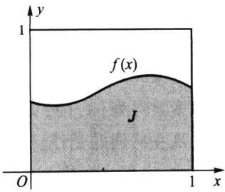
图 4.3.1 随机投点法
