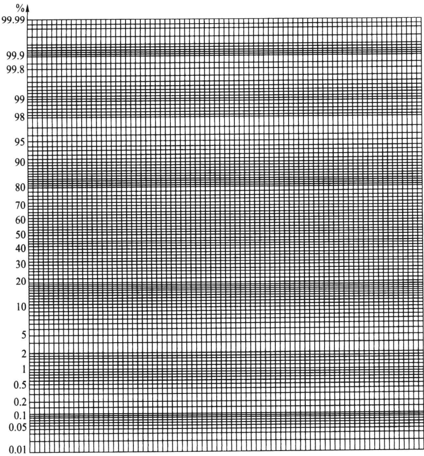
图 7.5.1 正态概率纸
