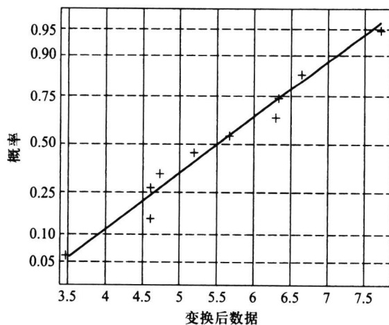
图 7.5.4 变换后数据的正态概率纸
