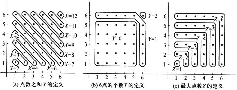
图 2.1.2 同一样本空间上不同随机变量
