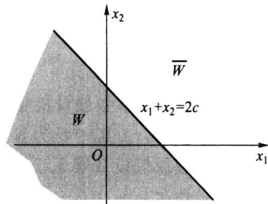
图 7.1.1 拒绝域示意图
