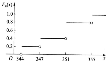
图 5.2.1 经验分布函数
