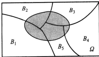
图 1.4.2 样本空间的一个分割( n=5 )
