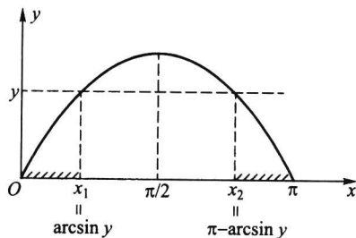
图 2.6.1 y = \sin x 的图形
