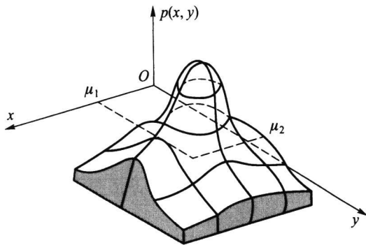
图 3.1.5 二元正态密度函数
