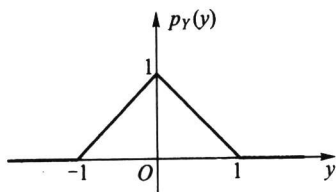
图 3.2.3 Y 的边际密度函数 (三角形分布)
