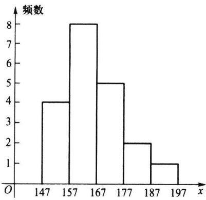
图 5.2.2 例 5.2.2 的频数直方图
