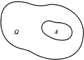
图 1.2.2 几何概率
