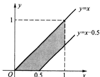
图 3.4.2 例 3.4.10 中 p(x, y) 的非零区域
