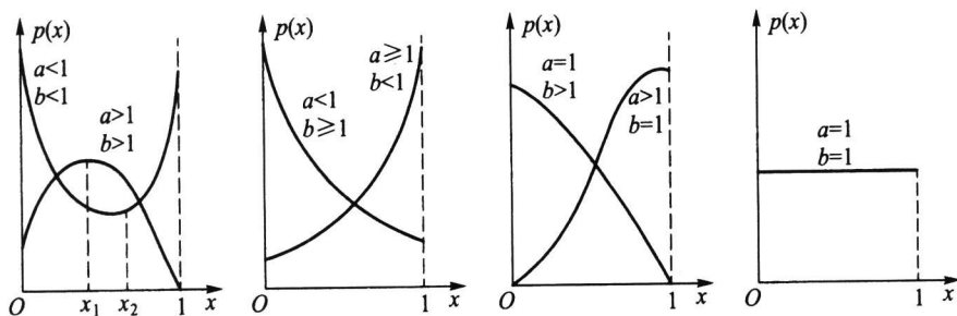
图 2.5.7 贝塔分布密度函数曲线
