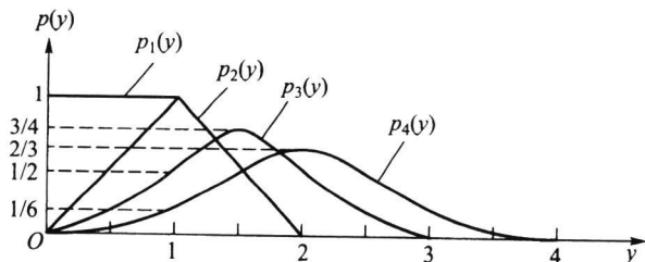
图 4.4.1 均匀分布的卷积
