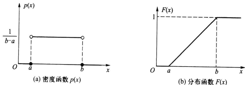
图 2.5.3 (a, b) 上的均匀分布
