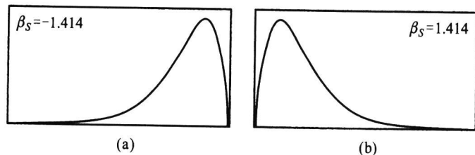
图 2.7.3 两个密度函数, (a) 为左偏, (b) 为右偏
