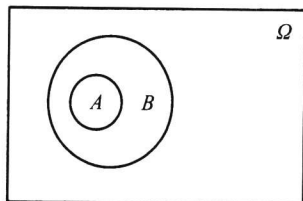
图 1.1.2 A \subset B
