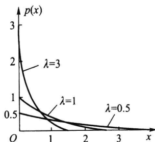
图 2.5.4 参数为 \lambda 的指数分布密度函数
