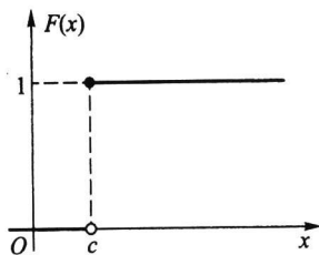
图 2.1.4 单点分布函数
