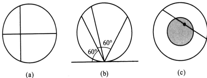
图 1.2.9 贝特朗奇论的三种解法
