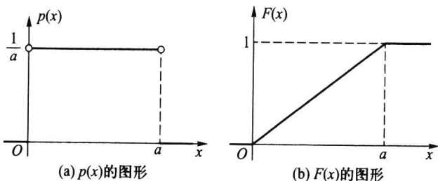
图 2.1.6 (0, a) 上的均匀分布
