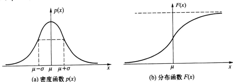
图 2.5.1 正态分布
