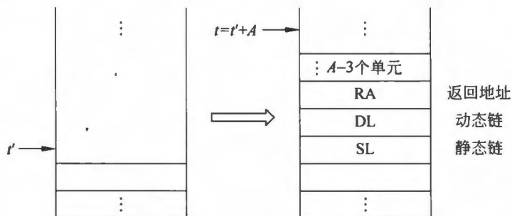
图 9.20 指令 INT 0 A 执行前后示意
