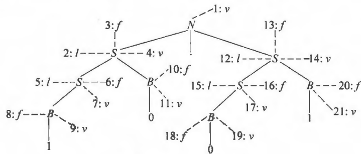
图 7.4 依赖图的结点
