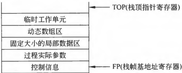
图 9.6 典型的过程活动记录结构
