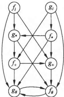
图 5.9 优先函数关系图
