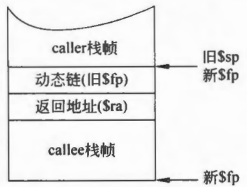
图 11.8 函数调用栈帧结构
