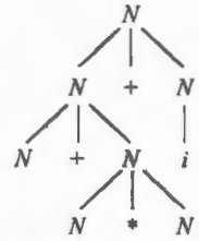
图 5.7 算符优先分析时语法树的框架
