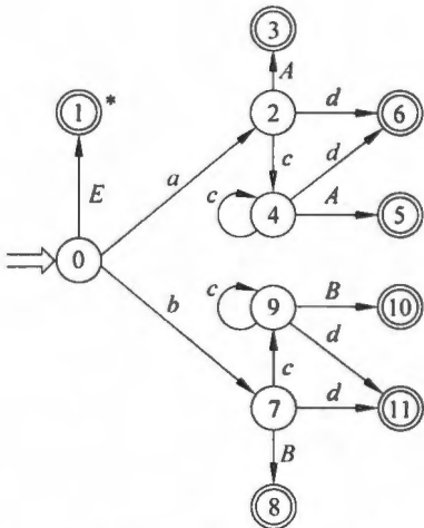
图 6.6 识别可归前缀的确定有限自动机
