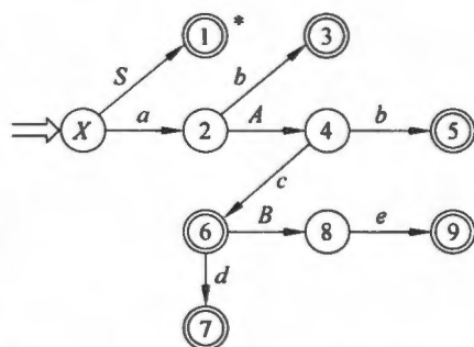
图 6.4 识别活前缀的确定有限自动机
