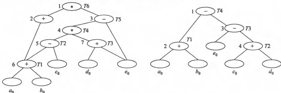
图 10.21 对 DAG 图内部结点进行标记
