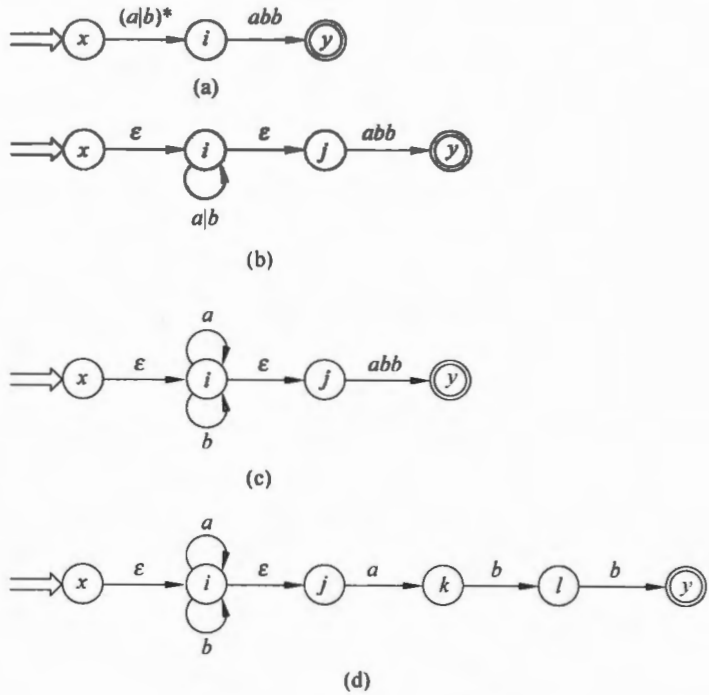
图 3.12 从正规式 r 构造 NFA
