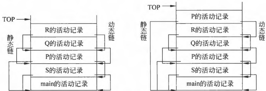
图 9.14 动态链与静态链
