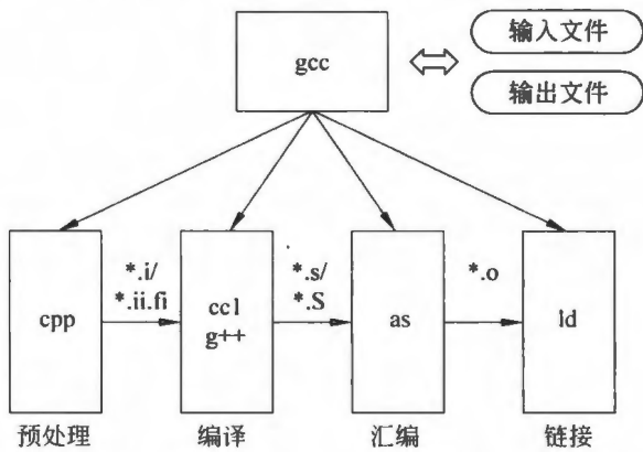
图 12.1 GCC 工作过程示意图
