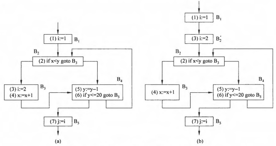
图 10.14 含循环不变量但不符合外提条件的流图
