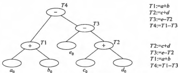
图 10.19 从基本块 DAG 图生成的等价但次序不同的 TAC 语句序列
