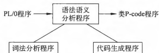
图 1.20 PL/0 编译程序组织结构
