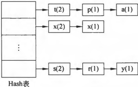
图 8.2 单符号表组织
