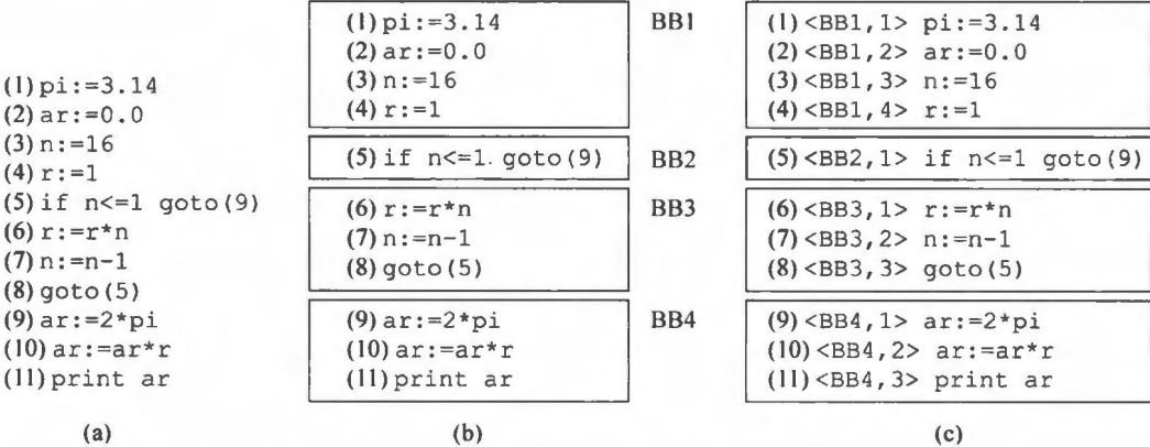
图 10.1 计算圆的周长的三地址中间代码和基本块
