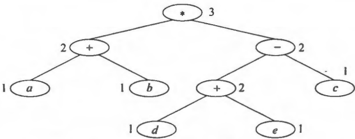
图 10.22 用 Ershov 数标记表达式树结点
