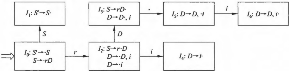
图 6.9 识别文法 G' 活前缀的 DFA
