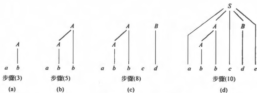
图 5.1 自底向上构造语法树的过程
