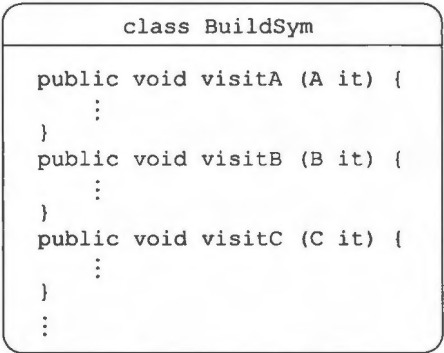
图 8.13 建立符号表的类 BuildSym
