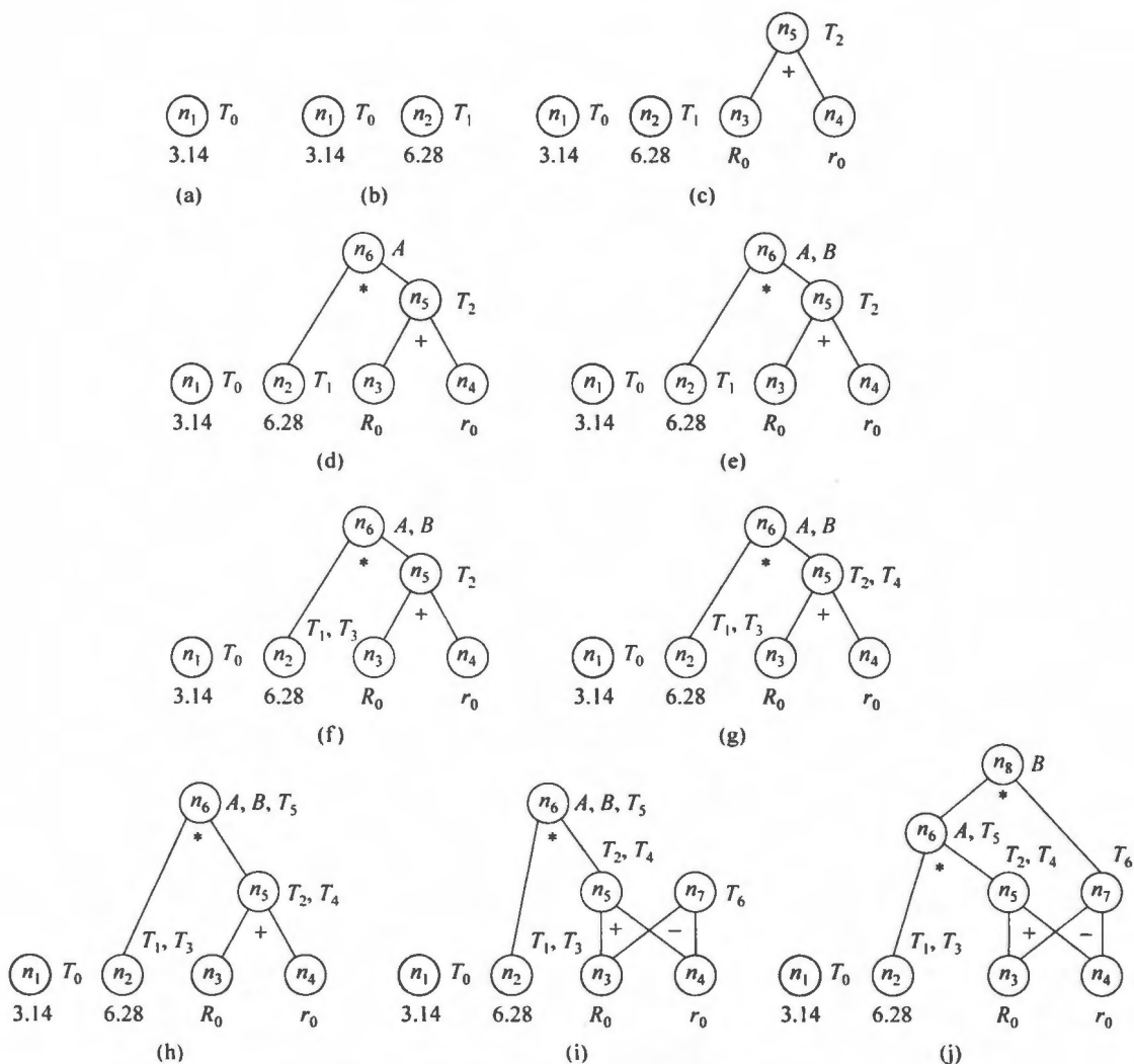
图 10.11 由 TAC 语句序列构造 DAG 图
