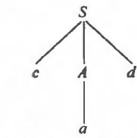
图 2.6 cad 的语法树
