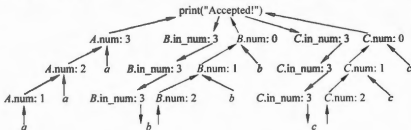
图 7.2 继承属性的计算：自顶向下传递信息
