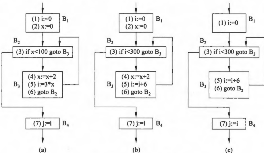
图 10.15 归纳变量的删除
