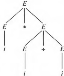
图 2.3 推导 2 的语法树
