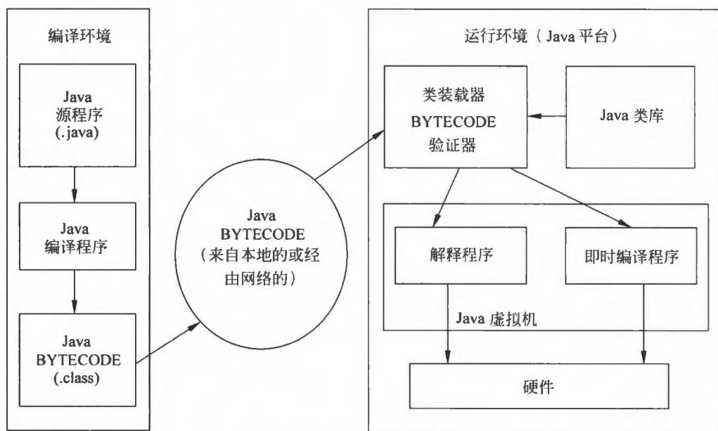
图 1.15 Java 语言环境
