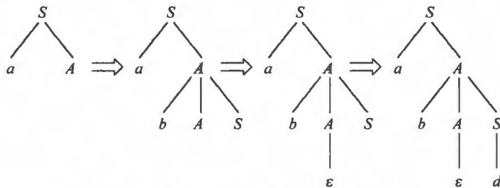
图 4.3 确定的自顶向下语法分析树(三)
