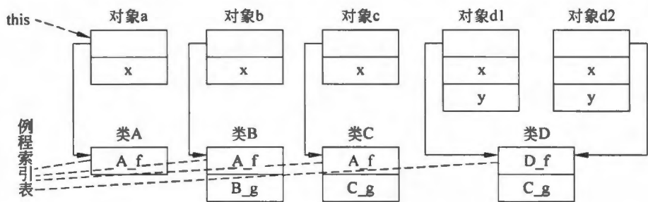
图 9.23 对象存储示例
