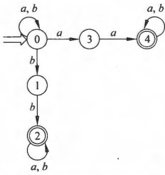
图 3.5 NFA M 的状态图
