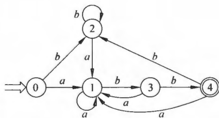
图 3.8 DFA M 的状态图
