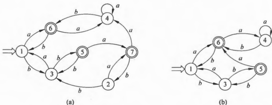
图 3.10 DFA M 和 DFA M'
