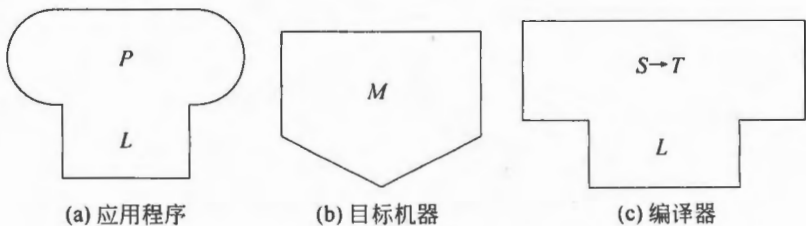
图 12.6 不同类型的 T 形图
