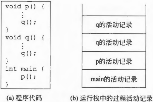
图 9.4 活动记录在运行栈上的分配
