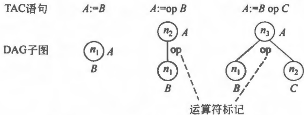
图 10.10 三类 TAC 语句对应的 DAG 子图
