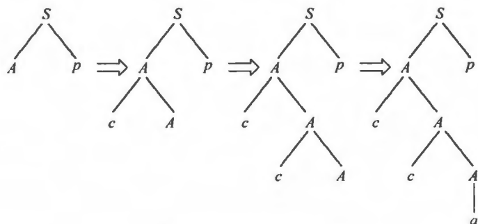
图 4.2 确定的自顶向下语法分析树(二)
