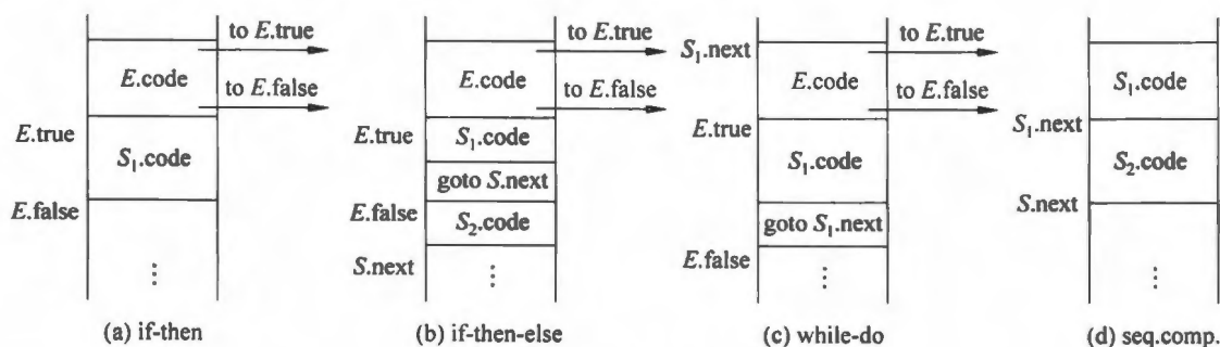
图 8.10 控制语句的翻译
