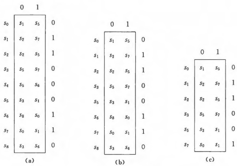
图 3.9 消除多余状态
