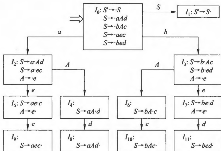
图 6.11 LR(0)识别 G' 的活前缀的 DFA
