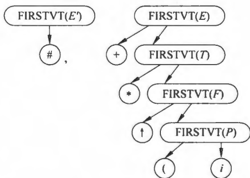
图 5.5 关系图形法计算 FIRSTVT 集合
