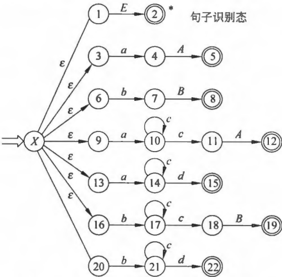
图 6.5 识别可归前缀的不确定有限自动机
