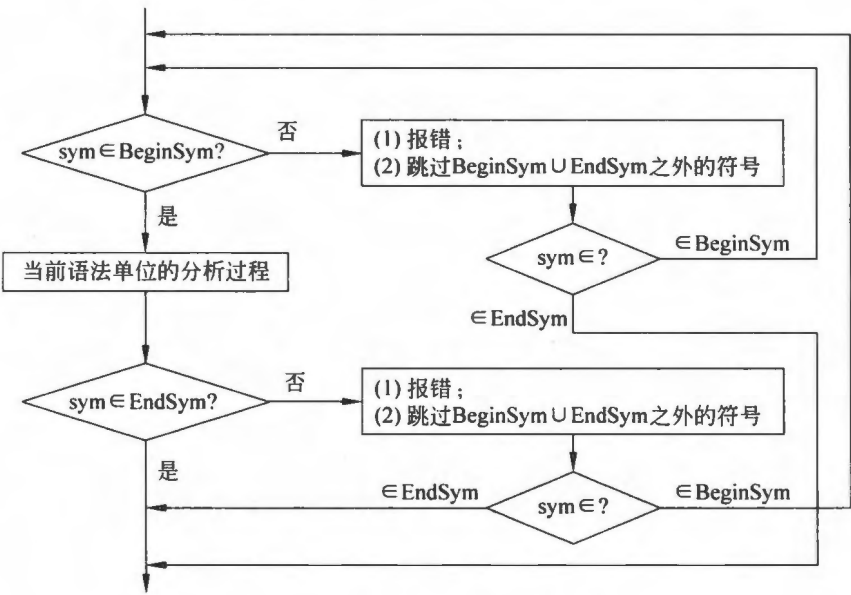
图 4.12 短语层恢复可采取的流程
