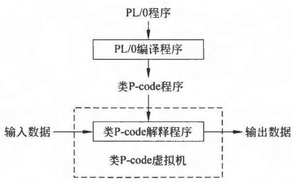
图 1.16 PL/0 语言编译系统
