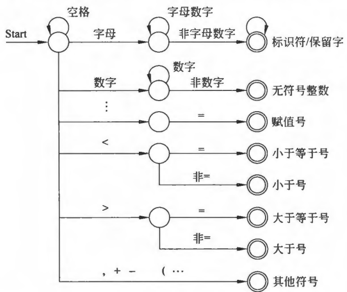
图 3.2 PL/0 词法规则状态转换图
