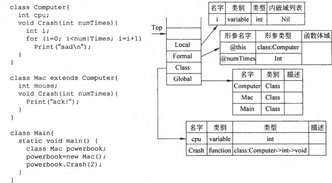
图 11.3 Decaf 编译器作用域栈示意
