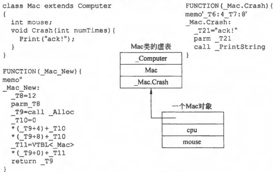
图 11.6 New 函数和成员函数的另一个例子
