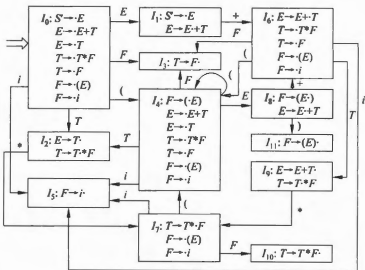
图 6.10 识别表达式文法活前缀的 DFA
