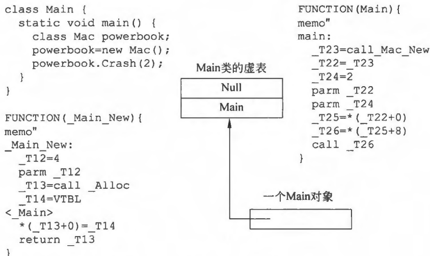
图 11.7 类 Main 及 static main 函数
