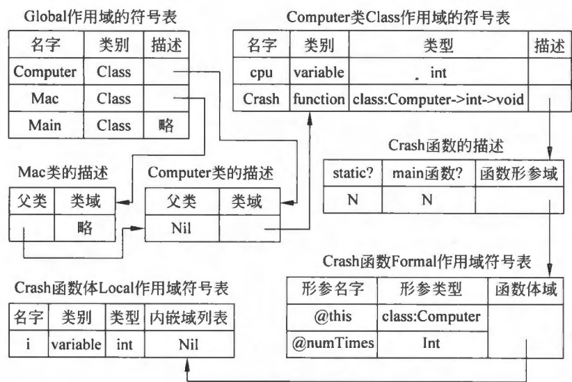
图 11.2 Decaf 编译器符号表结构示意图
