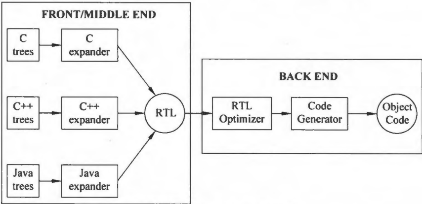
图 12.2 GCC 3. X 结构示意图
