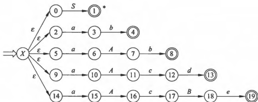
图 6.3 识别活前缀的不确定有限自动机
