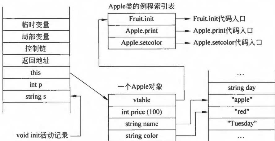
图 9.24 例程的动态绑定
