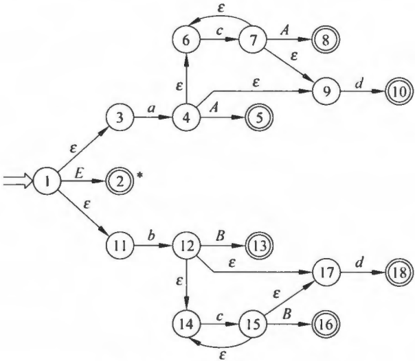
图 6.7 识别活前缀的 NFA
