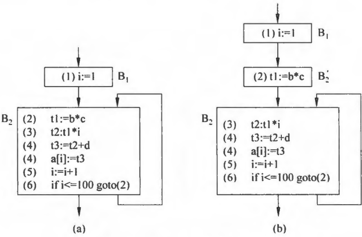
图 10.13 循环不变量代码外提
