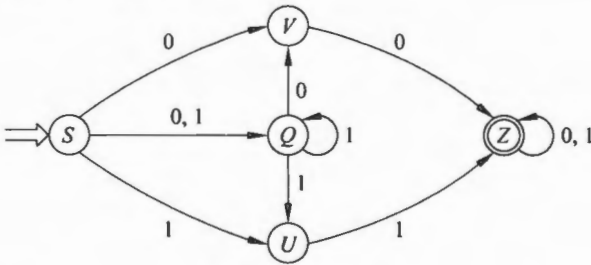
图 3.16 NFA
