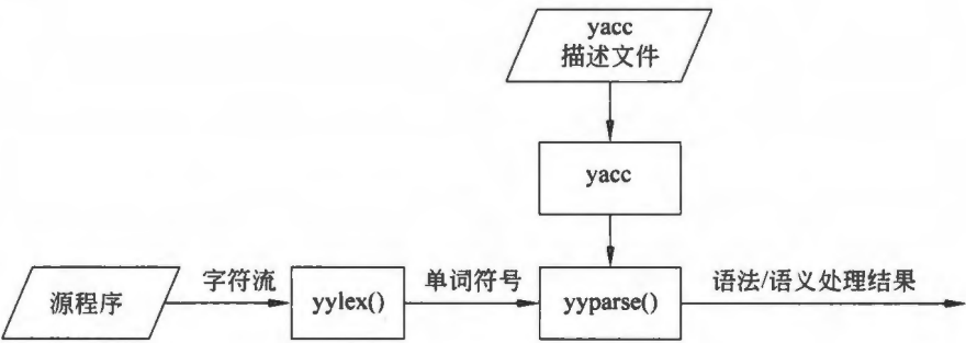
图 7.18 yacc 简介
