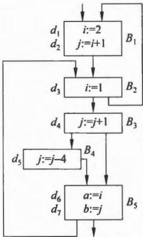
图 10.4 某个流图
