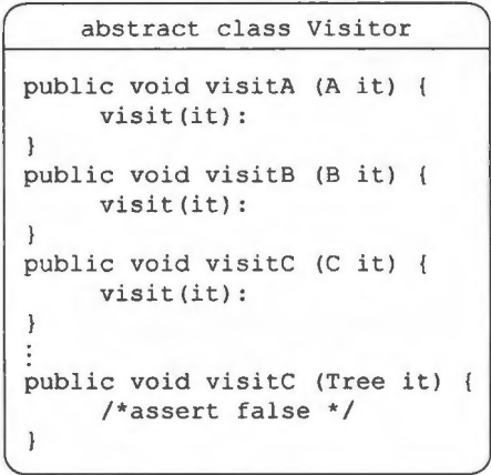
图 8.14 抽象类 Visitor
