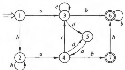
图 3.18 DFA
