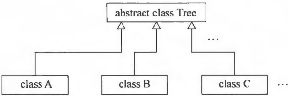
图 8.12 AST 结点类都是抽象类 Tree 的子类
