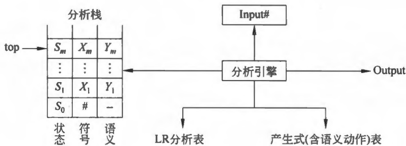
图 7.8 附加语义栈的 LR 分析模型
