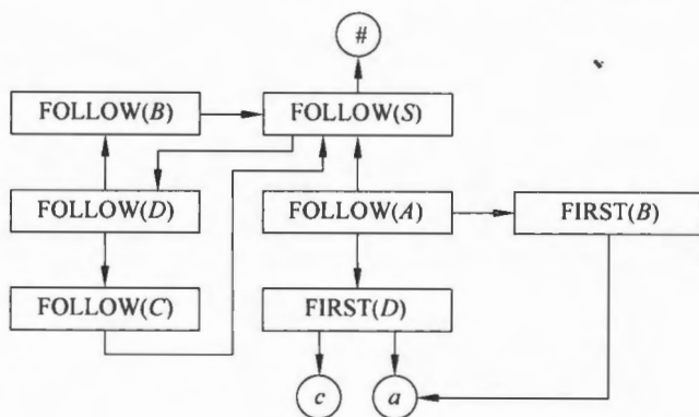
图 4.5 计算 FOLLOW 集的关系图
