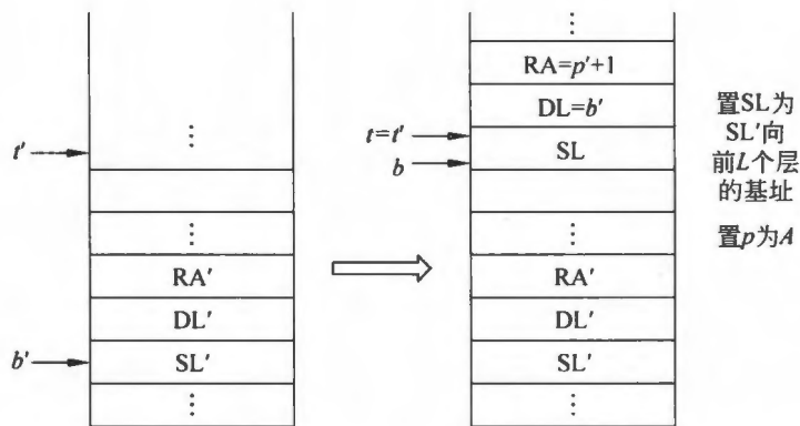
图 9.19 指令 CAL L A 执行前后示意
