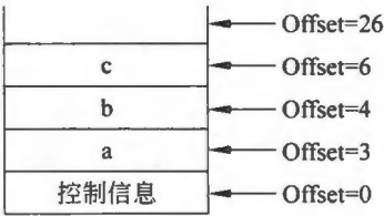
图 9.7 不含动态数据区的过程活动记录
