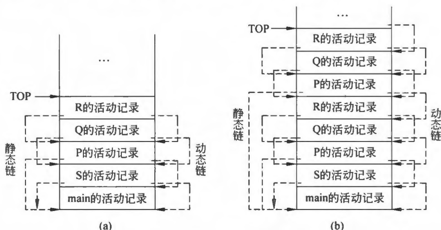
图 9.18 PL/0 程序运行栈的变化
