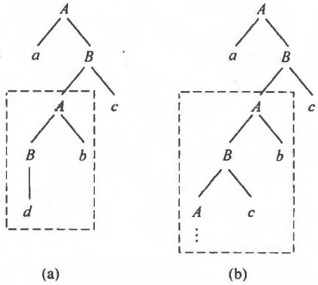
图 4.7 含间接左递归文法的语法分析树
