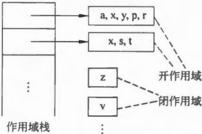
图 8.3 多符号表组织
