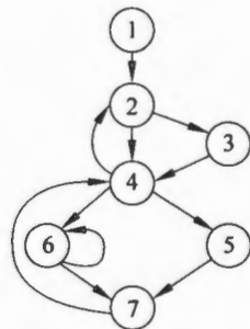
图 10.3 某程序的流图结构
