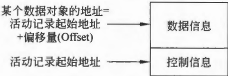
图 9.5 活动记录中数据对象的寻址
