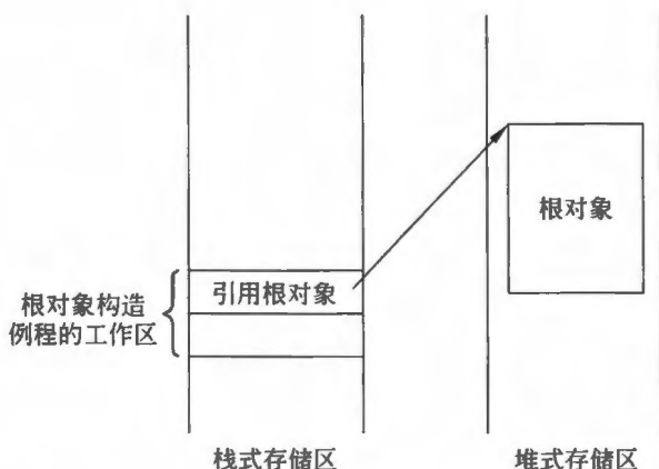
图 9.22 创建根对象时的存储结构
