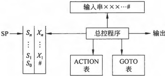
图 6.1 LR 分析器工作过程示意图
