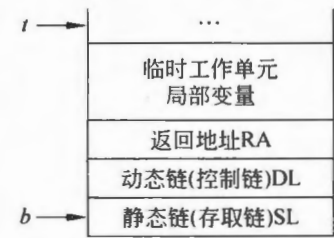
图 9.17 PL/0 的过程活动记录
