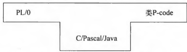
图 1.17 PL/0 编译程序 T 形图
