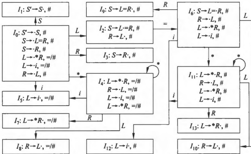
图 6.13 LR(1)项目集及转换函数
