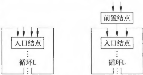
图 10.12 为代码外提建立前置结点
