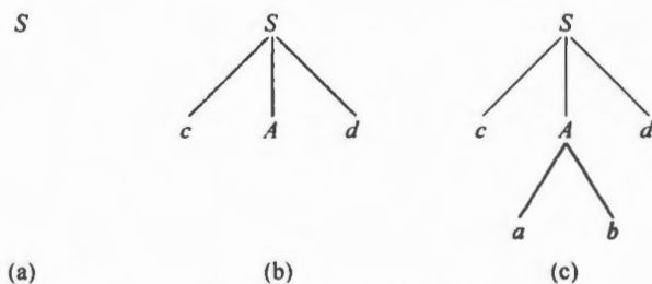
图 2.4 自上而下的分析步骤
