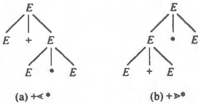
图 5.4 二义性文法的语法树
