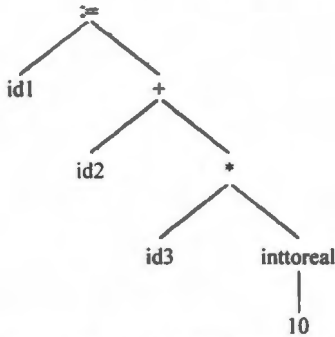
图 1.6 插入语义处理结点的树
