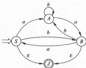
图 3.13 与 G[S] 等价的 NFA M
