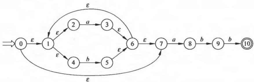
图 3.6 NFA N 的状态图
