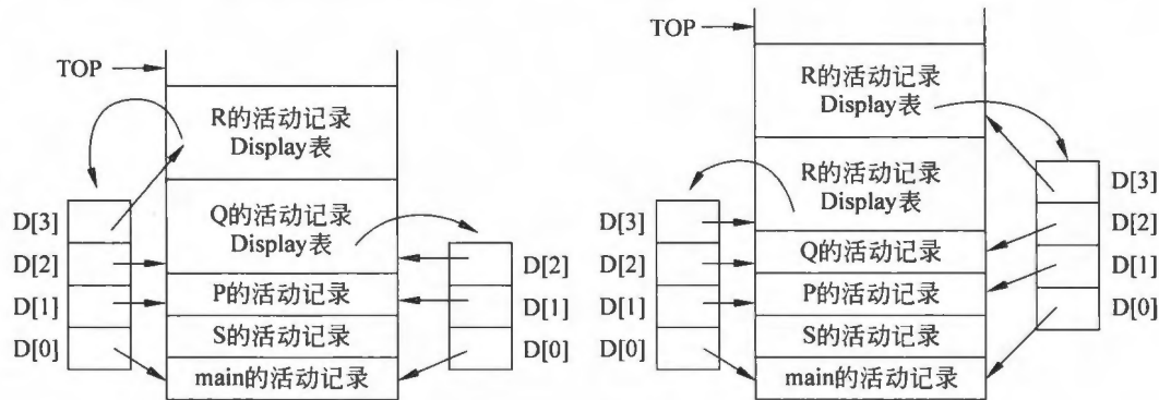
图 9.11 Display 表的维护(一)
