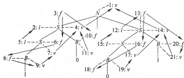
图 7.5 依赖图的有向边
