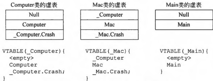
图 11.4 Decaf 编译器中 Vtable 结构的示意
