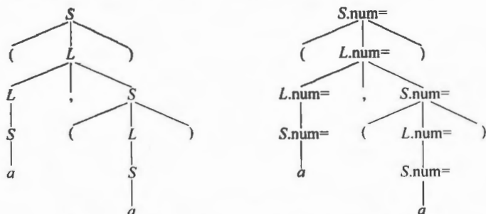
图 7.19 题 2 的语法分析树和带标注语法树
