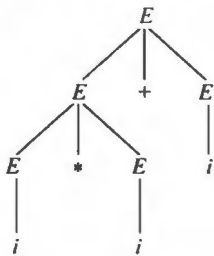
图 2.2 推导 1 的语法树
