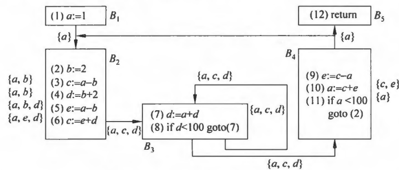
图 10.23 定值点之后的活跃变量信息
