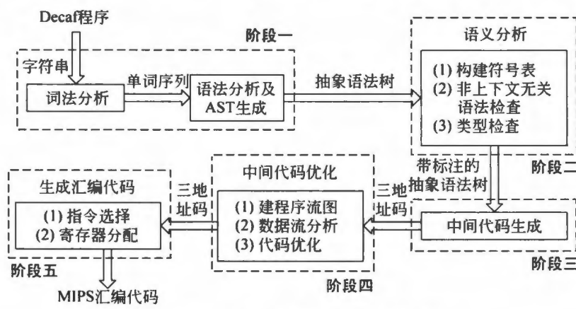
图 11.1 Decaf 编译器实验的总体结构
