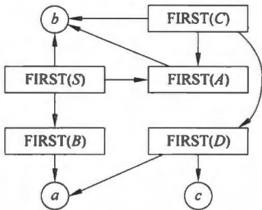
图 4.4 计算 FIRST 集的关系图
