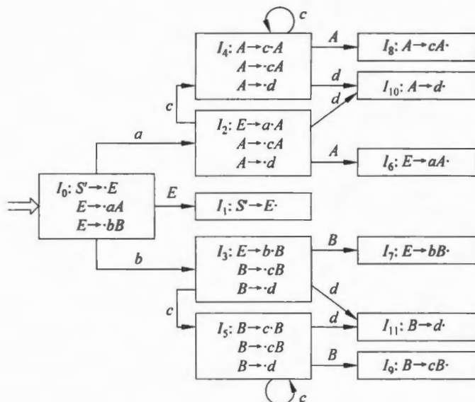
图 6.8 识别活前缀的 DFA
