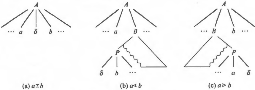
图 5.3 由语法树结构决定优先级
