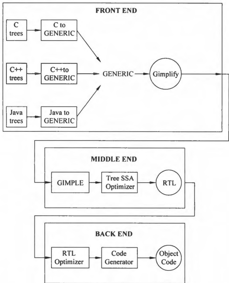
图 12.3 GCC 4.X 结构示意图
