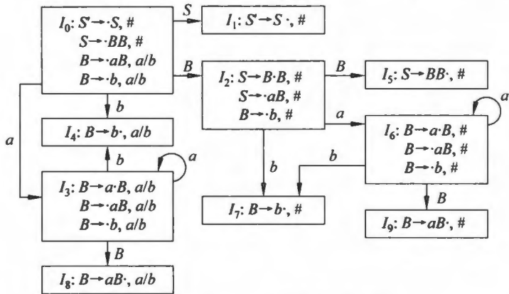
图 6.12 LR(1)项目集和转换函数
