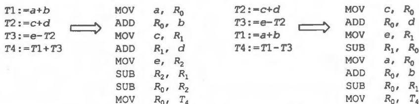
图 10.20 两段 TAC 代码对应的目标代码
