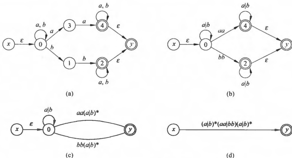
图 3.11 从 NFA M 构造正规式 r
