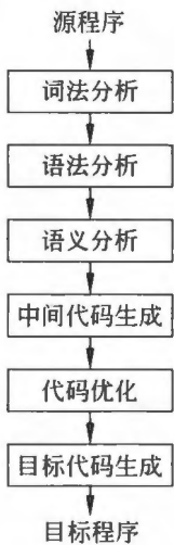
图 1.3 编译的各个阶段
