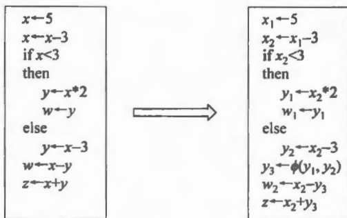
图 8.9 静态单赋值形式
