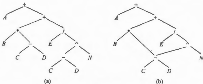
图 8.7 抽象语法树和有向无圈图
