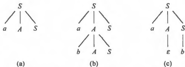
图 4.9 不确定的自顶向下语法分析树(二)
