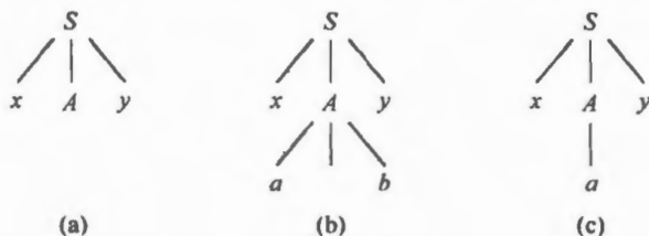
图 4.8 不确定的自顶向下语法分析树(一)
