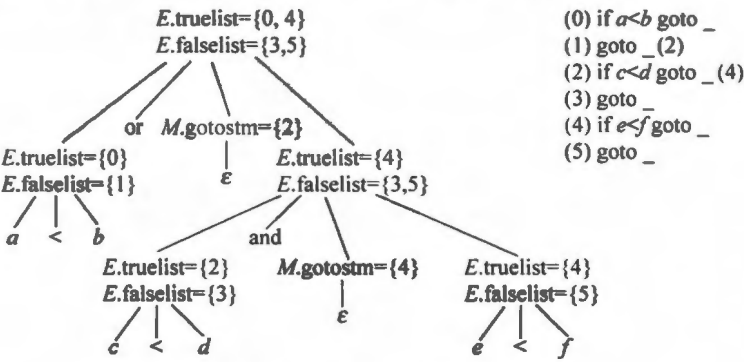
图 8.11 拉链与代码回填
