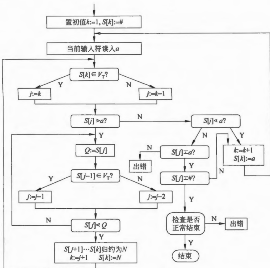
图 5.8 算符优先分析归约过程流程图
