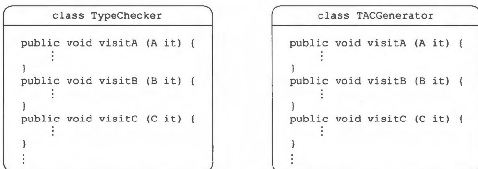
图 8.18 完成静态语义检查的类 TypeChecker 和实现 TAC 生成的类 TACGenerator
