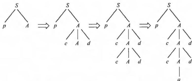
图 4.1 确定的自顶向下语法分析树(一)
