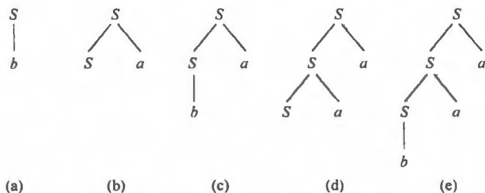
图 4.10 不确定的自顶向下语法分析树(三)
