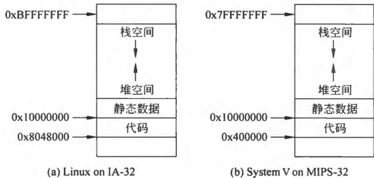
图 9.2 不同体系结构和操作系统的用户程序虚拟存储空间示例
