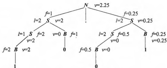
图 7.7 带标注语法分析树
