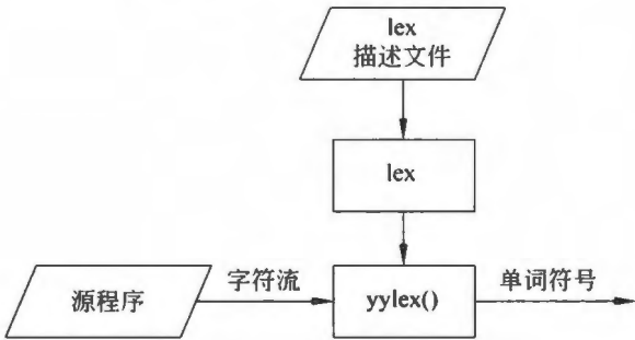
图 3.15 lex 简介
