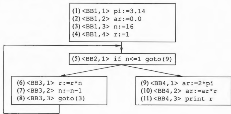
图 10.2 流图的例子
