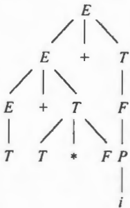
图 5.6 句型 T+T*F+i
