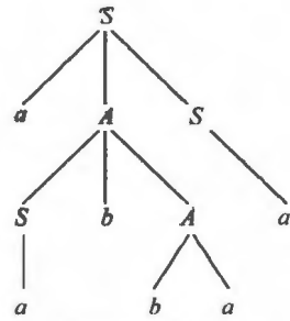
图 2.1 推导树
