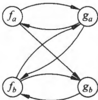
图 5.10 优先关系图
