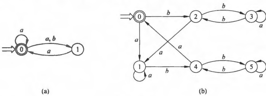
图 3.17 NFA
