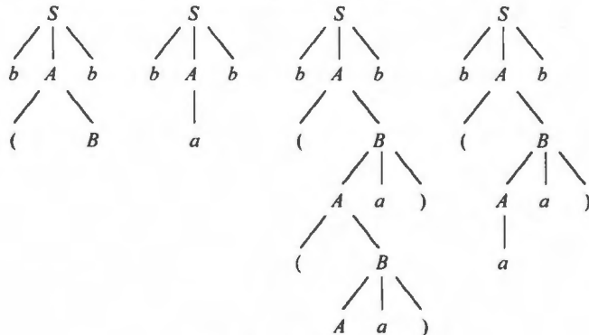
图 5.2 语法树结构
