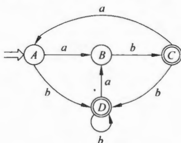
图 3.14 NFA
