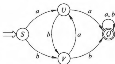
图 3.3 状态图表示
