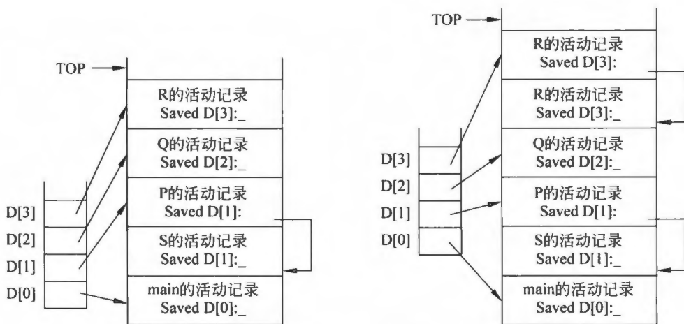
图 9.12 Display 表的维护(二)
