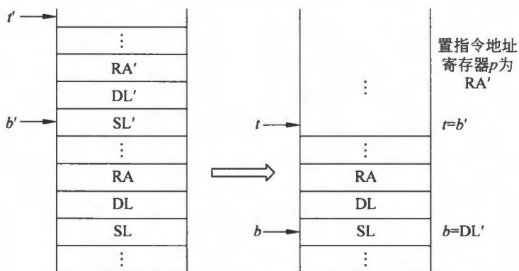
图 9.21 指令 OPR 0 0 执行前后示意
