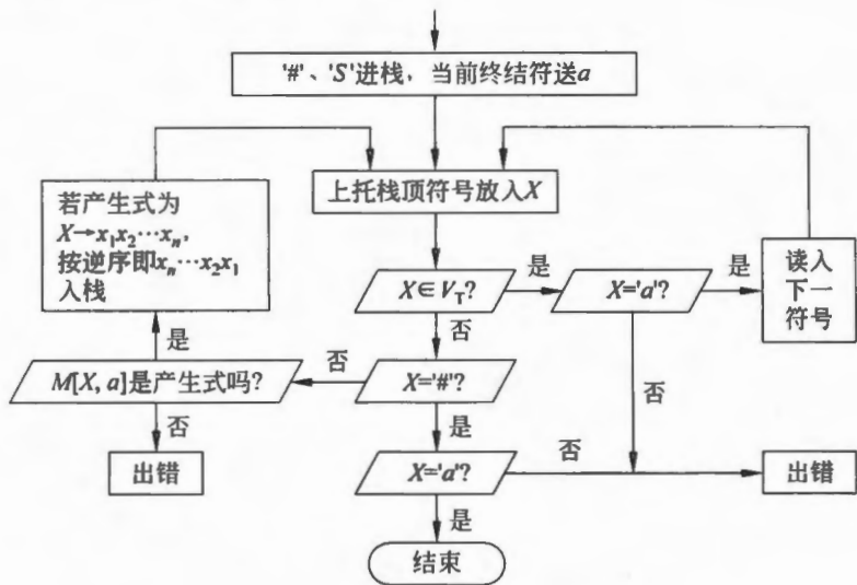
图 4.11 预测分析程序的流程图
