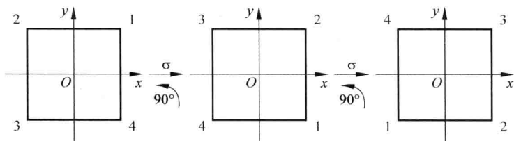
图 8.2 例 8.1.11 图
