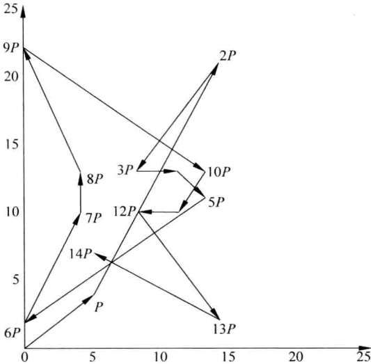
图 14.2 例 14.2.7 图
