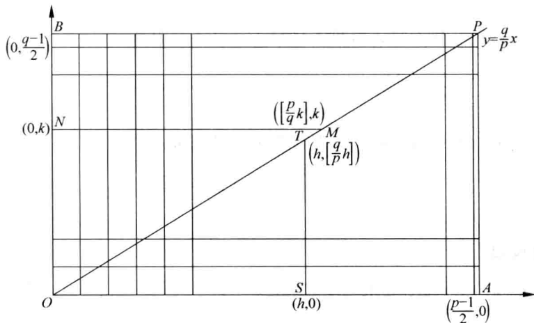
图 4.1 定理 4.4.1 证明
