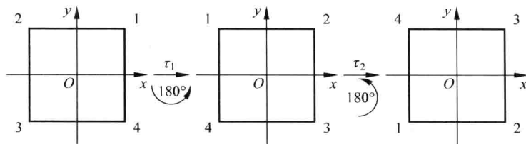
图 8.3 例 8.1.12 图
