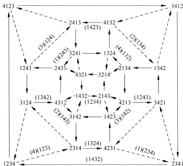
图 9.2 S_4 的 Cayley 图
