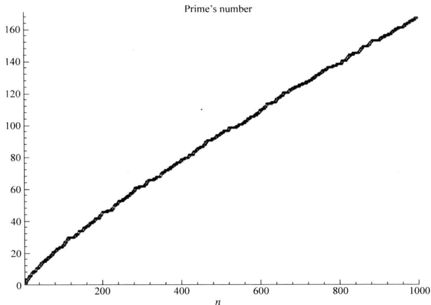
图 1.1 \pi(x) 的图形
