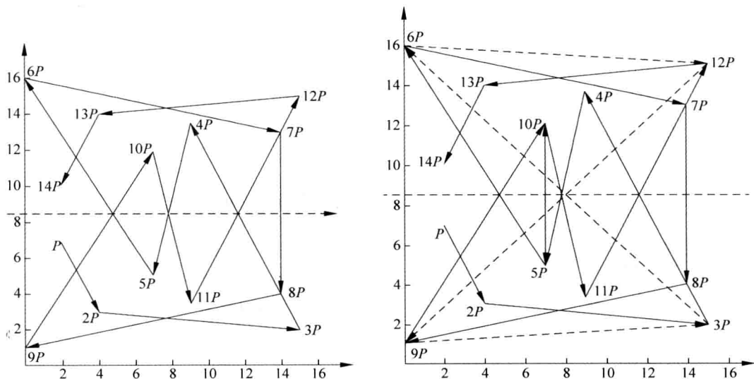
图 14.1 例 14.2.6 图
