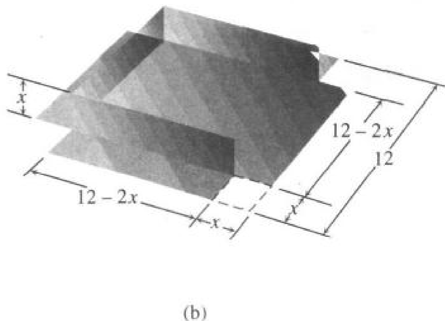
图 3.43 由四角切去正方形的马口铁制成的无盖方盒子.(例 1)
