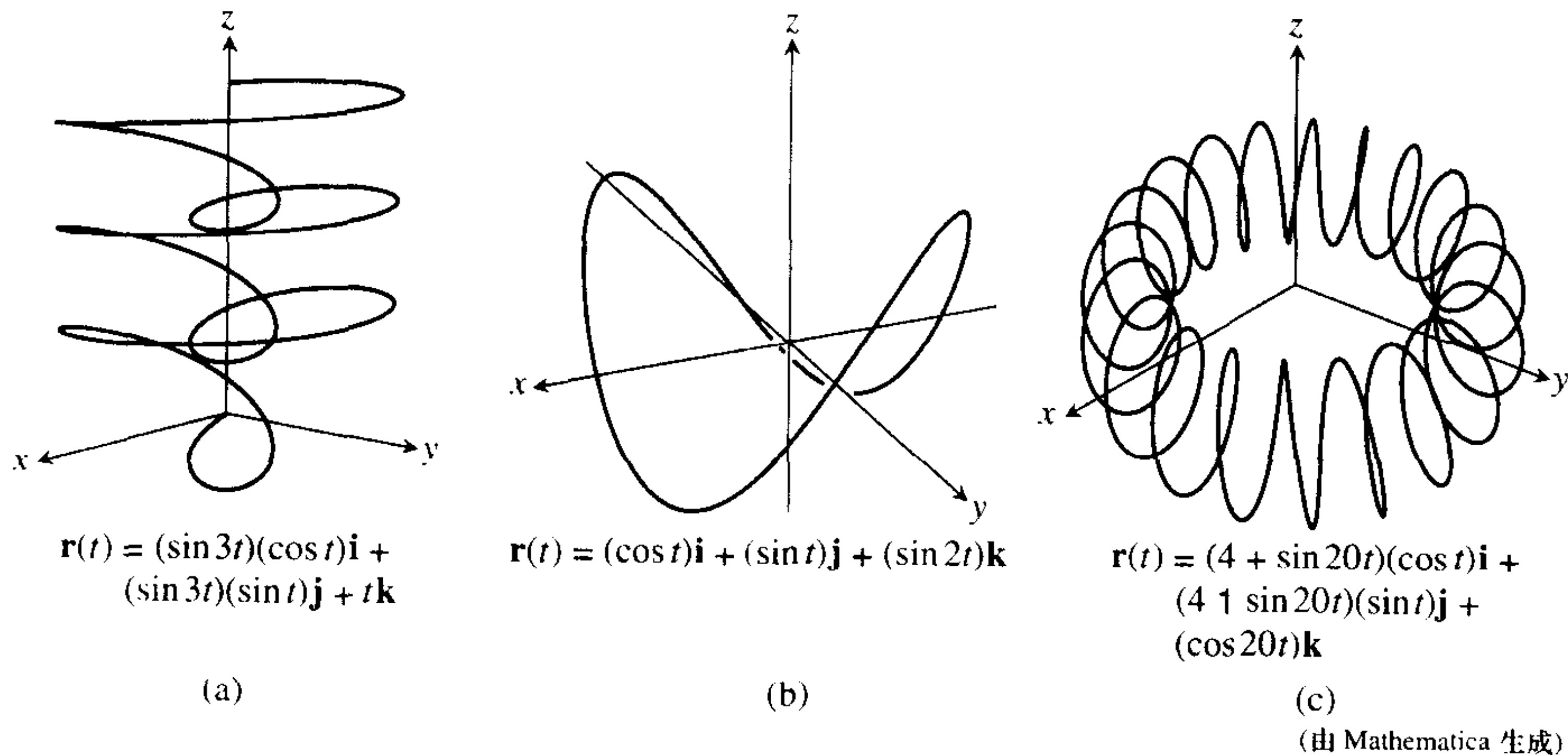
图 10.38 计算机生成的由位置向量定义的空间曲线
