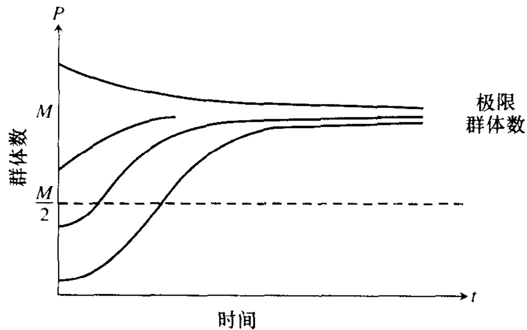
图 3.41 例 5 中的群体曲线.
