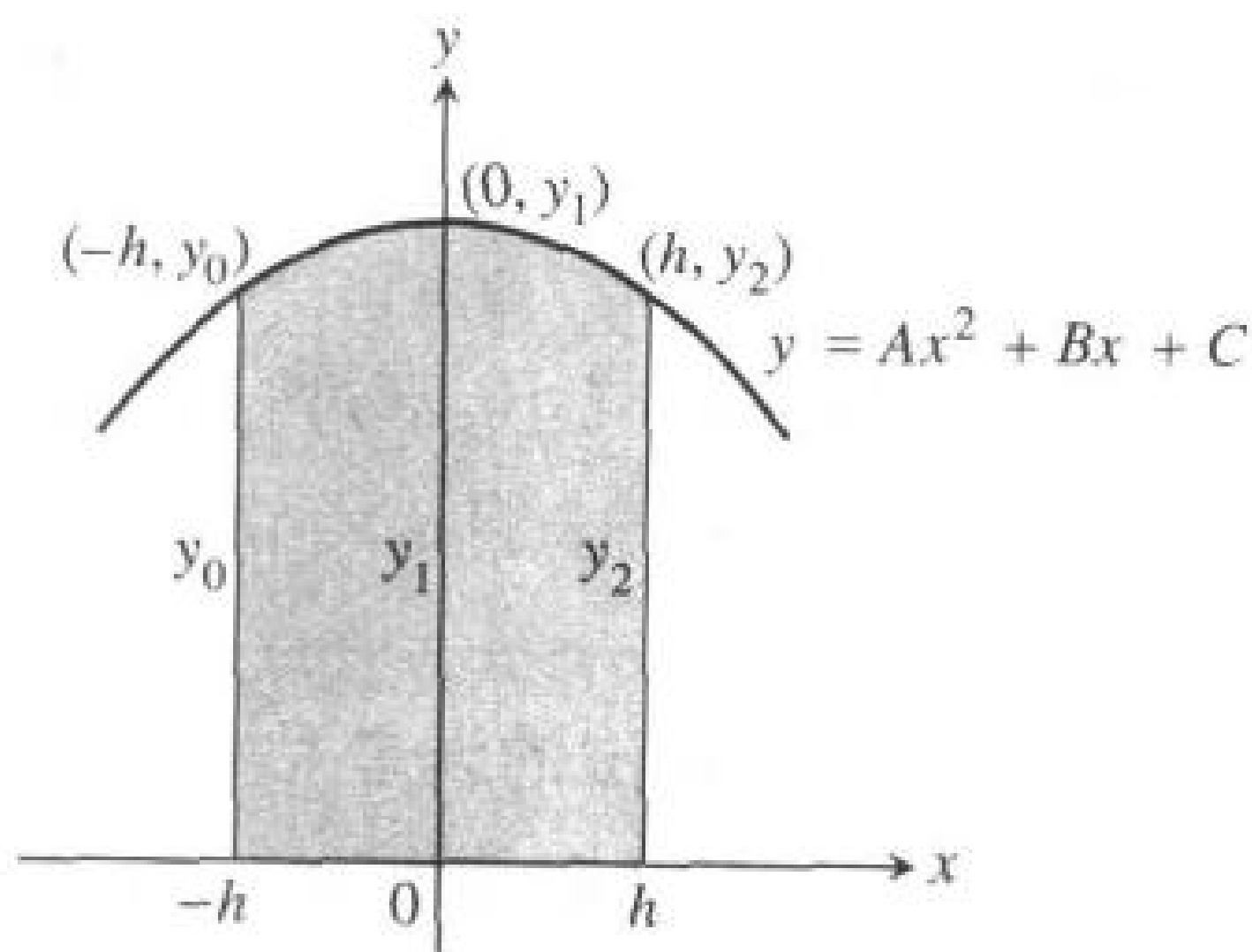
图 4.28 从 -h 到 h 积分, 我们求出阴影部分的面积是 \frac{h}{3}(y_0 + 4y_1 + y_2) .
