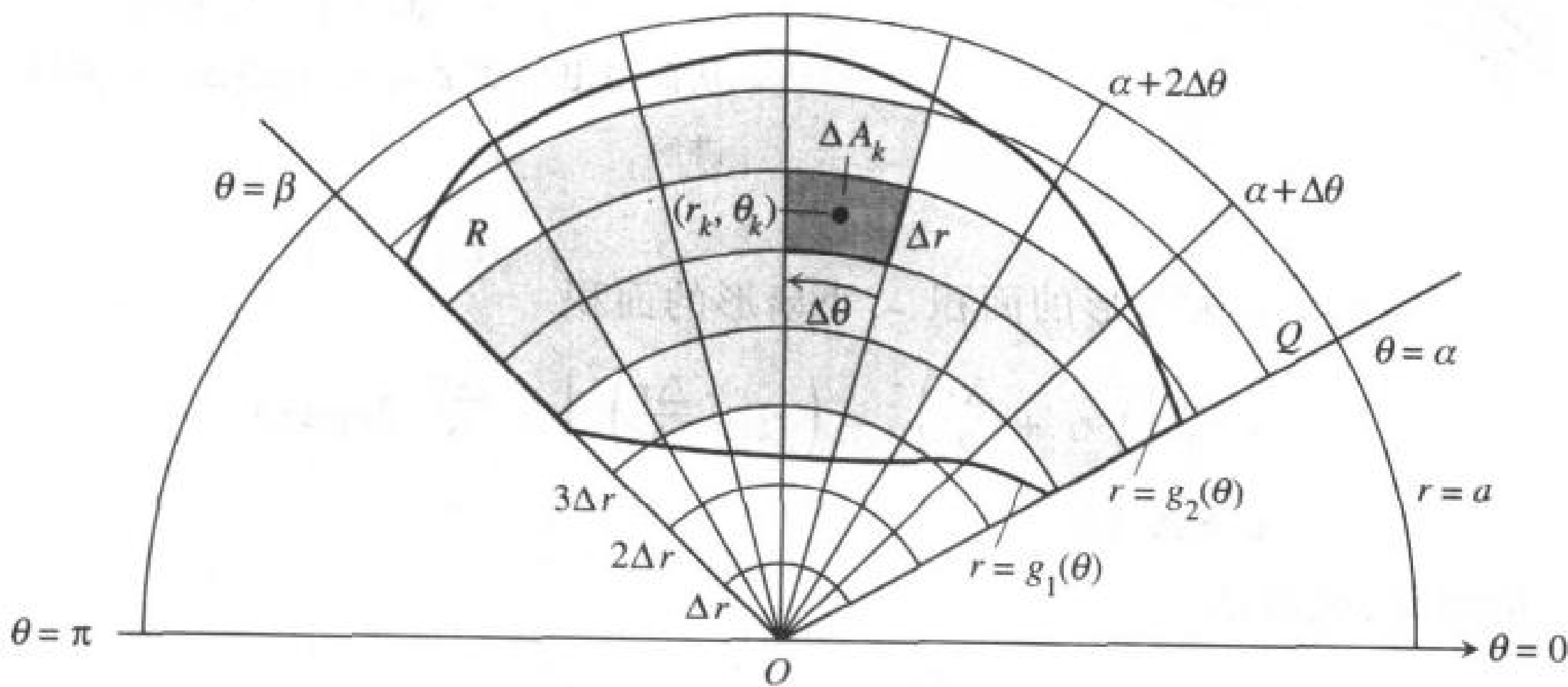
图 12.25 区域 R: g_1(\theta) \leq r \leq g_2(\theta), \alpha \leq \theta \leq \beta 包含在扇形区域 Q: 0 \leq r \leq a, \alpha \leq \theta \leq \beta 之内, 由圆弧与射线对 Q 的分割得到 R 的一个划分.
