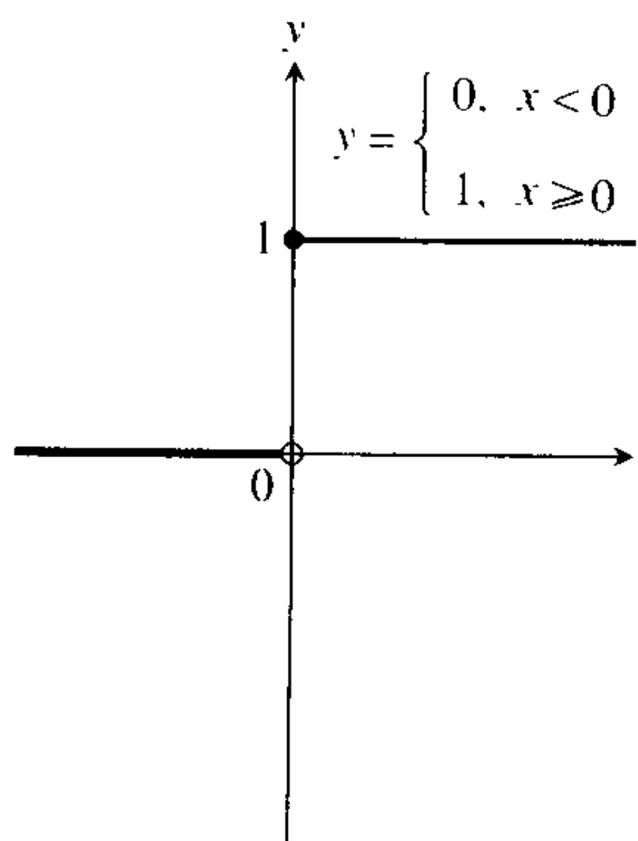
(a) 单位阶梯函数 U(x)
