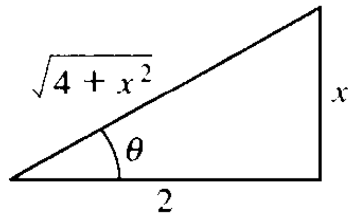
图 7.4 x = 2 \tan \theta (例 1) 的参考三角形: \tan \theta = x/2 ,
