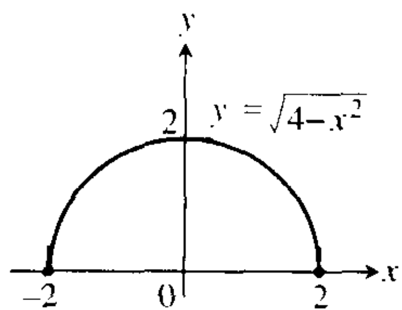
图 1.47 在定义域 每点连续的函数.
