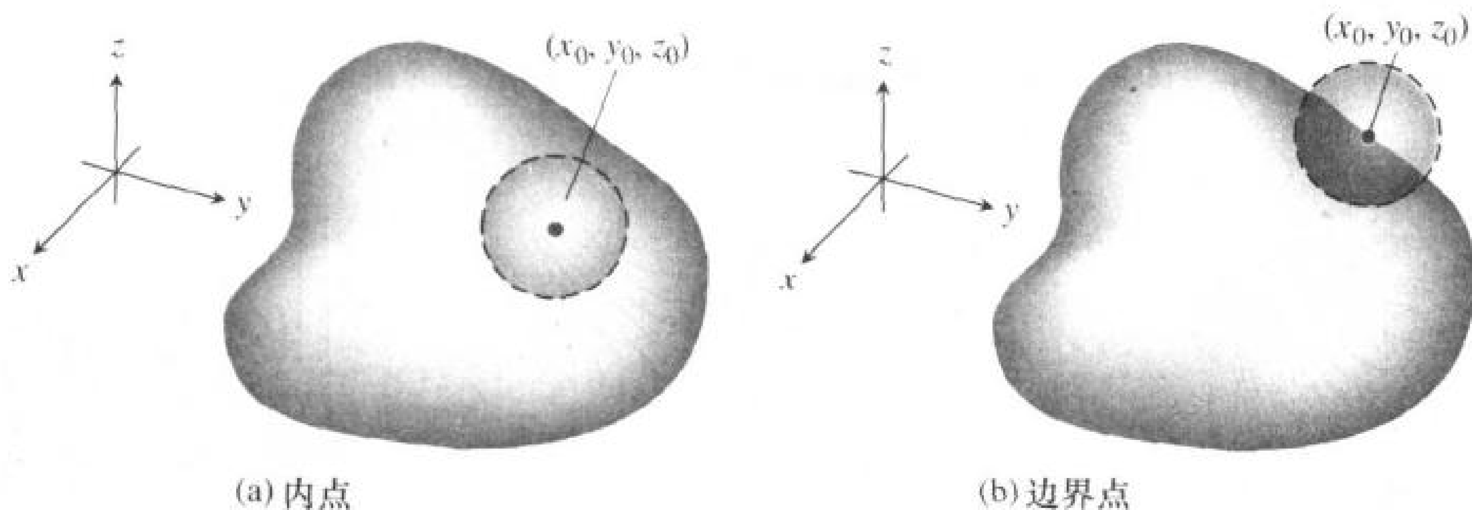
图 11.9 空间区域的内点和边界点
