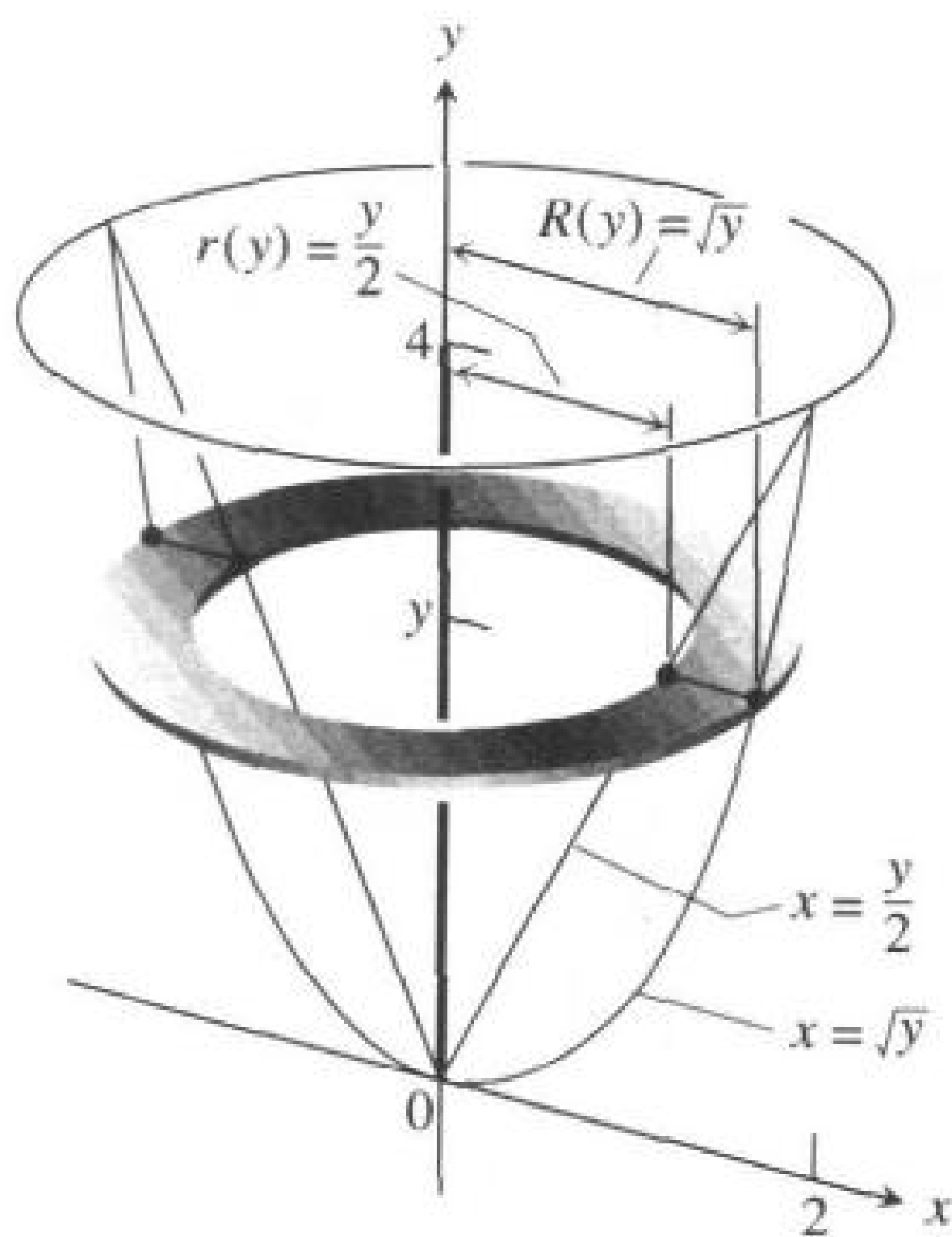
图 5.14 由在图 5.13 中的线段扫出的垫圈.
