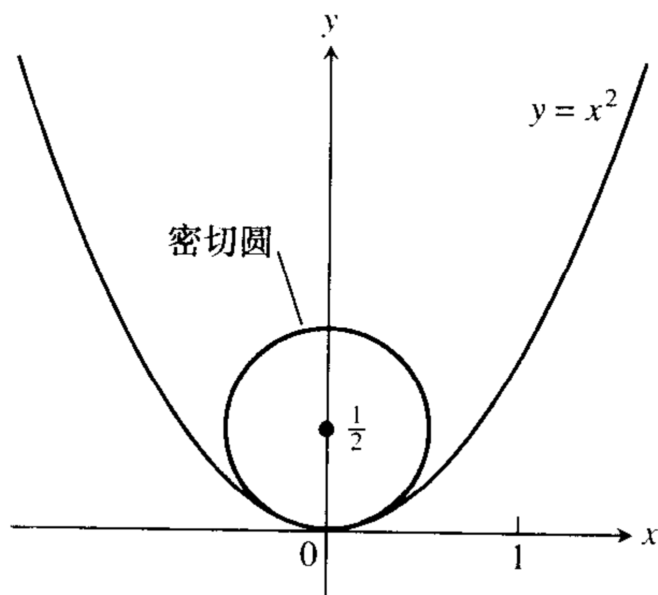
图 10.53 y = x^2 在原点的曲率圆 为 x^2 + \left(y - \frac{1}{2}\right)^2 = \frac{1}{4}
