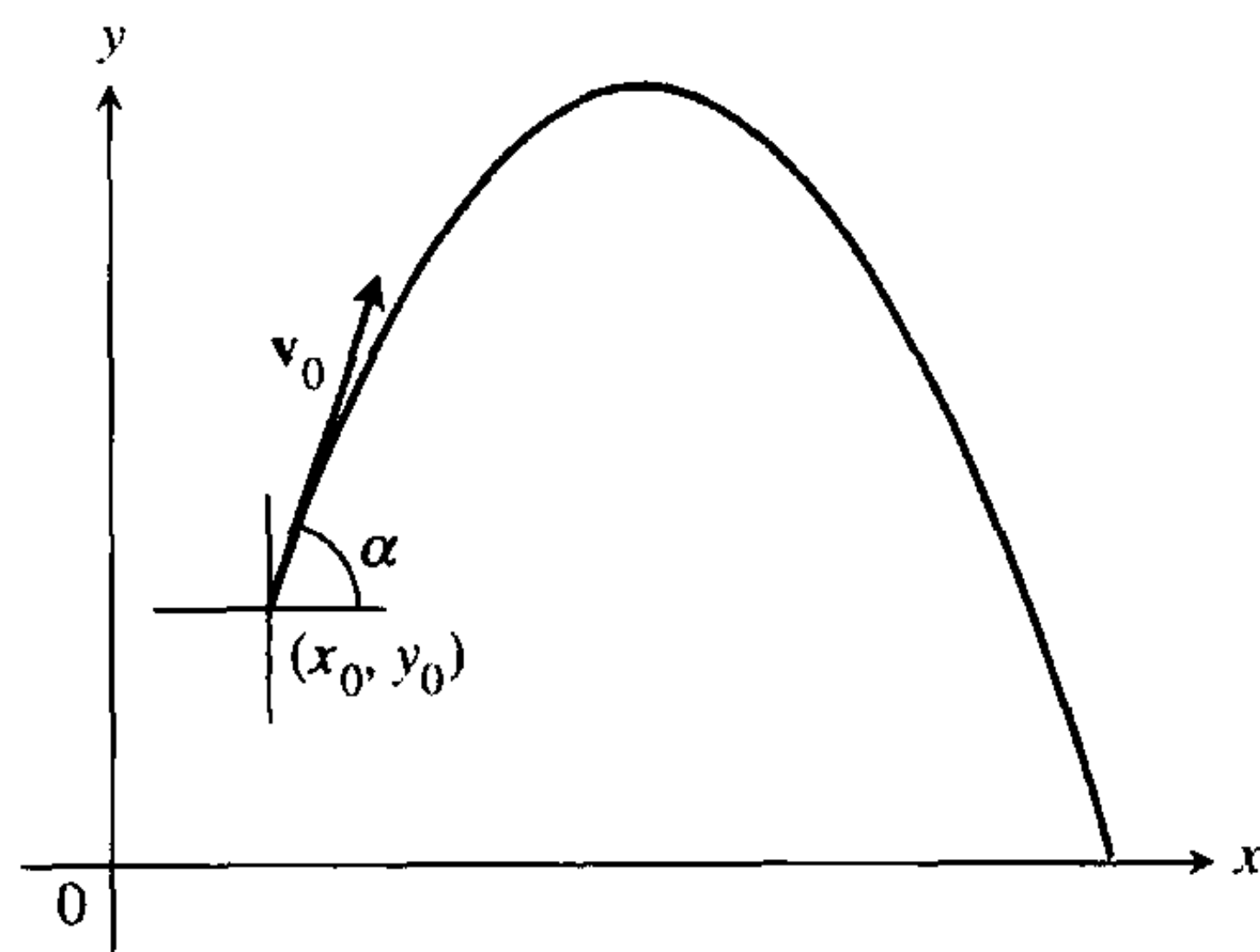
图 9.32 从 (x_0, y_0) 与水平线成 \alpha 度角的发射初速度为 v_0 的一个抛射体的路径.
