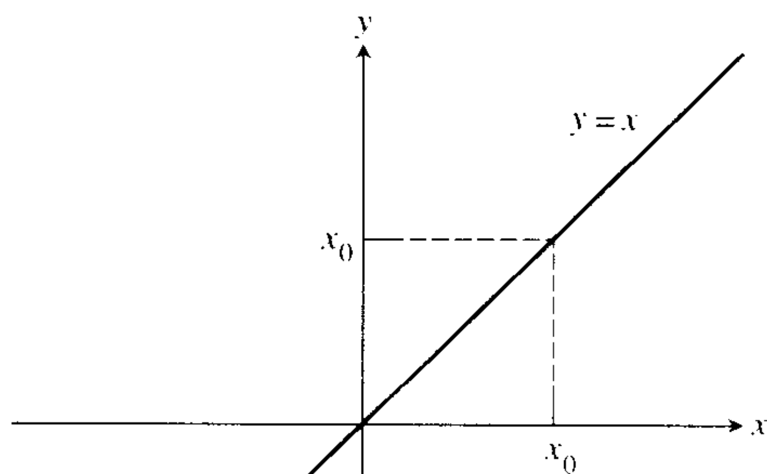
(a) 恒等函数
