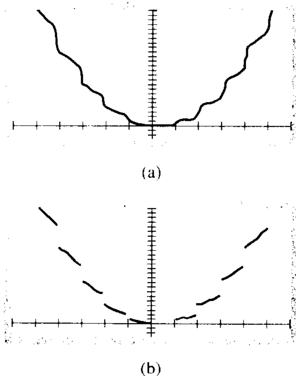
(a) 被不正确地以连通模式画出的 y_1 = x \times \operatorname{int} x 图形.(b) 以点模式正确地画出的 y_1 = x \times \operatorname{int} x 的图形.
