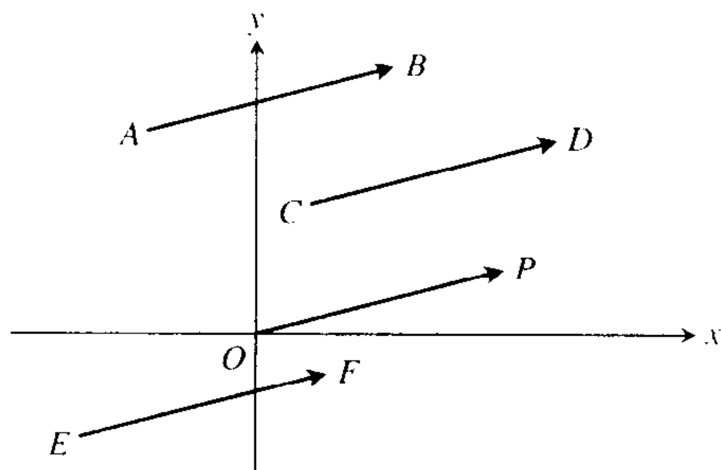
图 9.2 这里画的四个箭形(有向线段)有同一长度和方向.因此它们表示同一向量,并写成 \vec{AB} = \vec{CD} = \vec{OP} = \vec{EF}
