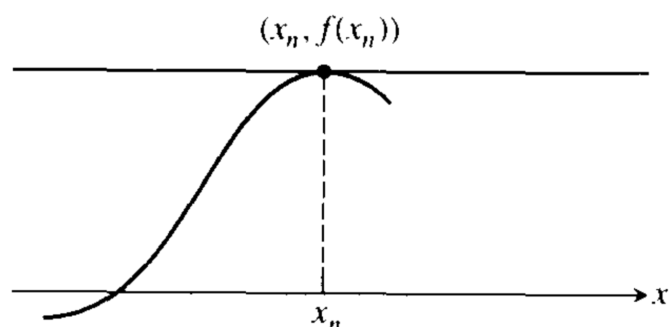
图 3.67 如果 f'(x_n) = 0 , 那么就没有能定义 x_{n+1} 的点.
