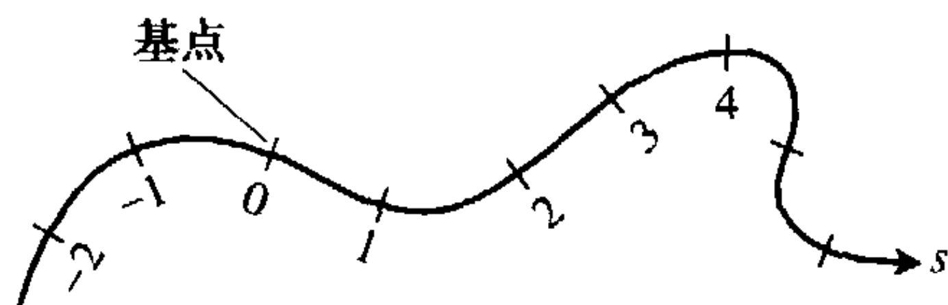
图 10.45 光滑曲线可像数直线一样度量,对等的,对每一点,为从预先选定的基点到该点的有向距离
