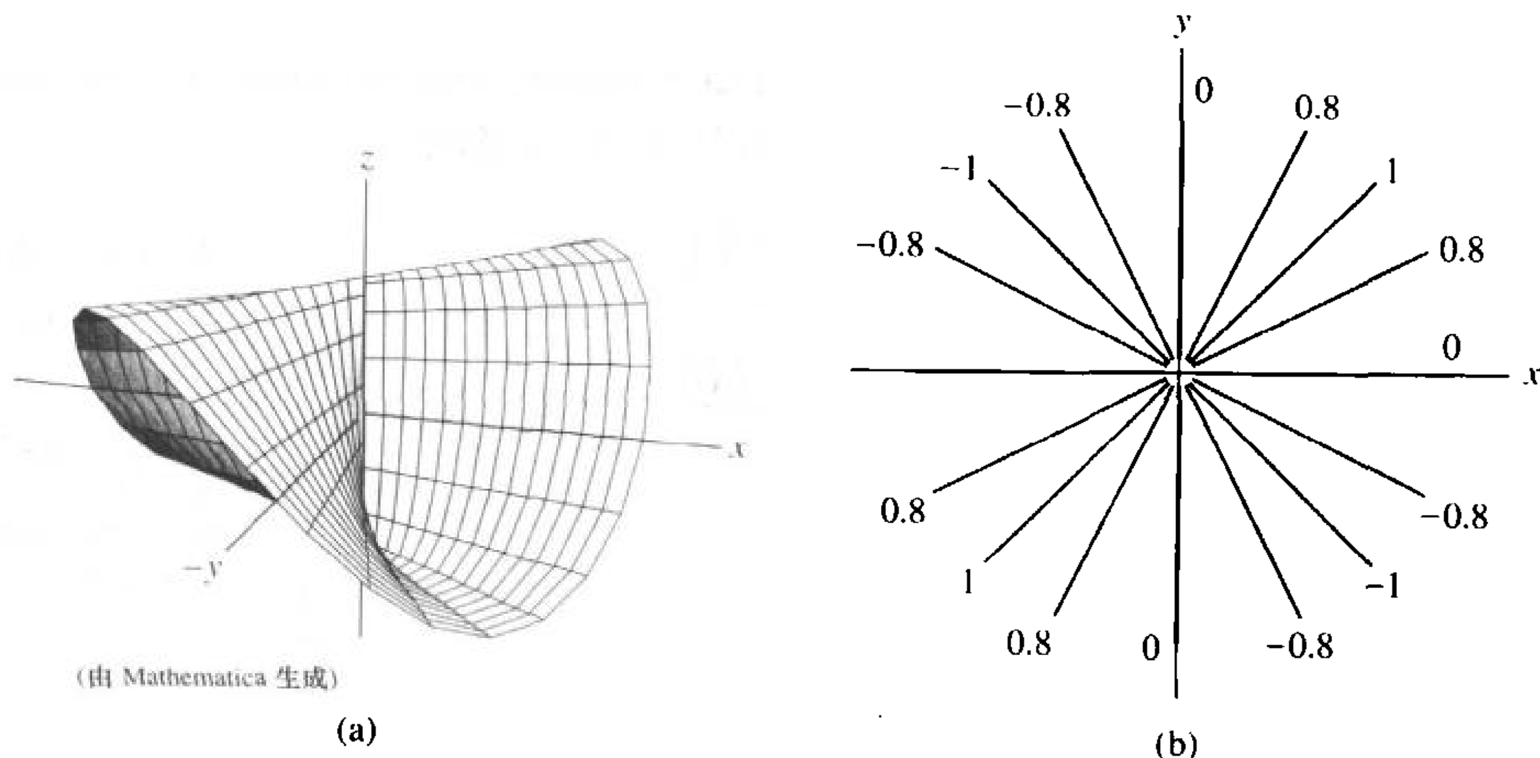
图 11.11 (a) f(x, y) = \begin{cases} \frac{2xy}{x^2 + y^2}, & (x, y) \neq (0, 0) \\ 0, & (x, y) = (0, 0) \end{cases} 的图形. 函数在 origin 以外的每个点连续.
