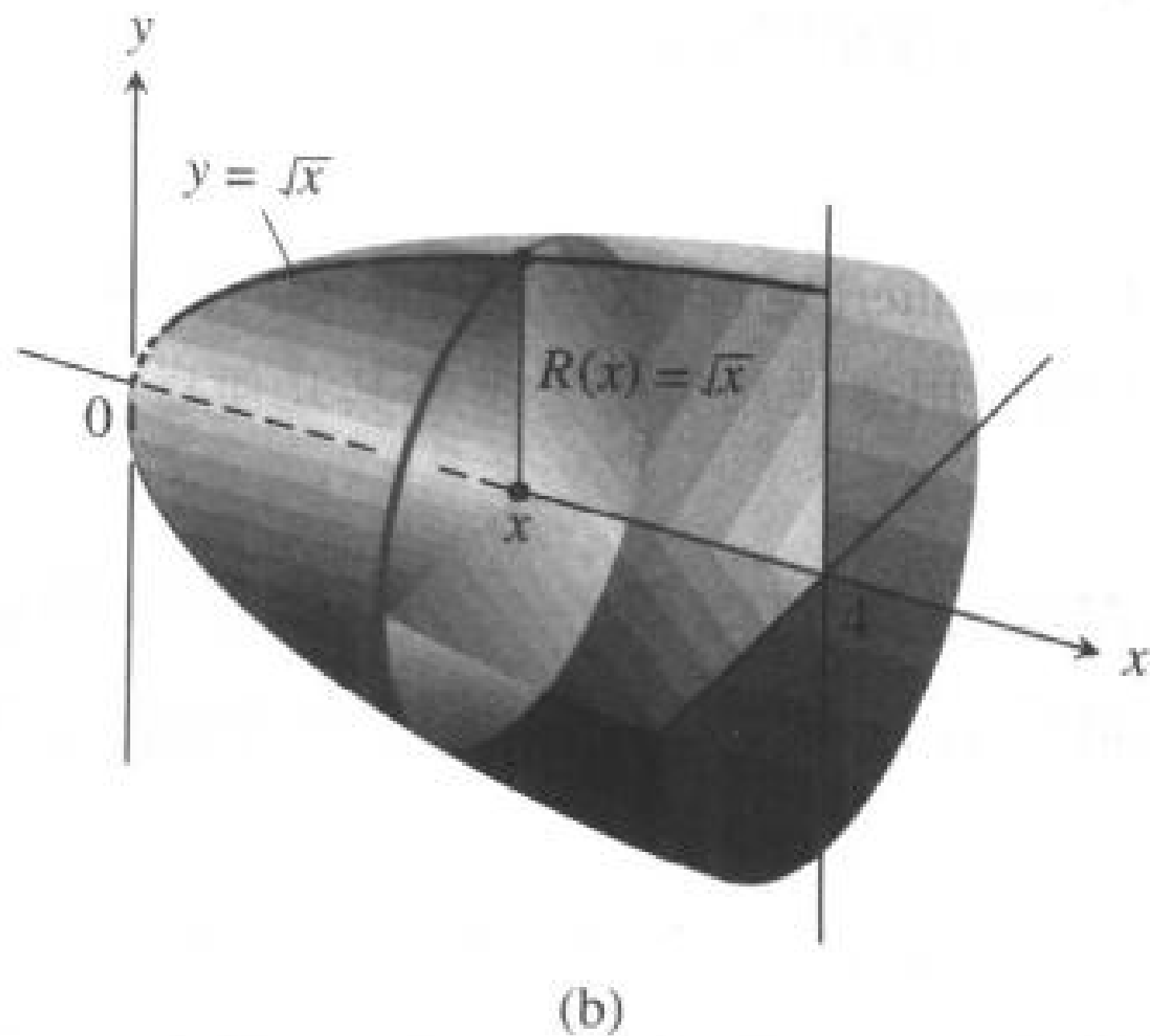
图 5.6 例 4 中的区域(a) 和立体(b).
