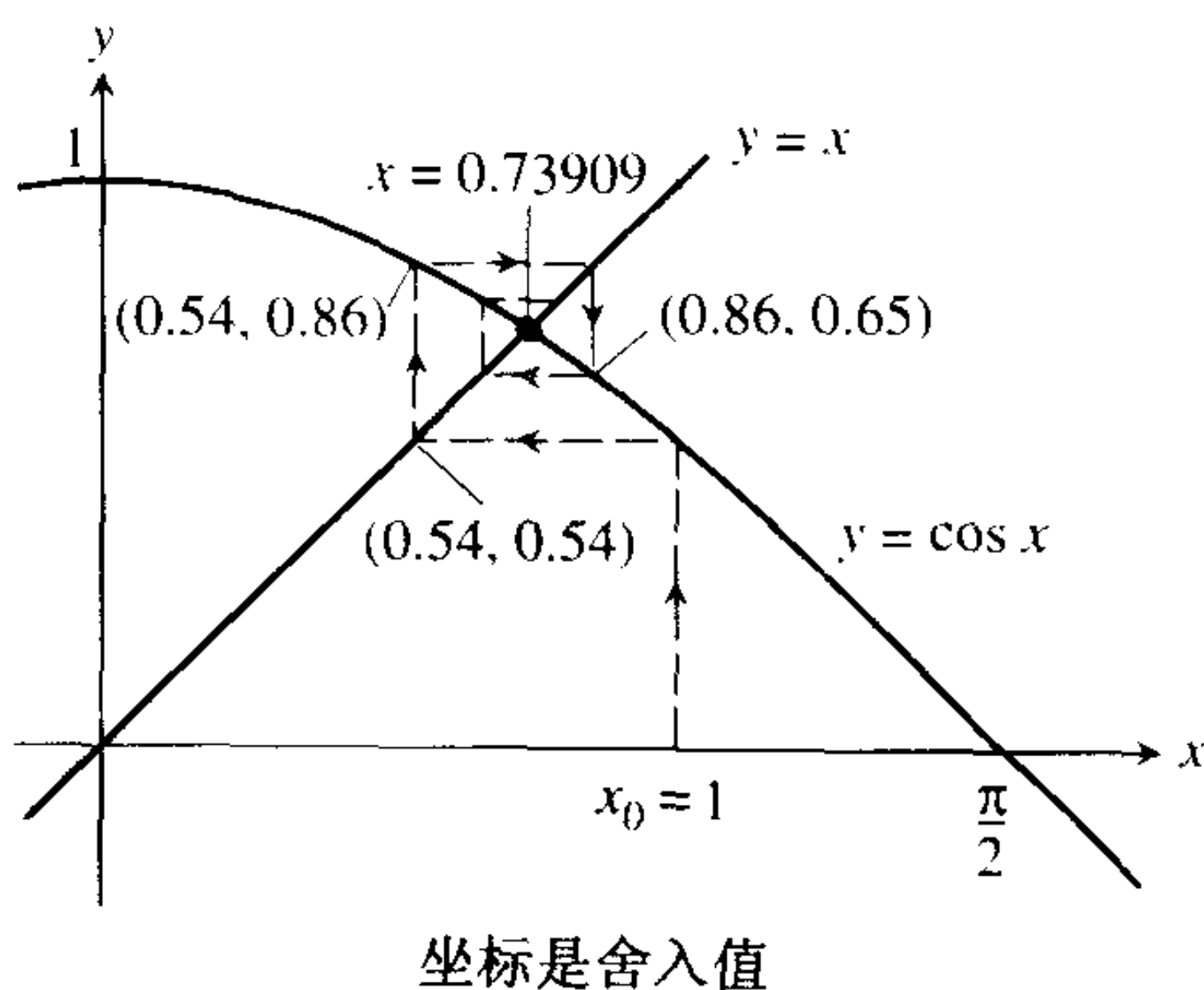
图 8.7 从 x_0 = 1 开始的 \cos x = x 的皮卡方法给出的解.(例 8)
