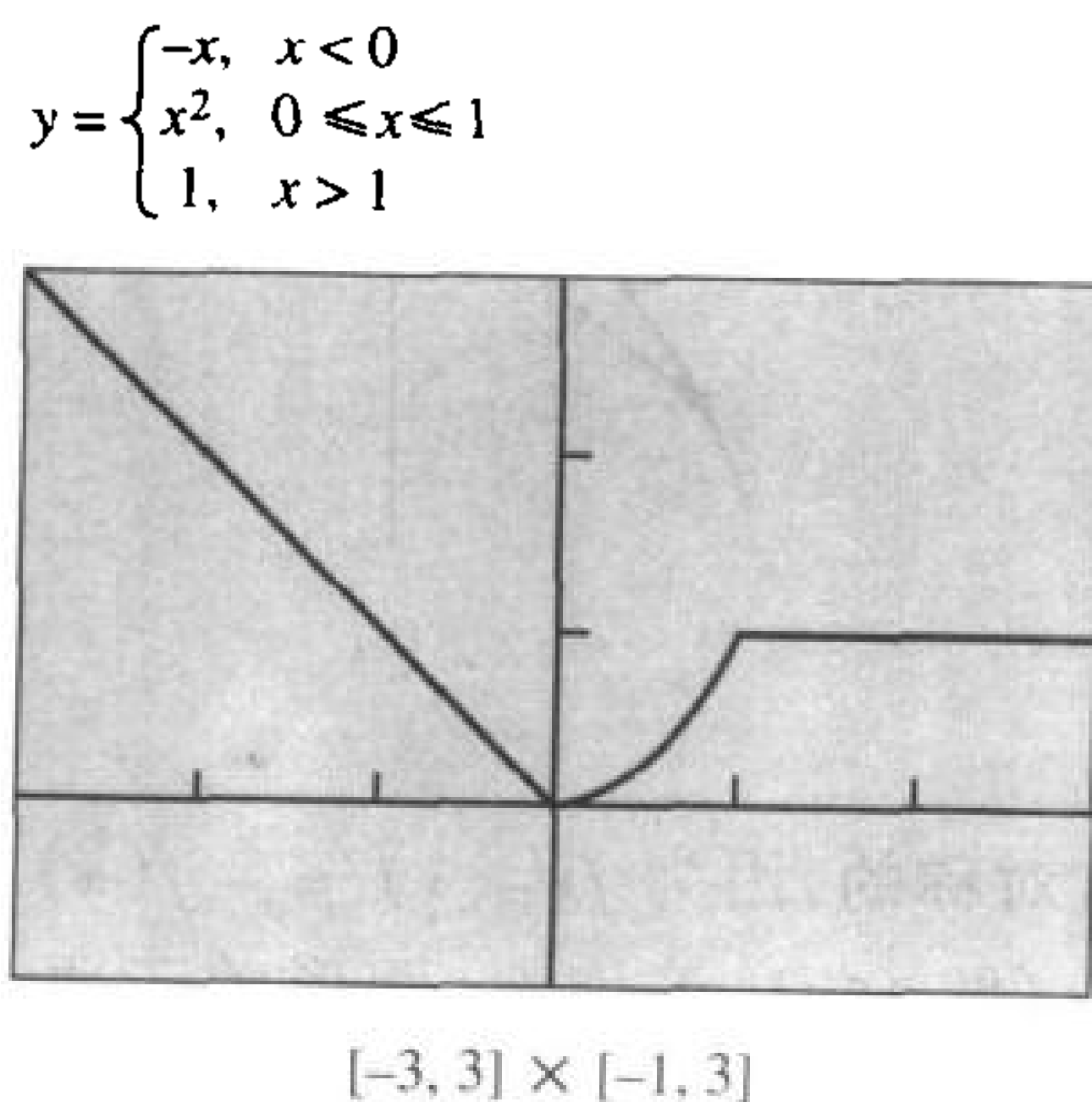
图 17 分段定义的函数的图形. (例 5)
