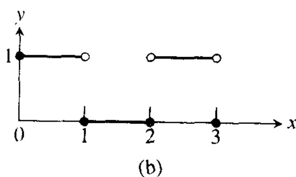
图 4.31 习题 17 和 18 中的图象.
