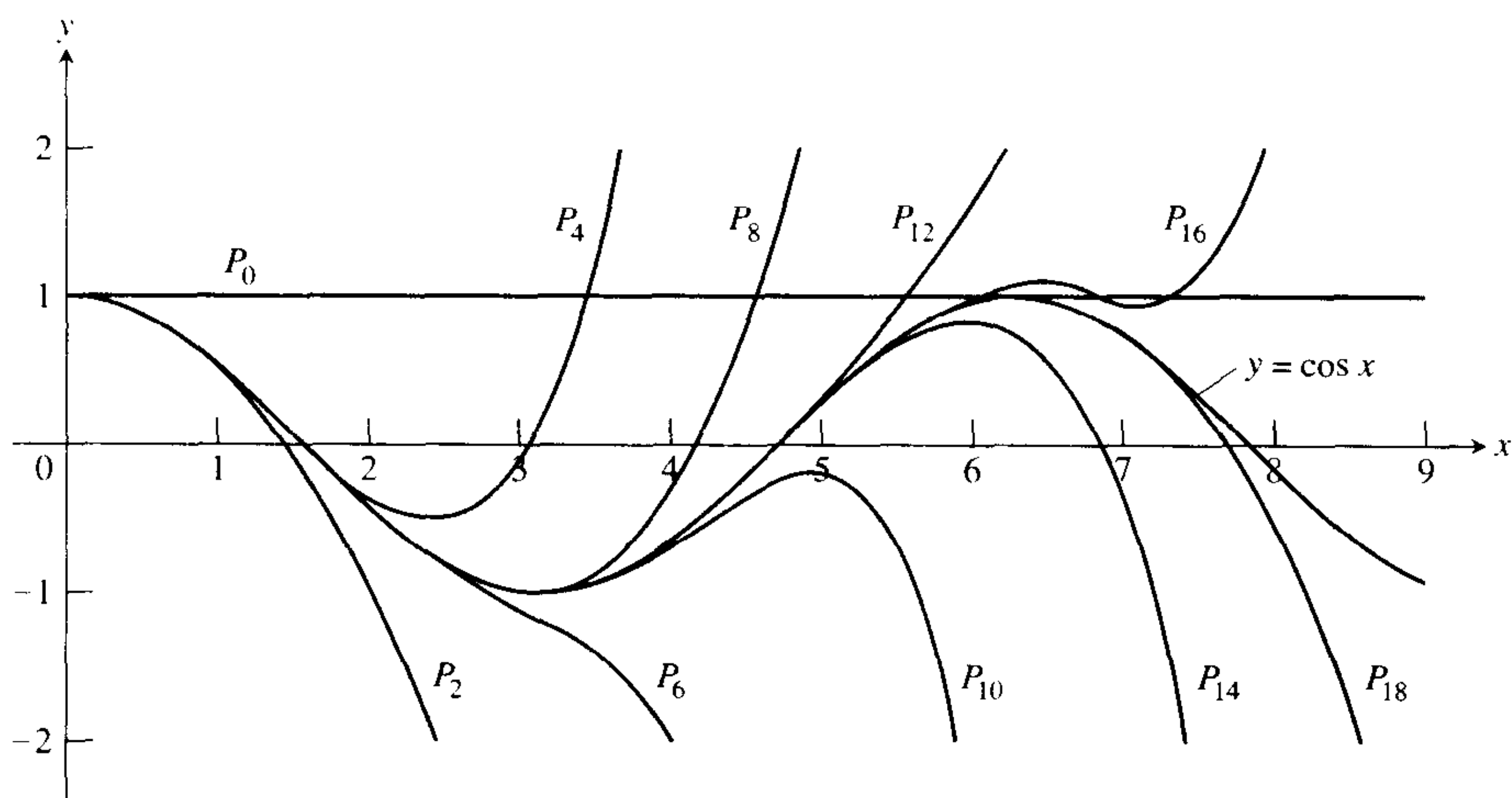
图 8.19 多项式 P_{2n}(x) = \sum_{k=0}^n \sum_{k=0}^n \frac{(-1)^k x^{2k}}{(2k)!} 当 n \rightarrow \infty 时收敛到 \cos x . 我们可以
