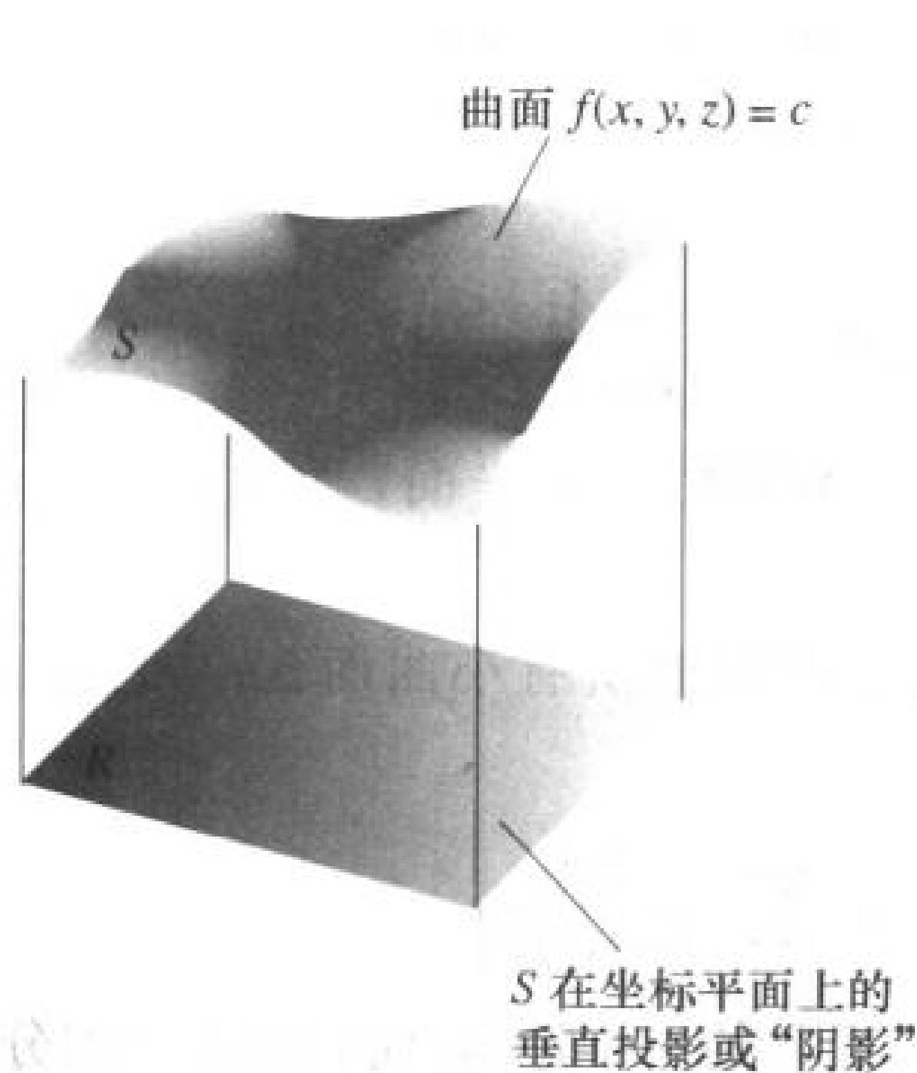
图 13.38 很快就会看到,函数 g(x, y, z) 在空间曲面 S 上的积分能够用在坐标平面上 S 的垂直投影或“阴影”上的一个相关的二重积分来计算.
