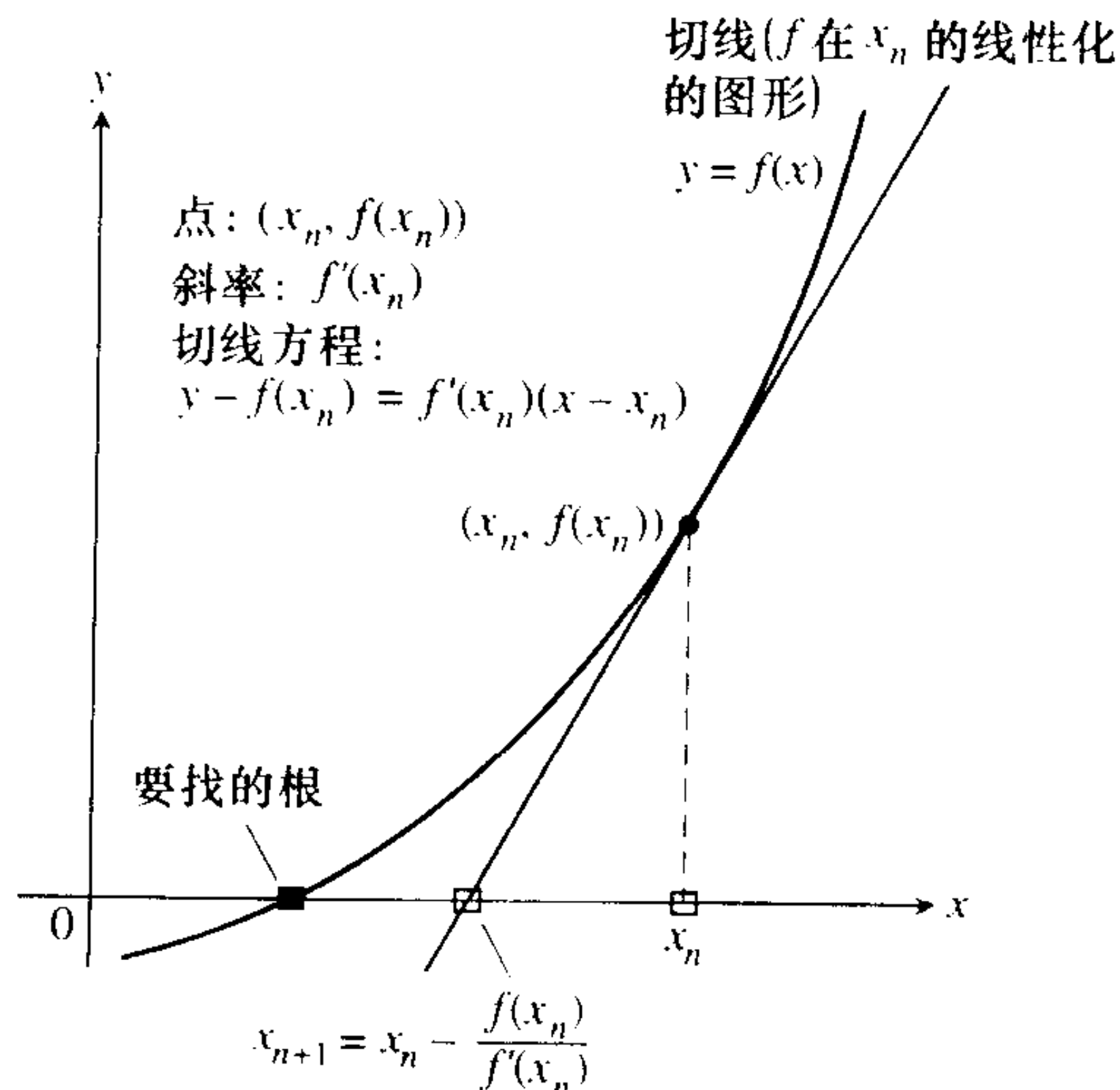
图 3.62 Newton 法逐次步骤的几何表示. 从 x_n 向上与曲线相交, 然后作切线往下与 x 轴相交, 求得 x_{n+1} .
