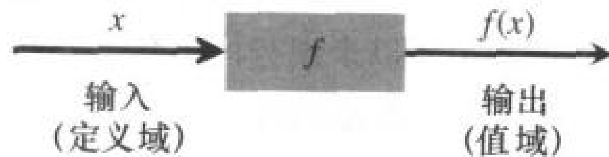
图 8 函数的“机器”图示
