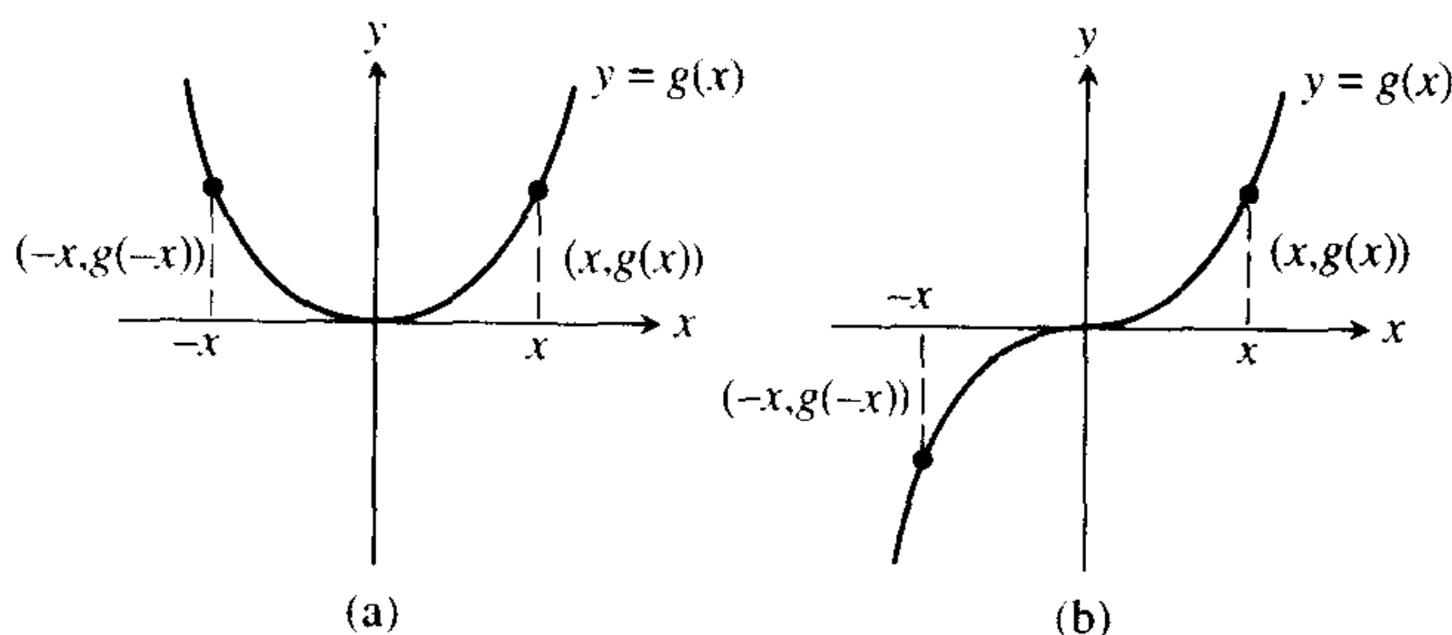
图 8.25 (a) 偶函数的图象关于 y 轴对称. (b) 奇函数的图象关于原点对称.
