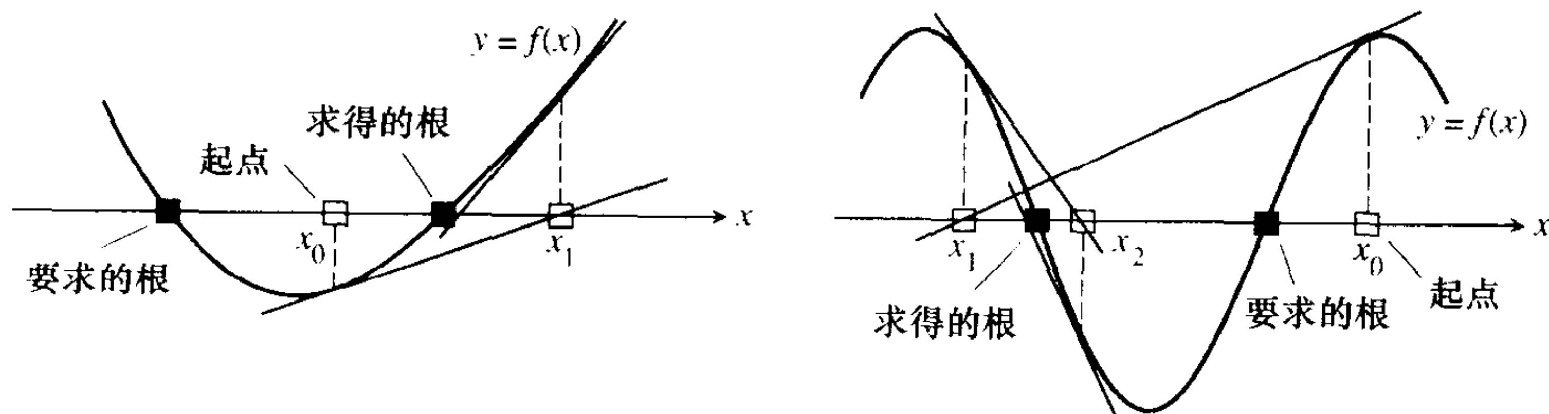
图 3.69 如果你从很远的地方开始, Newton 法可能会找不到你想要的根.
