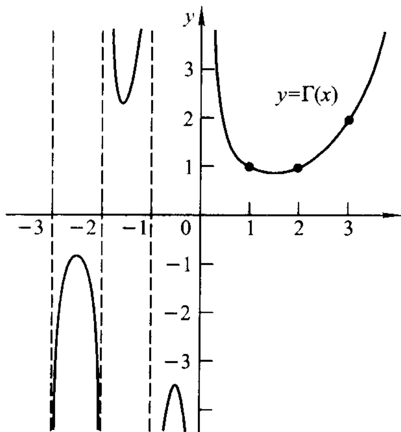
图 7.21 \Gamma(x) 是 x 的连续函数, 它在每个正整数 n+1 的值是 n! . 对 \Gamma 的定积分公式仅对 x > 0 有效, 但是我们可以用公式 \Gamma(x) = \frac{\Gamma(x+1)}{x} 把 \Gamma
