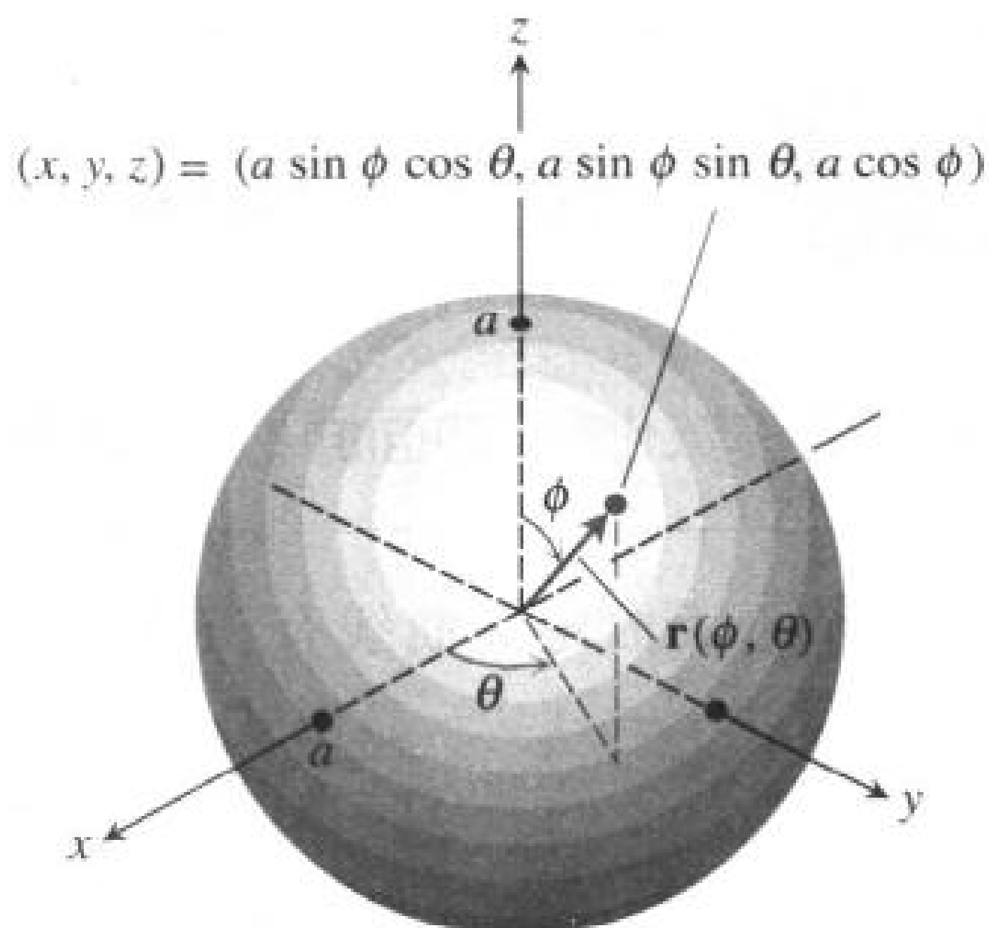
图 13.52 例 2 中的球面.
