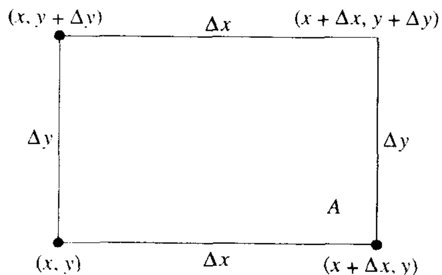
图 13.24 用于定义向量场在一点 (x, y) 的流量密度(散度)的小矩形.
