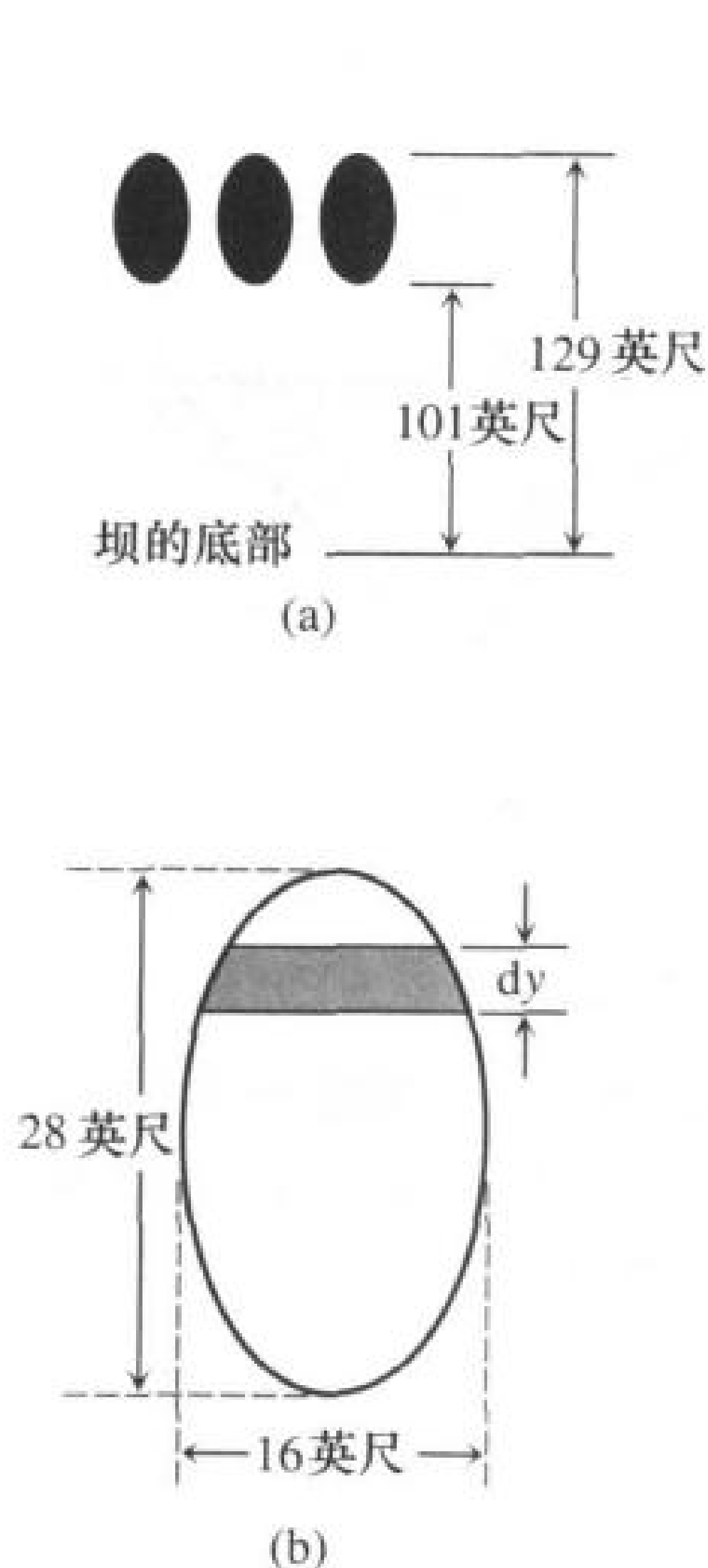
图 5.43 (a) 从坝的底部算起的水闸门的位置. (b) 水闸门分为水平条的放大图
