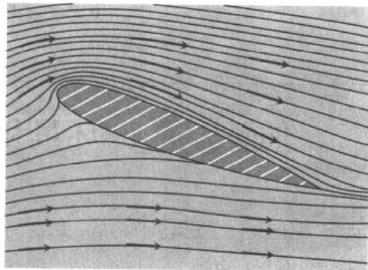
图 13.10 风洞内飞机机翼附近流体的速度向量.由煤油烟做出的可视流线.(摘自 NCFMF book of Film Notes , 1974, MIT 教育发展中心出版社; Inc., Newton, Massachusetts.)
