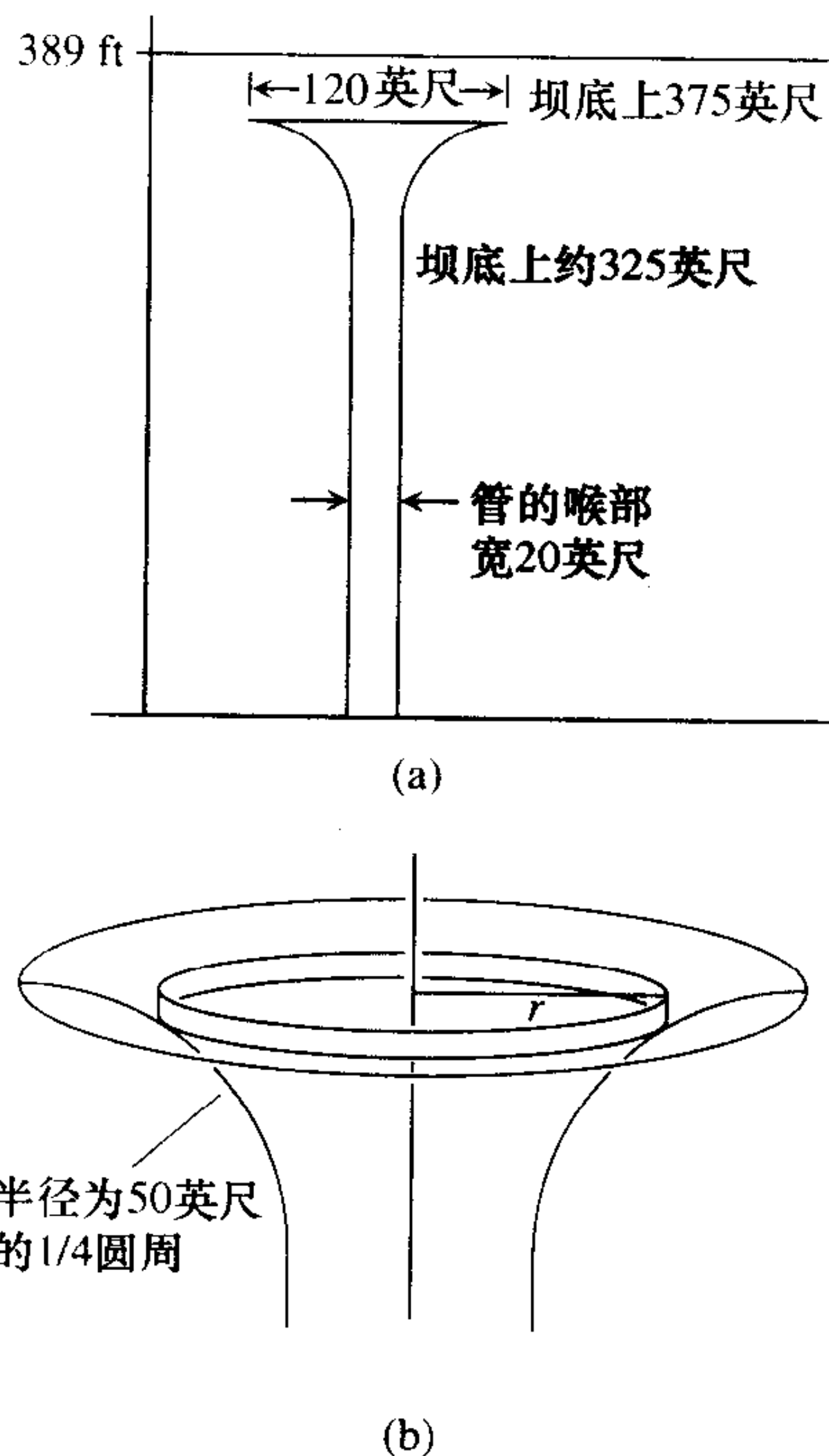
图 5.36 (a) 一个坝的竖井的横截面. (b) 竖井的顶部
