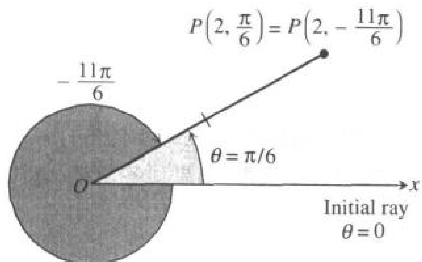
图 9.36 极坐标不是唯一的.
