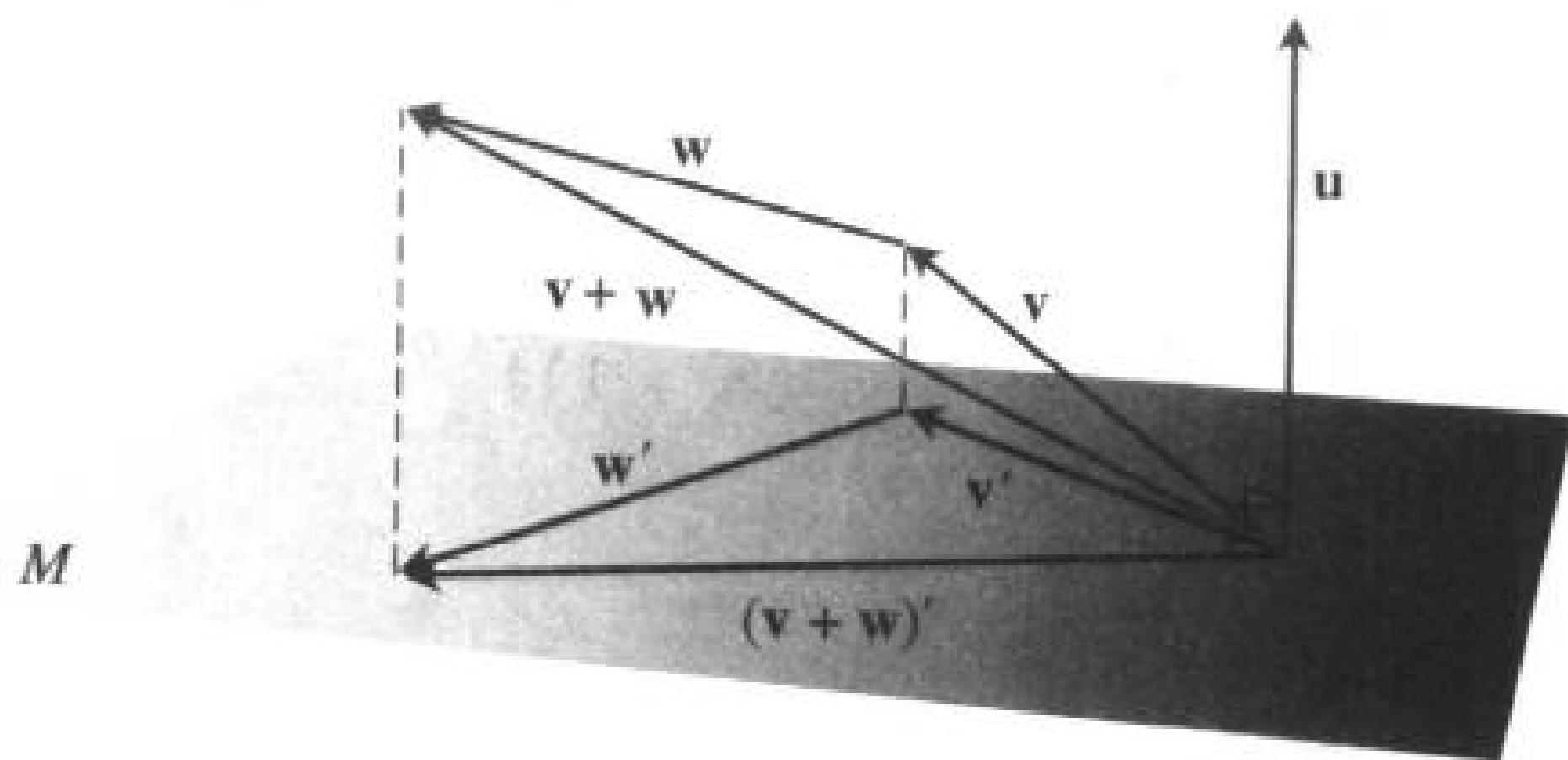
图 A.13 向量 \mathbf{v}, \mathbf{w}, \mathbf{v} + \mathbf{w} 以及它们在垂直于 \mathbf{u} 的平面上的投影.
