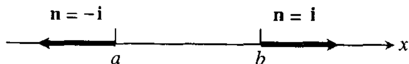
图 13.77 一维空间 [a, b] 边界的向外单位法方向.
