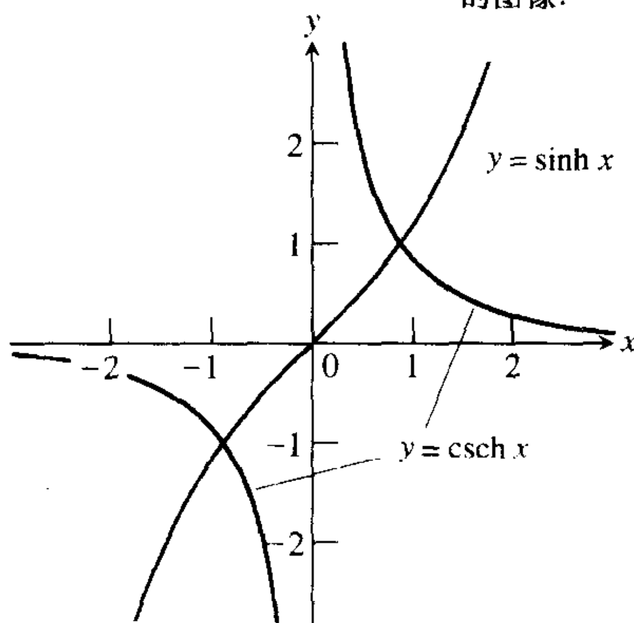
(e) y = \sinh x 和 y = \operatorname{csch} x = 1/\sinh x 的图像.
