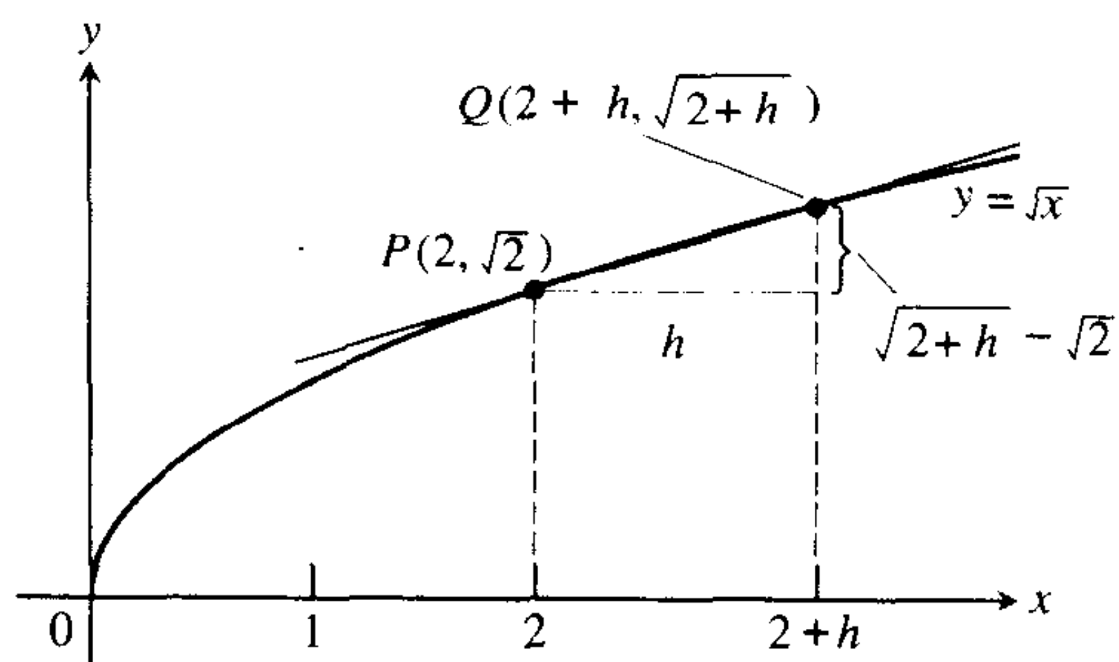
图 1.16 当 Q 沿曲线趋近 P 时割线 PQ 的斜率
