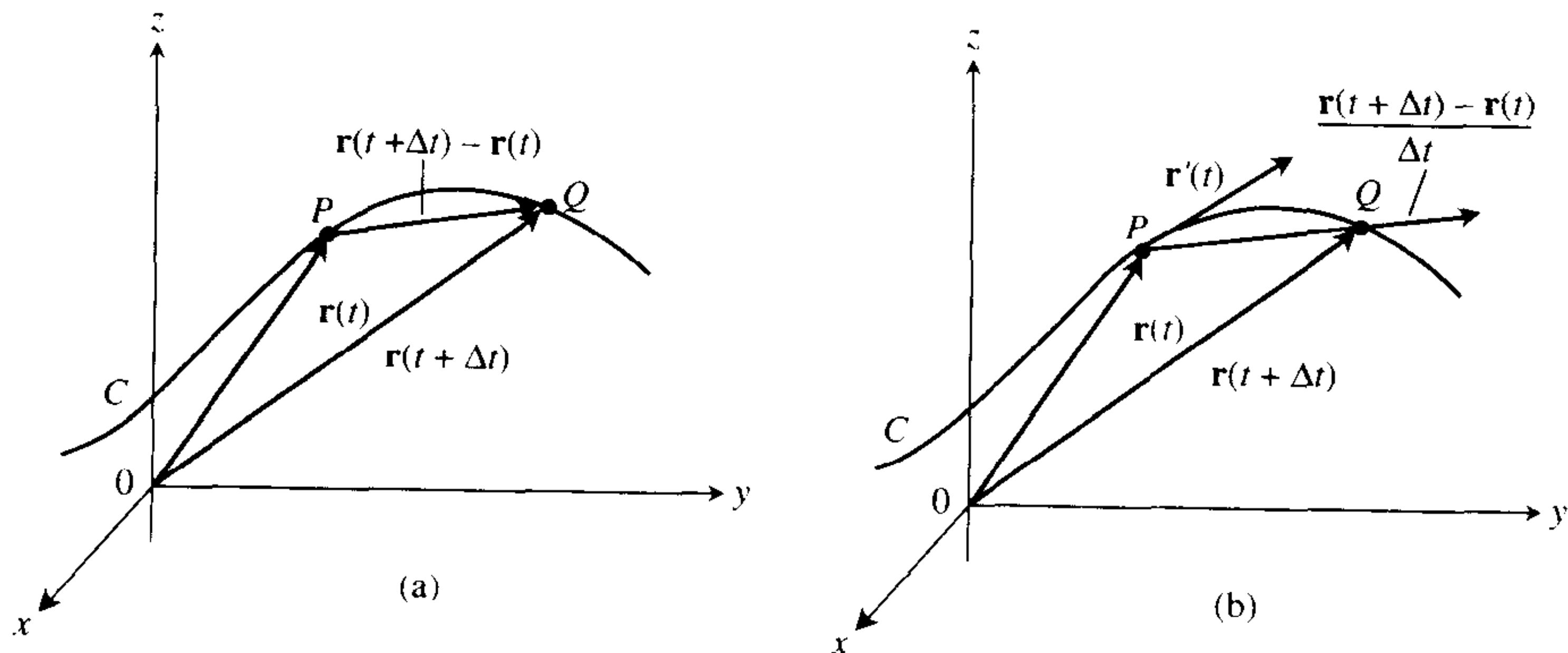
图 10.41 当 \Delta t \rightarrow 0 时, 点 Q 沿曲线 C 趋向于 P , 向量 \overrightarrow{PQ}/\Delta t 的极限值则为切向量 \mathbf{r}'(t) .
