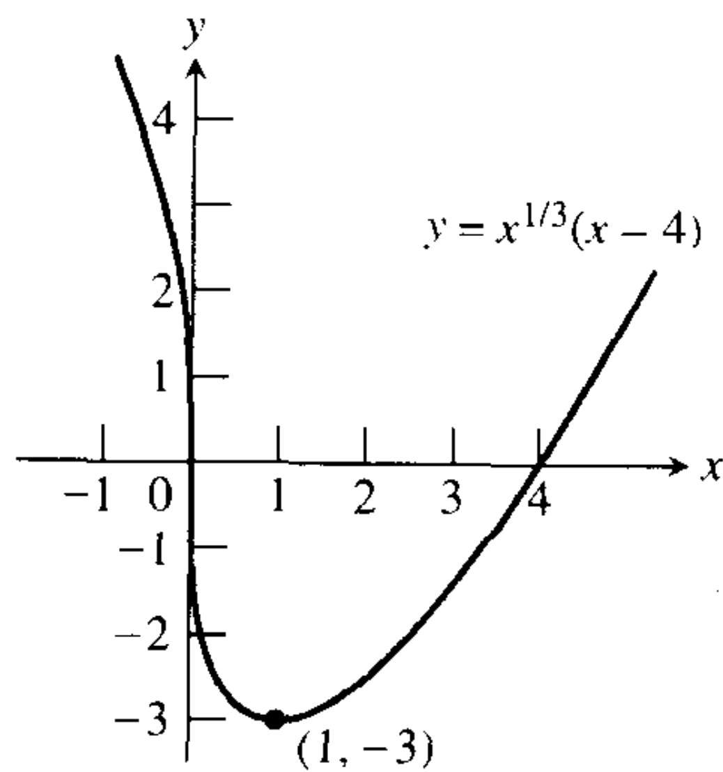
图 3.23 y = x^{1/3}(x - 4) 的图形.(例 2)
