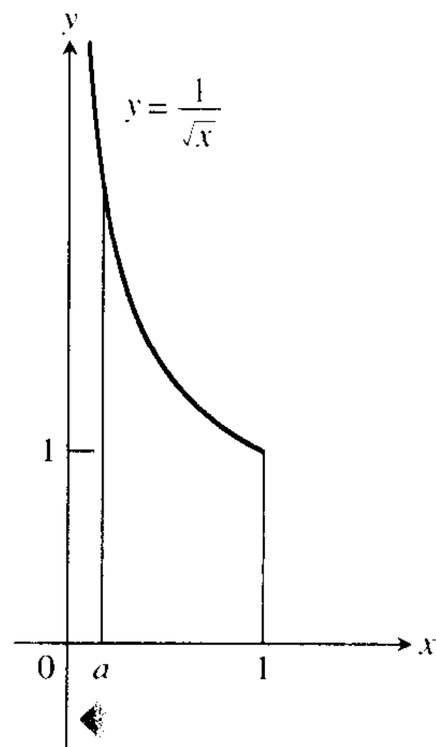
图 7.15 曲线下的面积是
