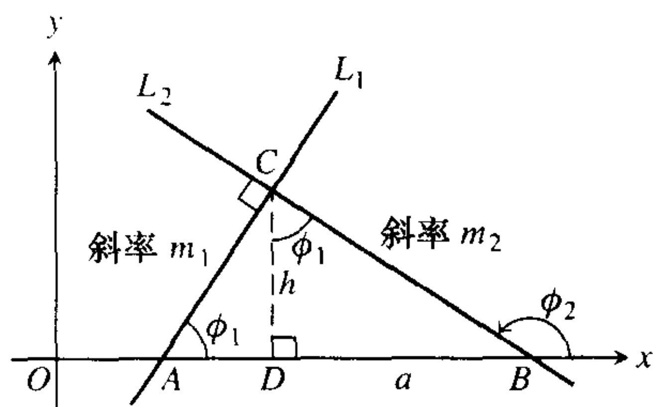
图3 \triangle ADC 与 \triangle CDB 相似. 因此 \phi_1 也是 \triangle CDB 的上角, \tan \phi_1 = \frac{a}{h} .
