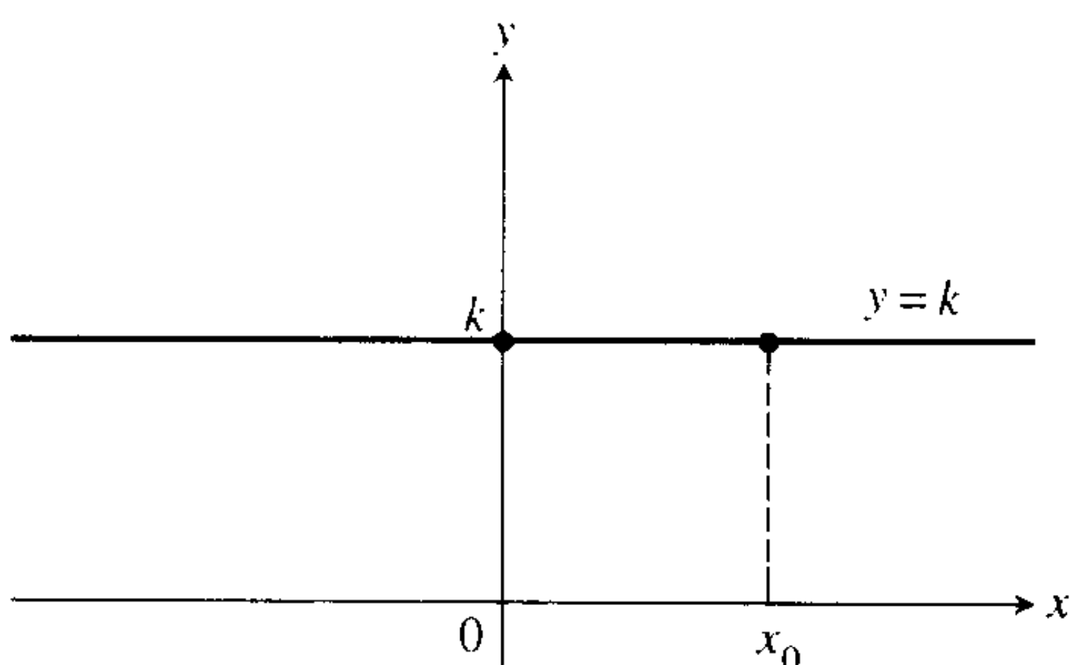
(b) 常数函数
