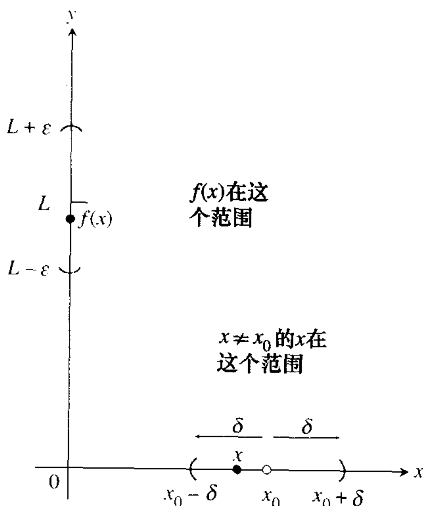
图 1.11 极限定义中 \delta 和 \varepsilon 的关系.
