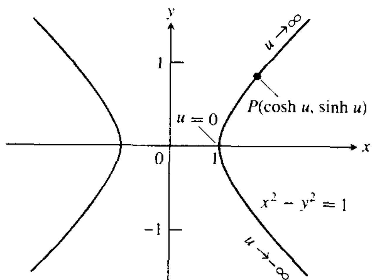
图 6.29 因为 \cosh^2 u - \sinh^2 u = 1 , 所以对于任一 u 的值, 点 (\cosh u, \sinh u) 落在双曲线 x^2 - y^2 = 1 的右分支上. (题 84)
