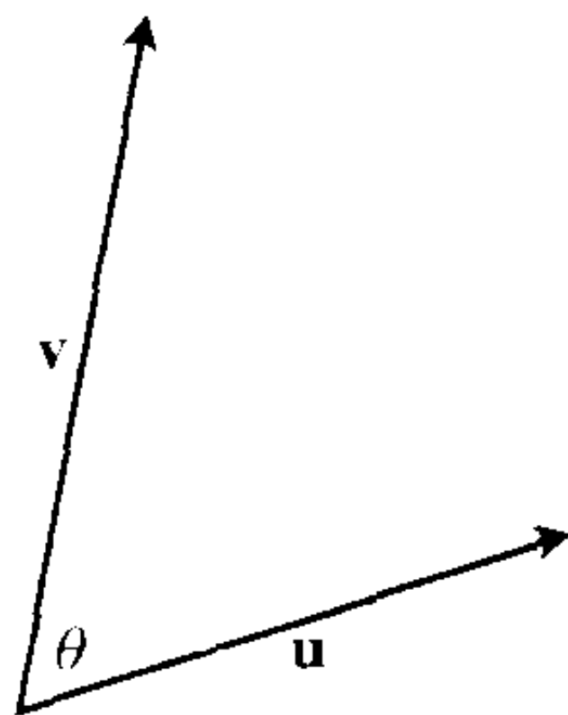
图 9.15 \mathbf{u} 和 \mathbf{v} 之间的夹角.
