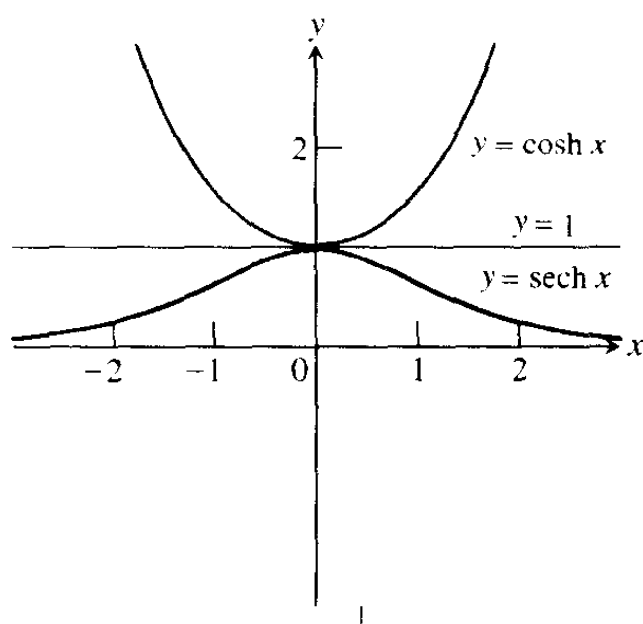
(d) y = \cosh x 和 y = \operatorname{sech} x = 1/\cosh x 的图像.
