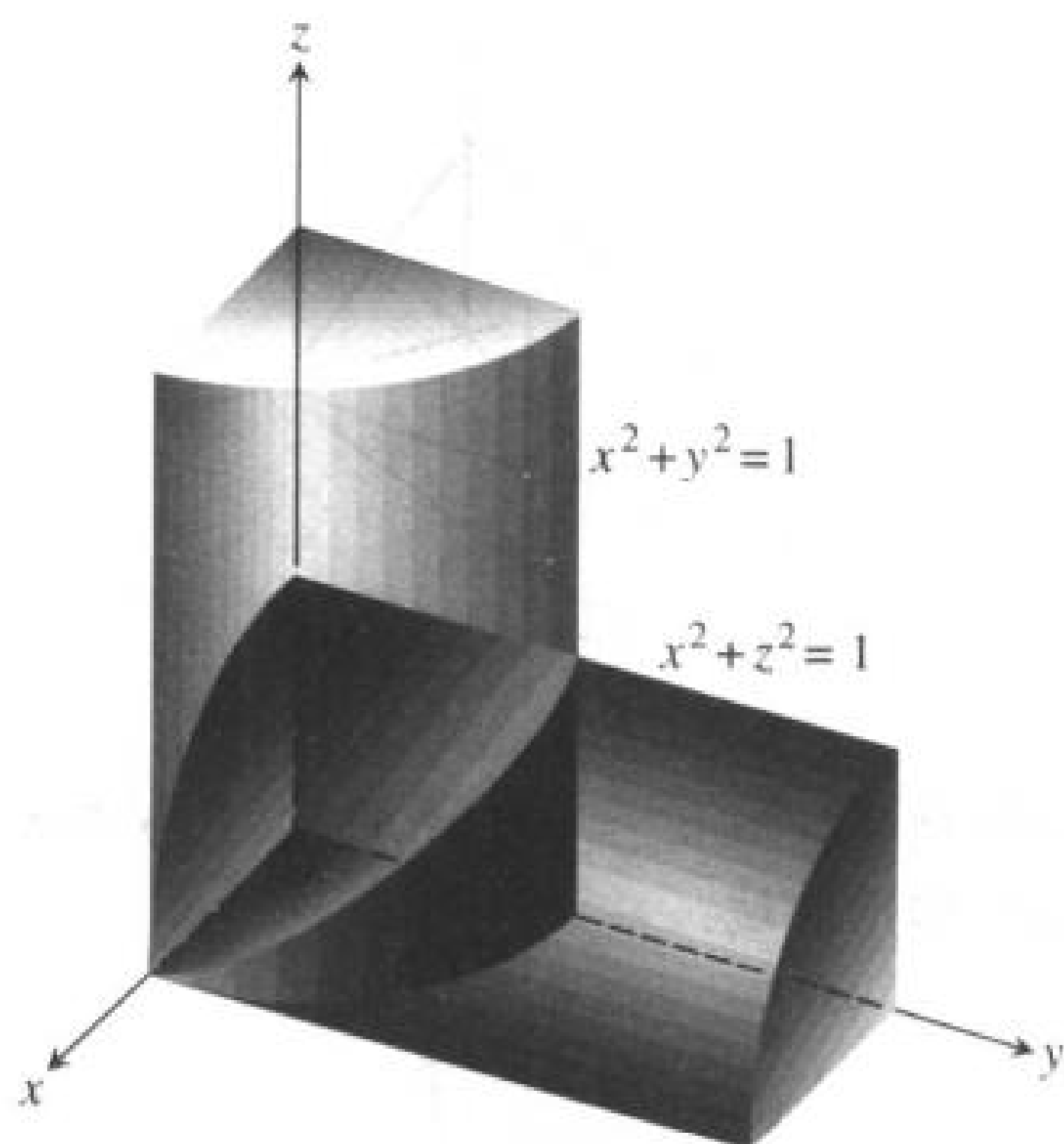
图 12.36 题 29 中两柱面 x^2 + y^2 = 1 和 x^2 + z^2 = 1 的公共部分区域的 1/8 .
