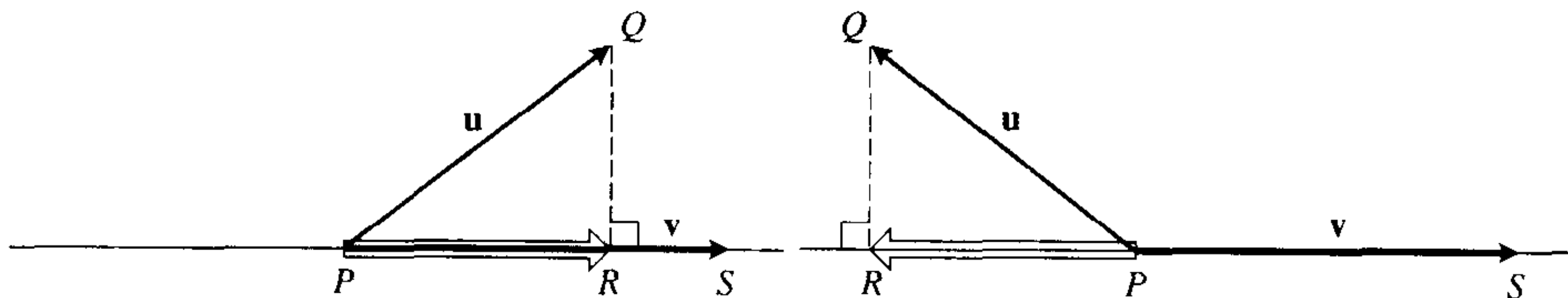
图 10.9 \mathbf{u} 在 \mathbf{v} 上的向量投影
