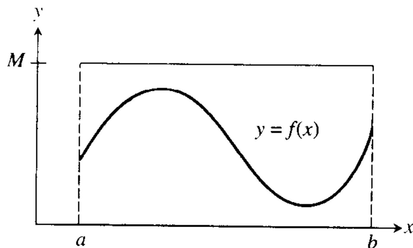
图 7.9 把矩形想象为一个靶.
