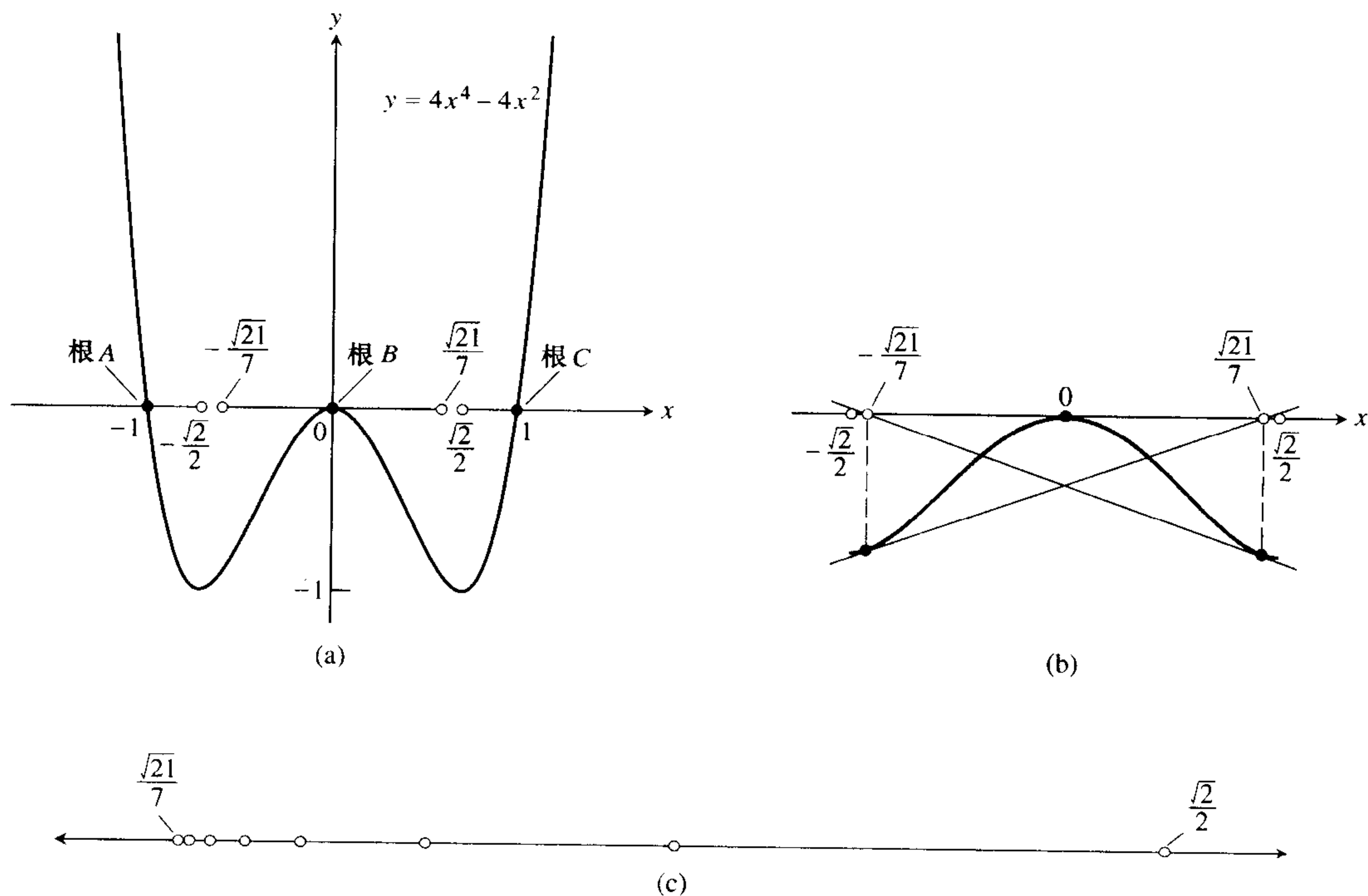
图 3.70 (a) 在 (-\infty, -\sqrt{2}/2) , (-\sqrt{21}/7, \sqrt{21}/7) 和 (\sqrt{2}/2, \infty) 中的起始值分别导至根 A, B 和 C . (b) 值 x = \pm\sqrt{21}/7 互相导至. (c) 在 \sqrt{21}/7 和 \sqrt{2}/2 之间有无穷多个吸引到 A 的点组成的开区间交替着吸引到 C 的点组成的开区间. 这种性态被反射到区间 (-\sqrt{2}/2, -\sqrt{21}/7) .
