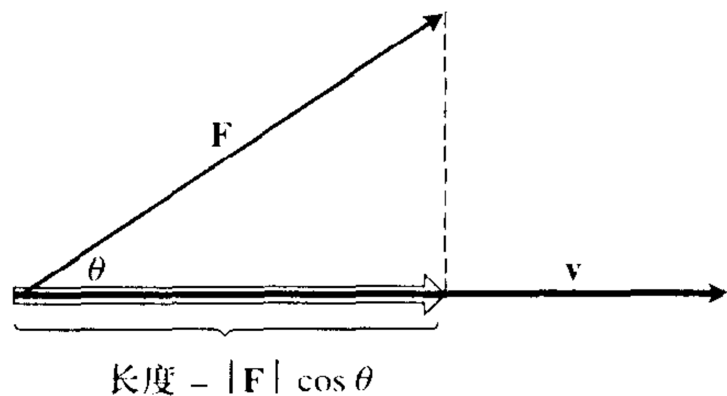
图 9.14 力 \mathbf{F} 在向量 \mathbf{v} 的方向的大小是 \mathbf{F} 在 \mathbf{v} 上的投影的长度 |\mathbf{F}| \cos \theta
