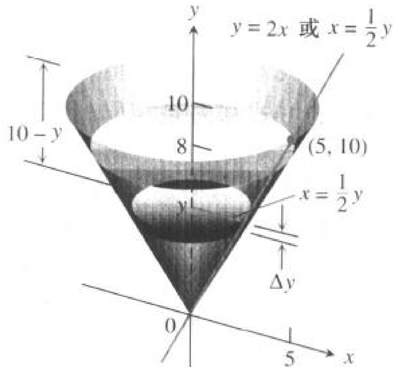
图 5.35 例 7 中的橄榄油
