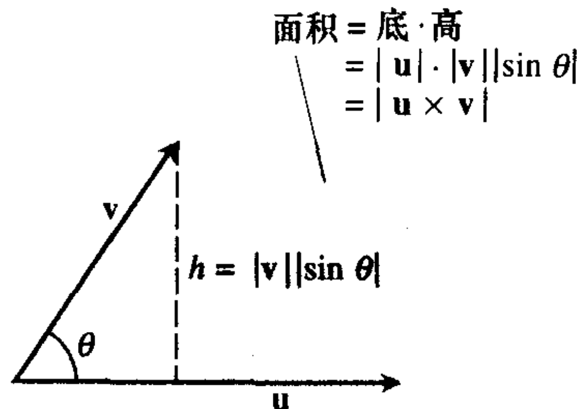
图 10.15 \mathbf{u} 和 \mathbf{v} 确定的平行四边形
