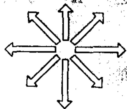
图 13.25 在流体穿过一平面区域的流动中,在“源”处散度为正值,流体进系统,在“漏”处散度为负值,流体离开系统.
