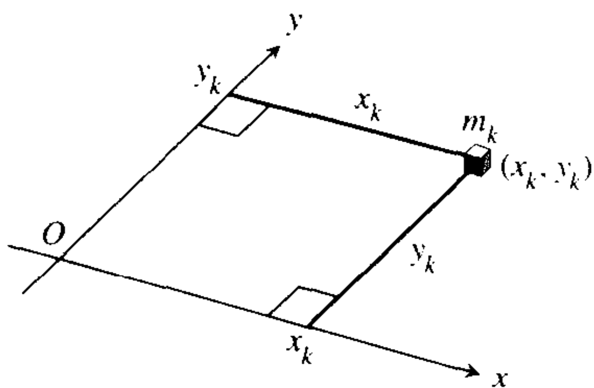
图 12.17 每一质量 m_k 关于每个轴有一个力矩
