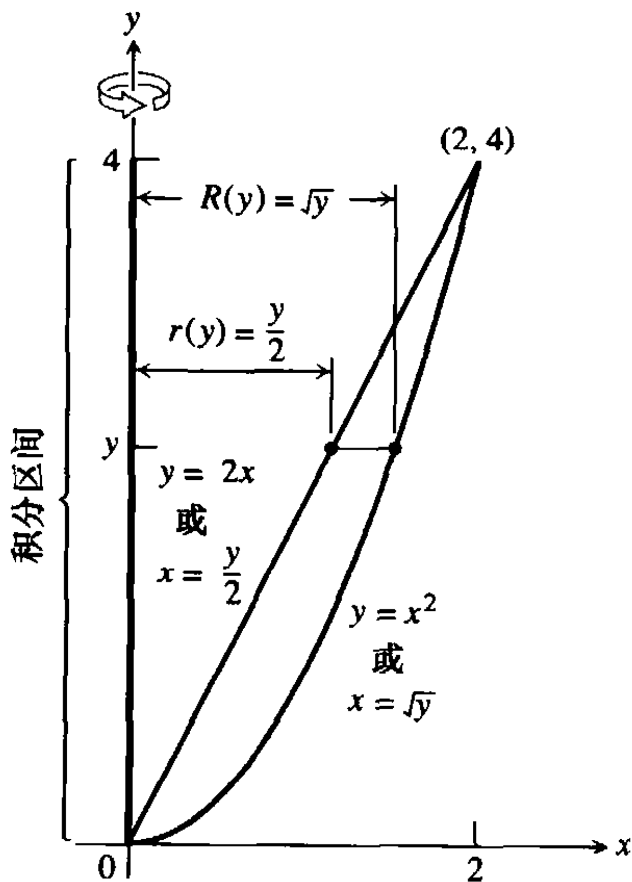
图 5.13 在例 9 中的区域、积分限和半径.
