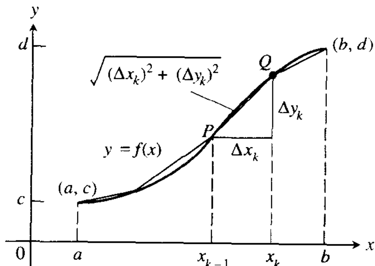
图 5.27 用直线段逼近 f 的图象.
