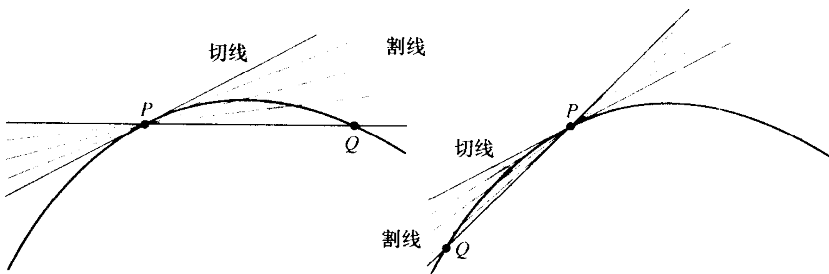
图 1.60 动态地趋向切点.曲线在点 P 的切线是过 P 的直线其斜率是当曲线上的点 Q 沿曲线从点 P 的两侧趋于点 P 时割线 PQ 的斜率的极限.
