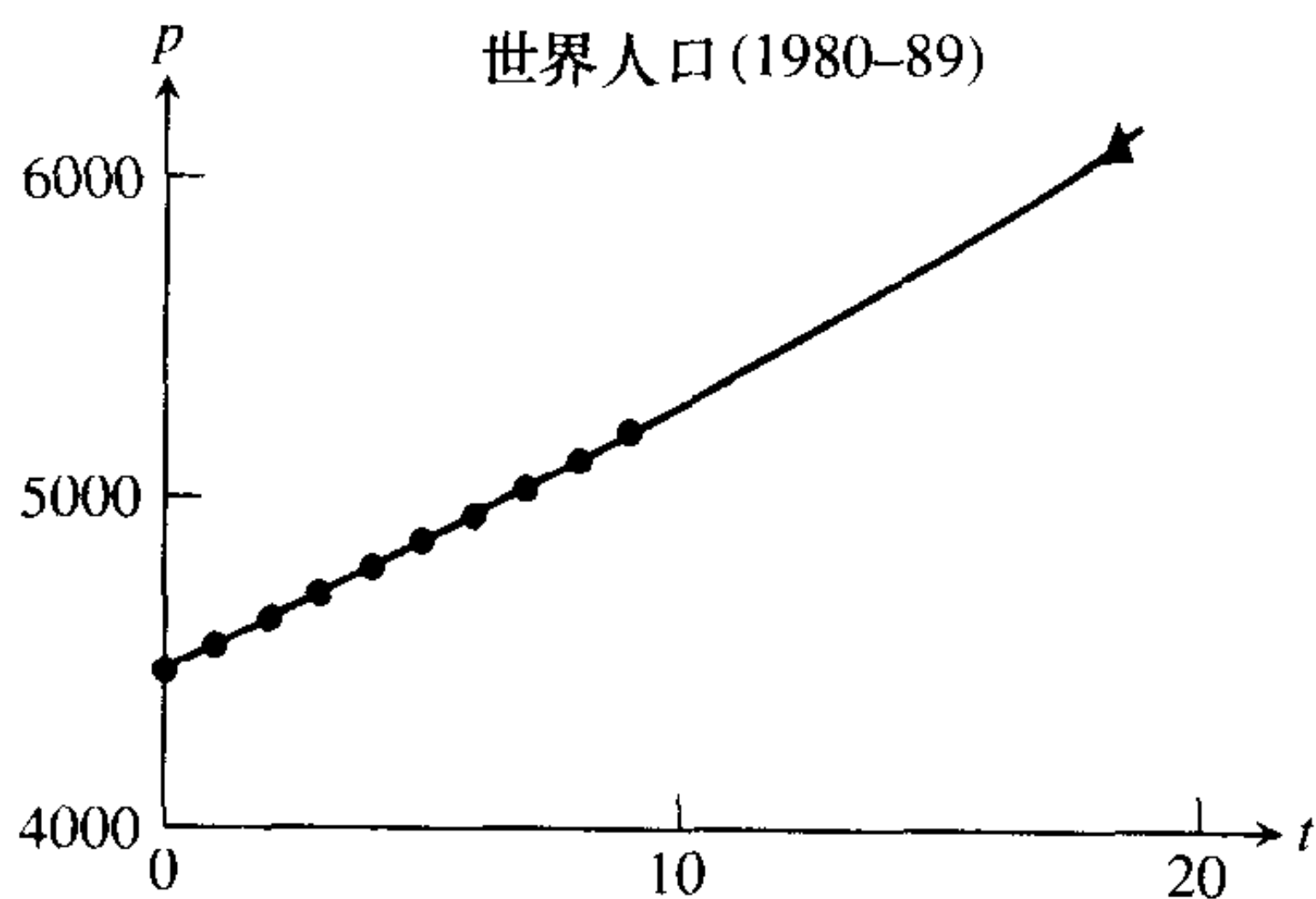
图 6.21 注意解 P = 4454e^{0.017t} 给的 t = 19 的值是 6152.16. (例 5)
