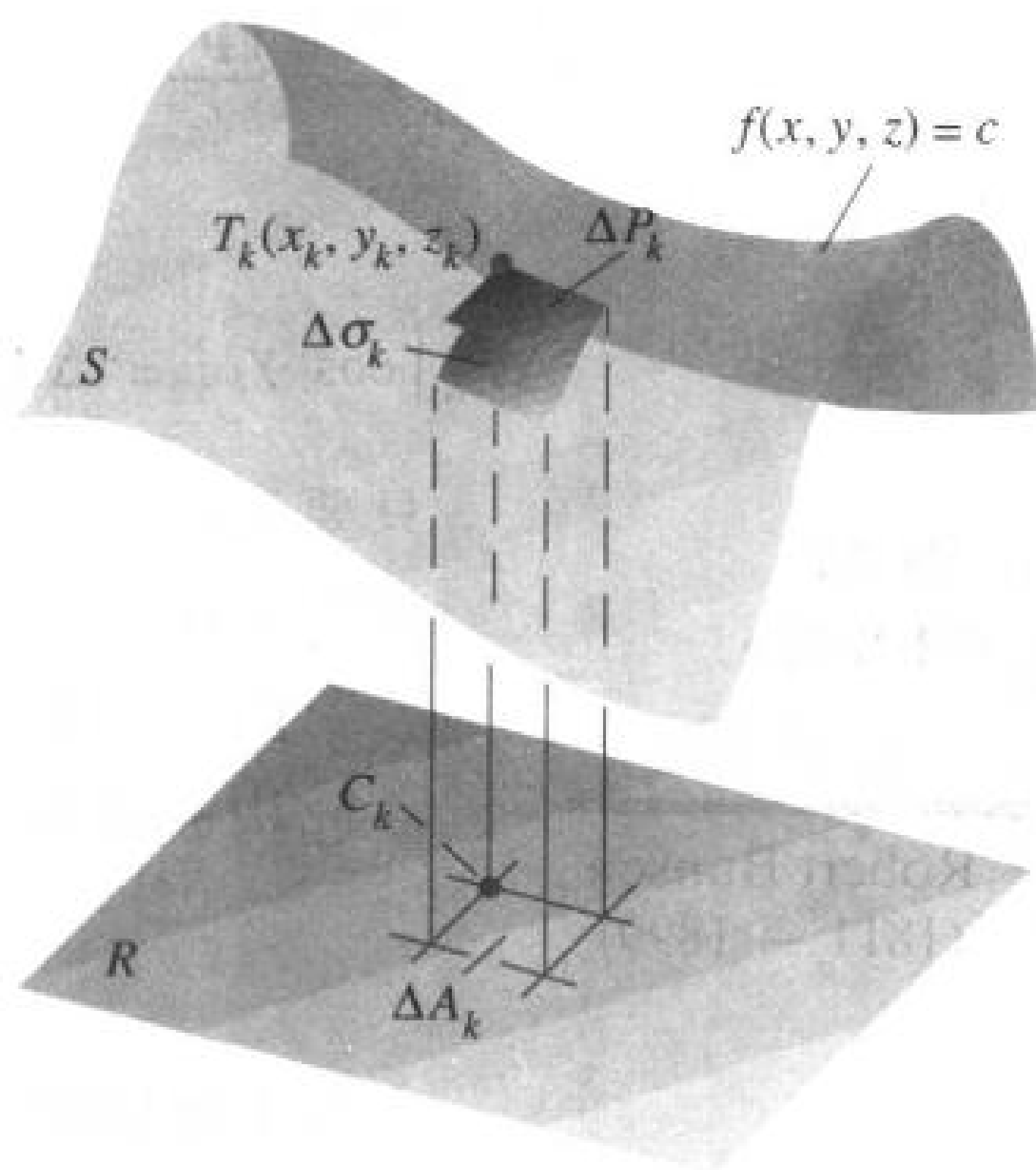
图 13.39 曲面 S 及其在它之下的平面上的垂直投影,你可以把 R 想像成 S 在平面上的影子.小切平面 \Delta P_k 是对 \Delta A_k 之上的小曲面片 \Delta \sigma_k 的近似.
