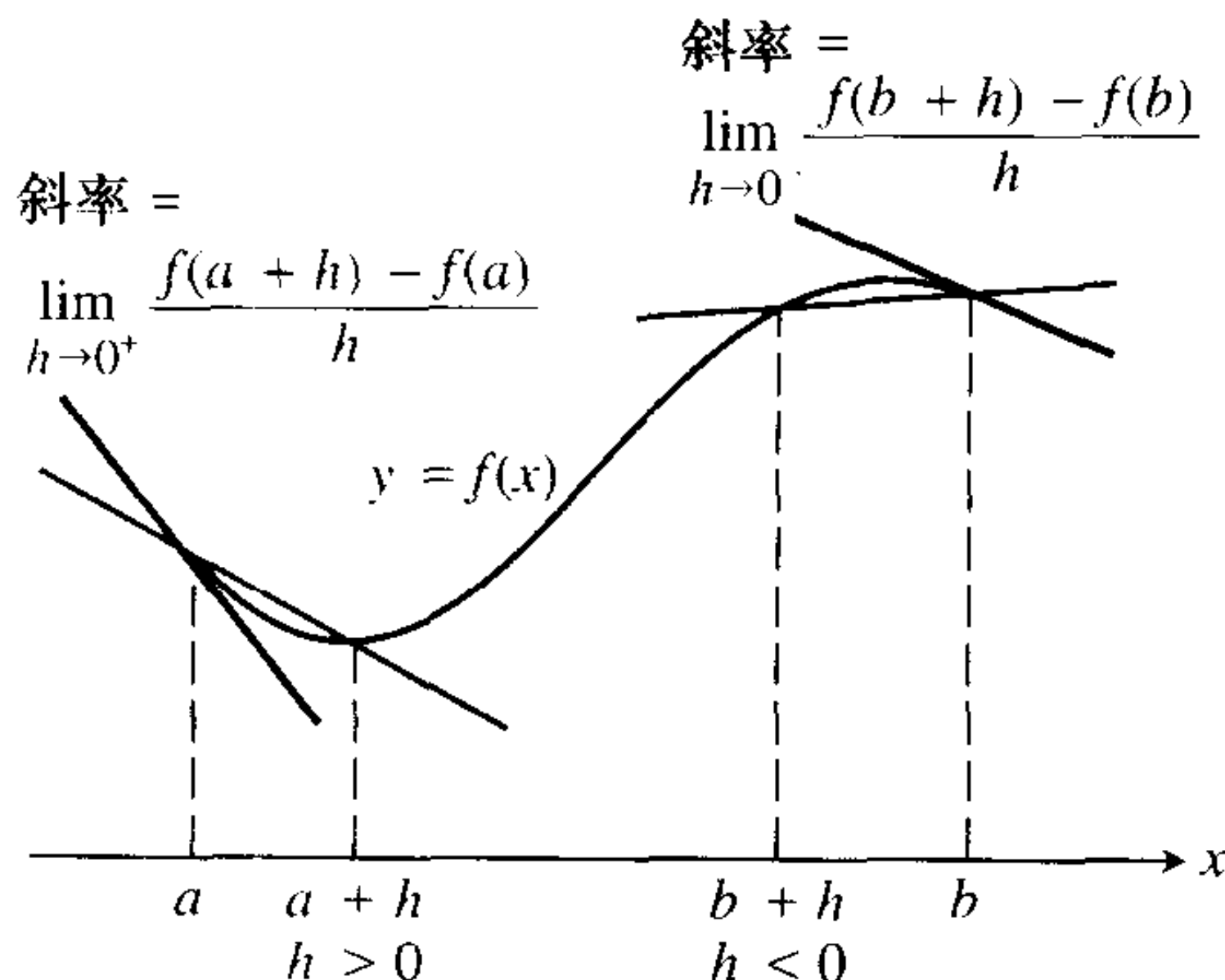
图 2.7 端点的导数是单侧极限.
