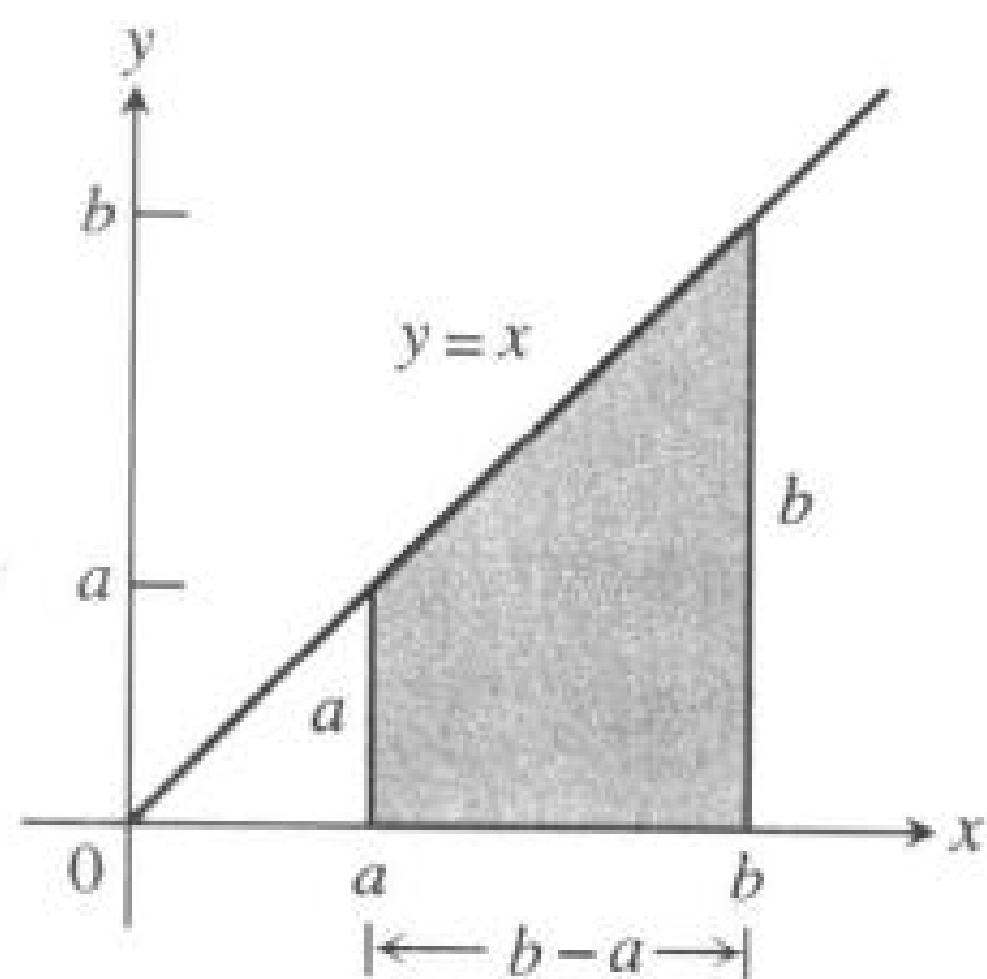
图 4.10 例 3 中的区域.
