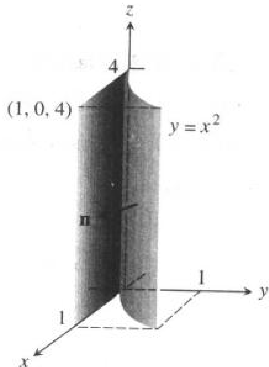
图 13.57 例 7 的抛物面.
