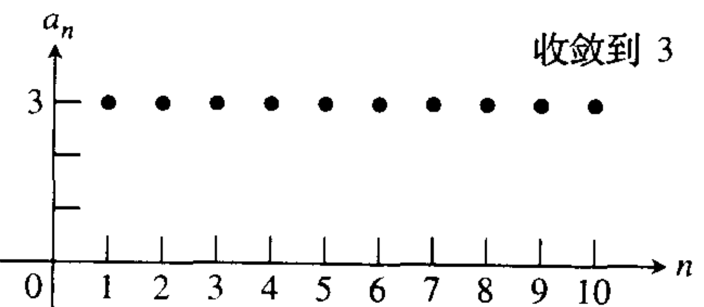
图 8.1 对例 1 中的序列以两种方式作图. 把 a_n 画在数轴上和把 (n, a_n) 画在坐标平面上.
